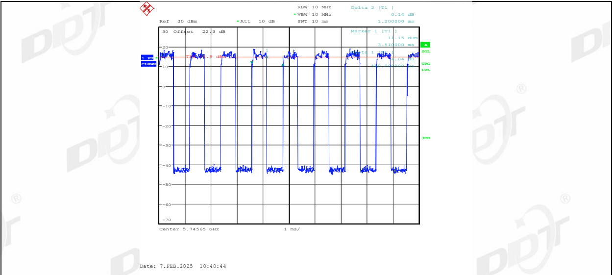
11AX20MIMO_Ant2_5745_26Tone_RU8
