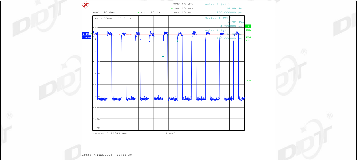
11AX20MIMO_Ant1_5745_52Tone_RU39
