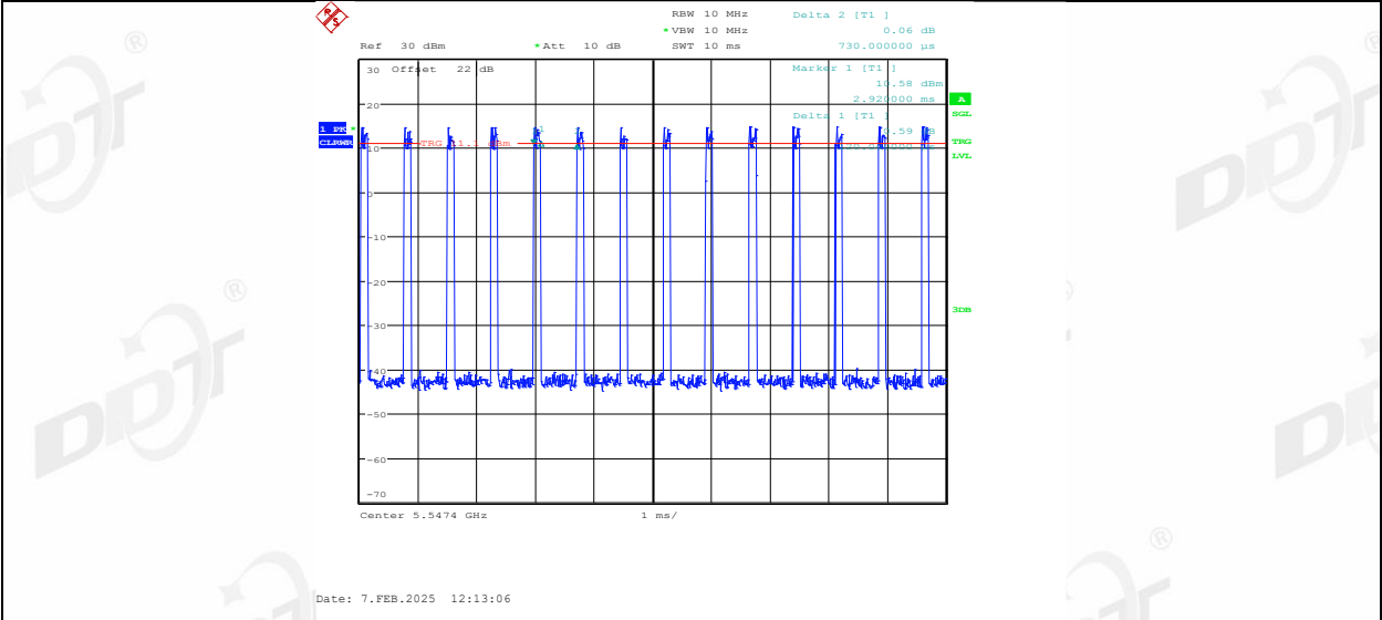
11AX40MIMO_Ant2_5550_242Tone_RU62
