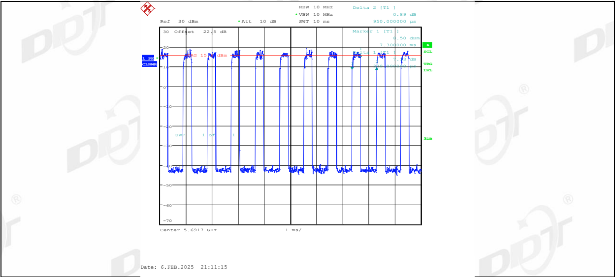
11AX20MIMO_Ant2_5700_52Tone_RU39
