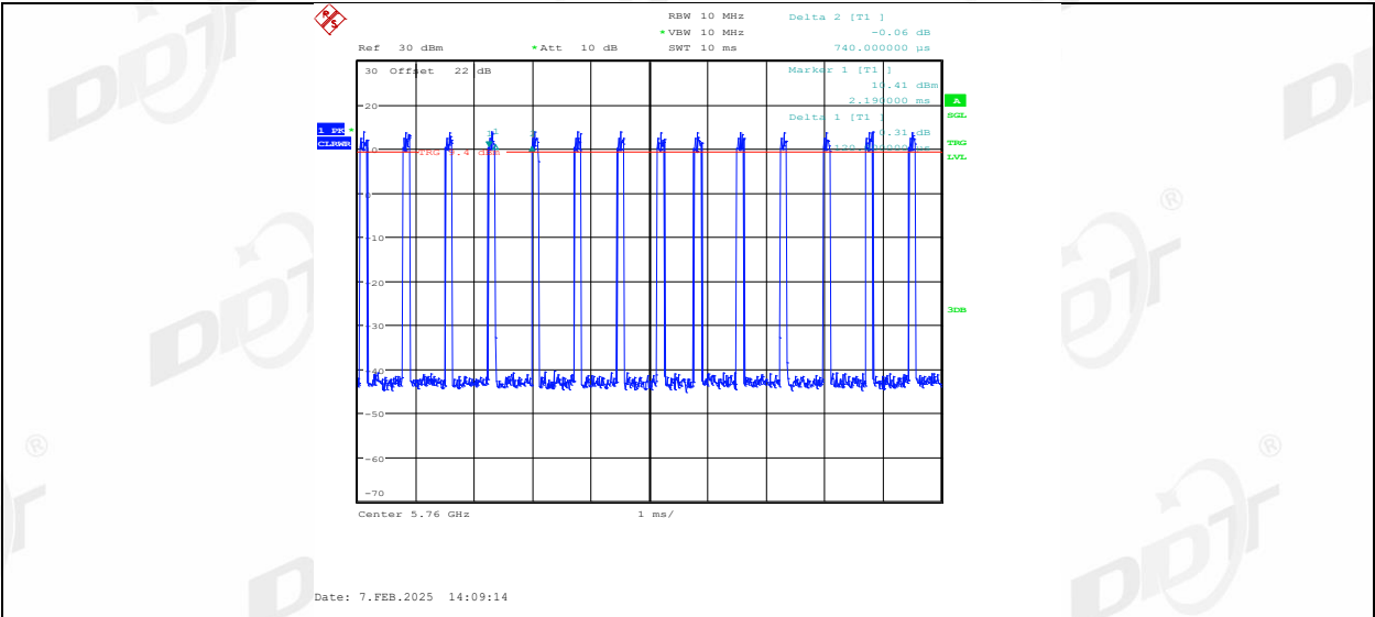
11AX40MIMO_Ant2_5755_242Tone_RU61
