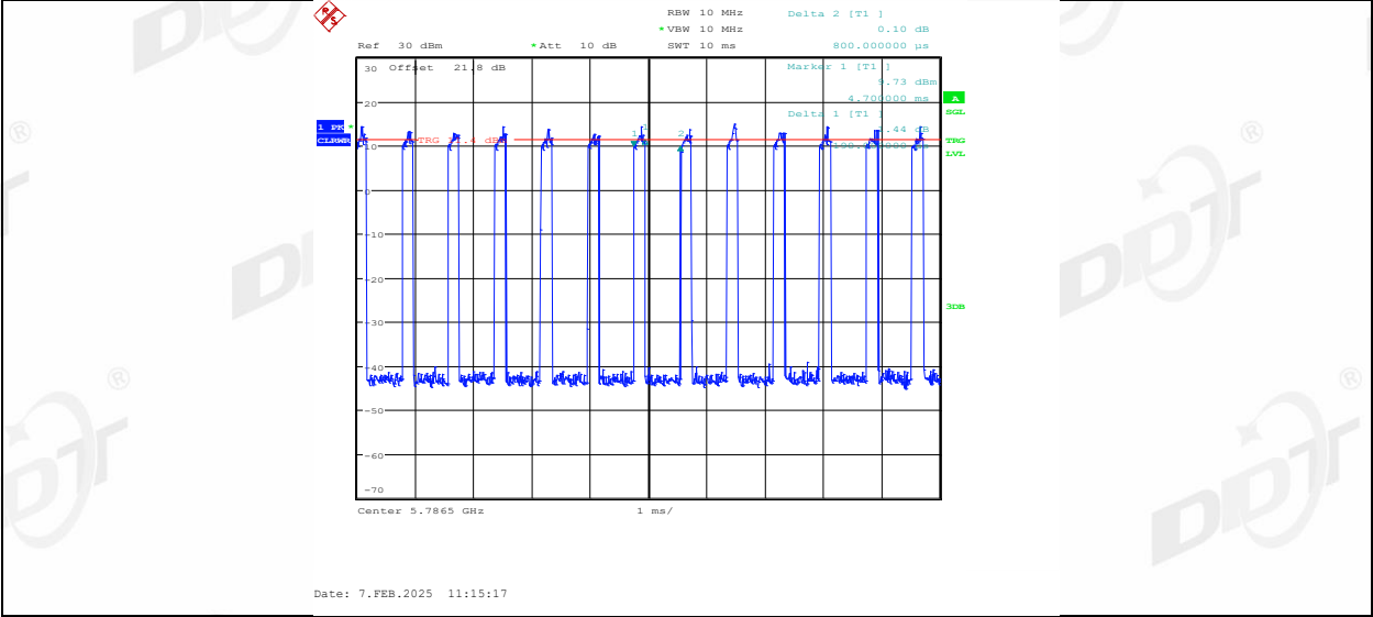
11AX20MIMO_Ant2_5785_26Tone_RU0
