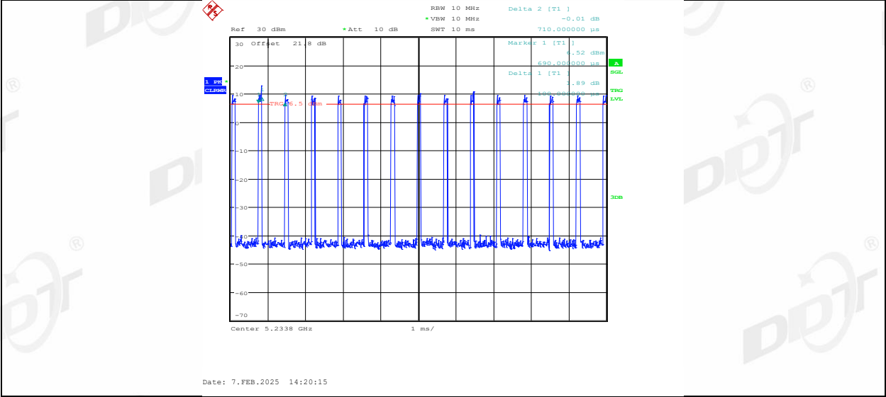
11AX80MIMO_Ant2_5210_484Tone_RU65
