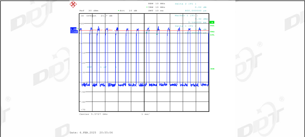
11AX20MIMO_Ant1_5580_106Tone_RU54
