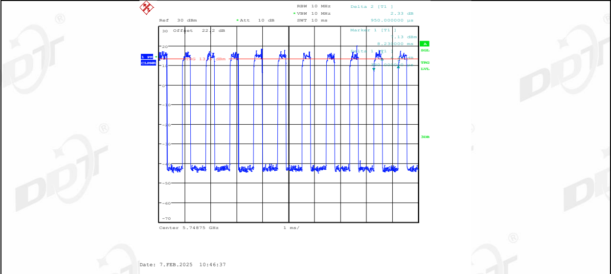
11AX20MIMO_Ant1_5745_52Tone_RU40
