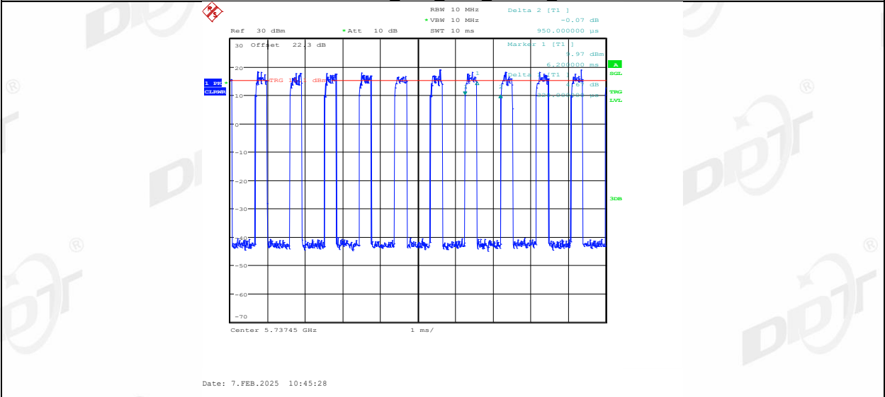
11AX20MIMO_Ant2_5745_52Tone_RU39
