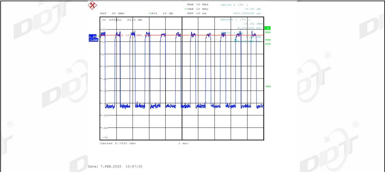
11AX20MIMO_Ant2_5745_52Tone_RU40
