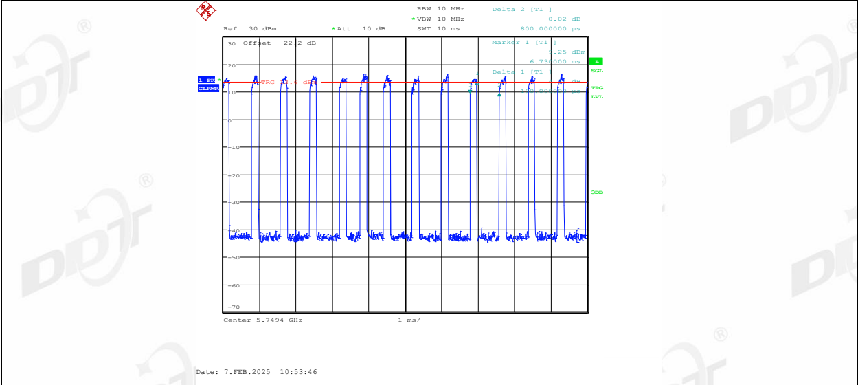
11AX20MIMO_Ant2_5745_26Tone_RU0
