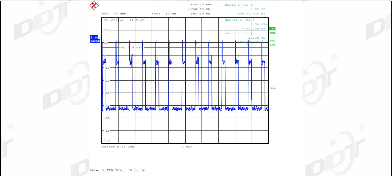
11AX20MIMO_Ant1_5745_106Tone_RU54
