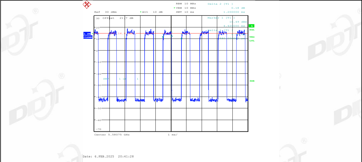
11AX20MIMO_Ant1_5580_26Tone_RU8
