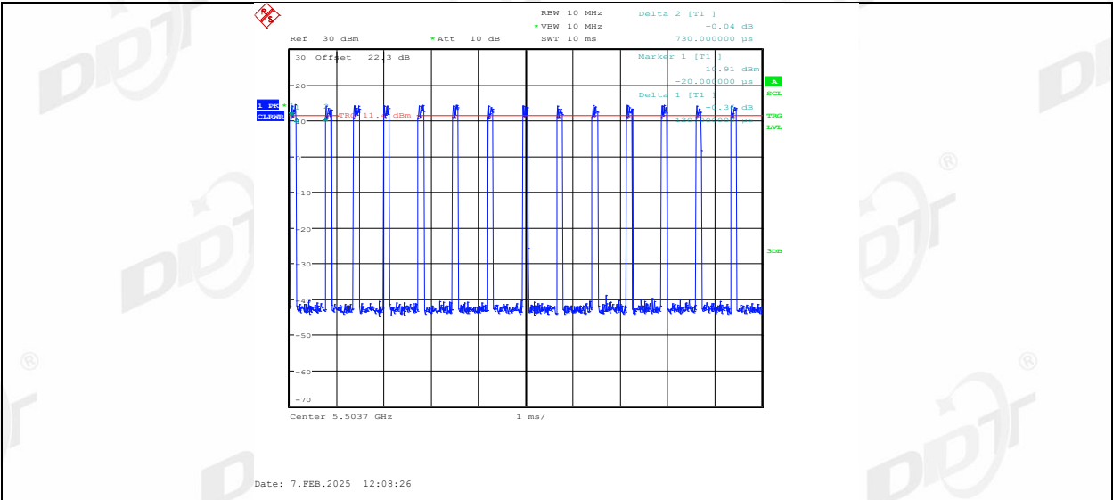
11AX40MIMO_Ant2_5510_242Tone_RU62
