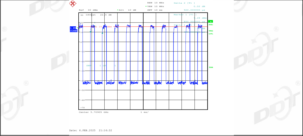
11AX20MIMO_Ant2_5700_106Tone_RU53
