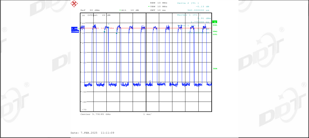
11AX20MIMO_Ant2_5785_106Tone_RU53
