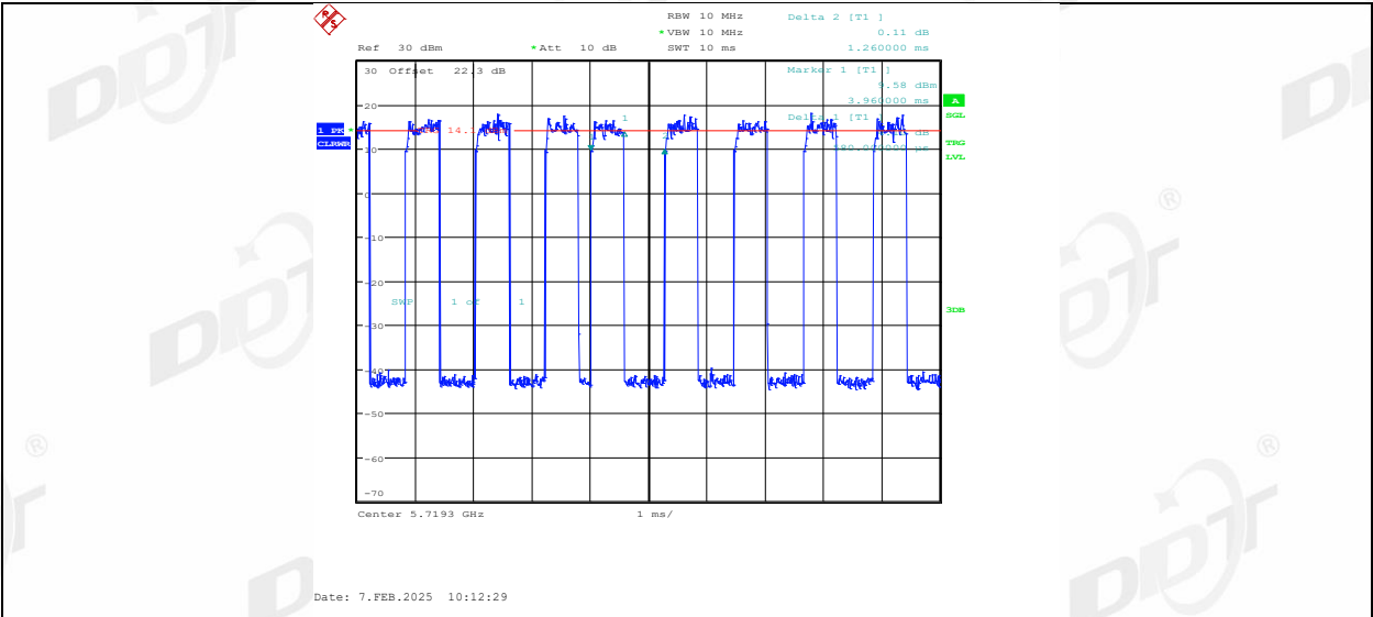
11AX20MIMO_Ant1_5720_26Tone_RU8
