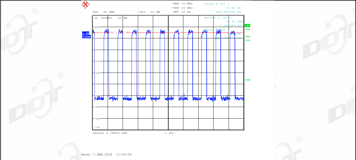
11AX20MIMO_Ant2_5785_52Tone_RU40
