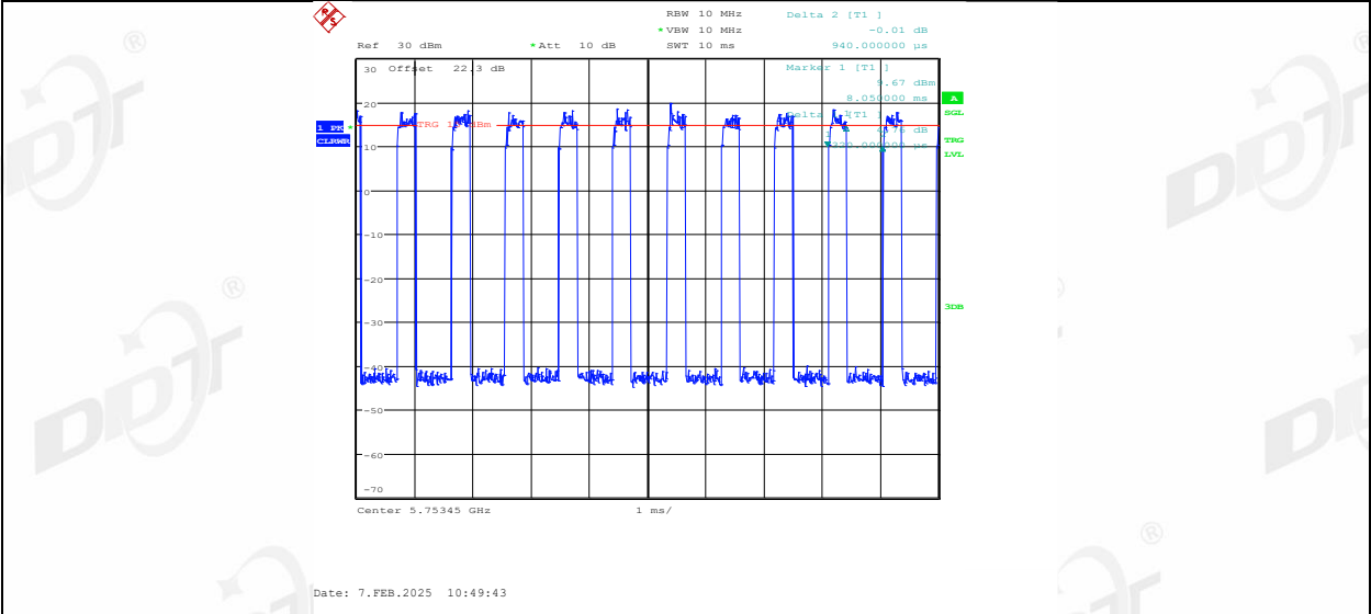
11AX20MIMO_Ant2_5745_106Tone_RU53
