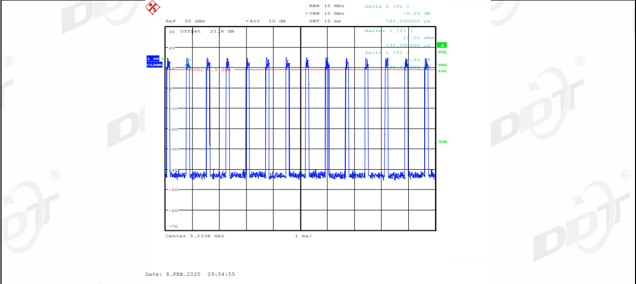
11AX40MIMO_Ant2_5230_242Tone_RU61
