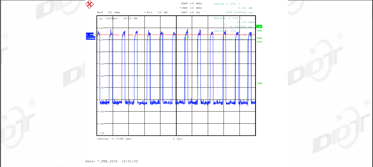
11AX20MIMO_Ant2_5745_106Tone_RU54
