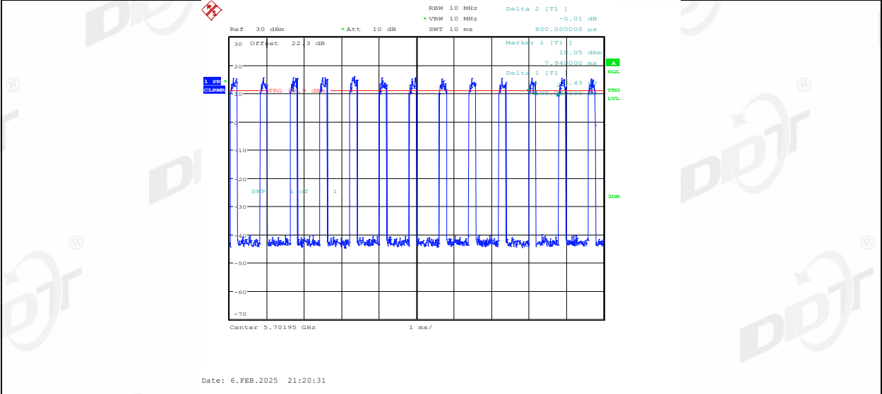
11AX20MIMO_Ant2_5700_26Tone_RU0
