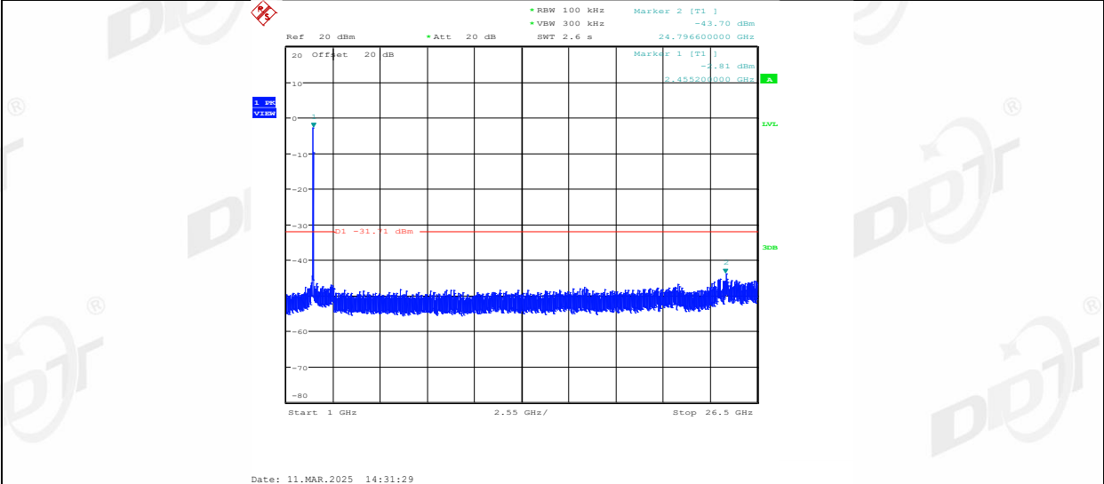
11AX40MIMO_Ant2_2452_0~Reference
