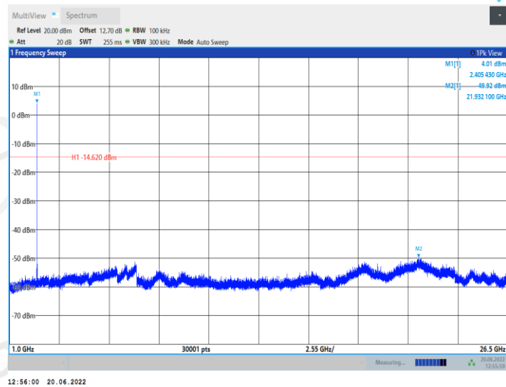
GFSK_Ant1_2442_0~Reference
