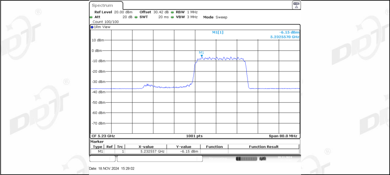
11AX40MIMO_Ant2_5230_242Tone_RU61
