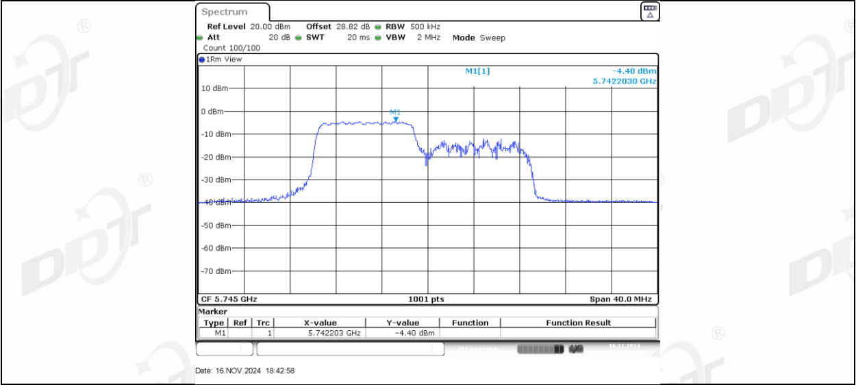
11AX20MIMO_Ant2_5745_106Tone_RU54
