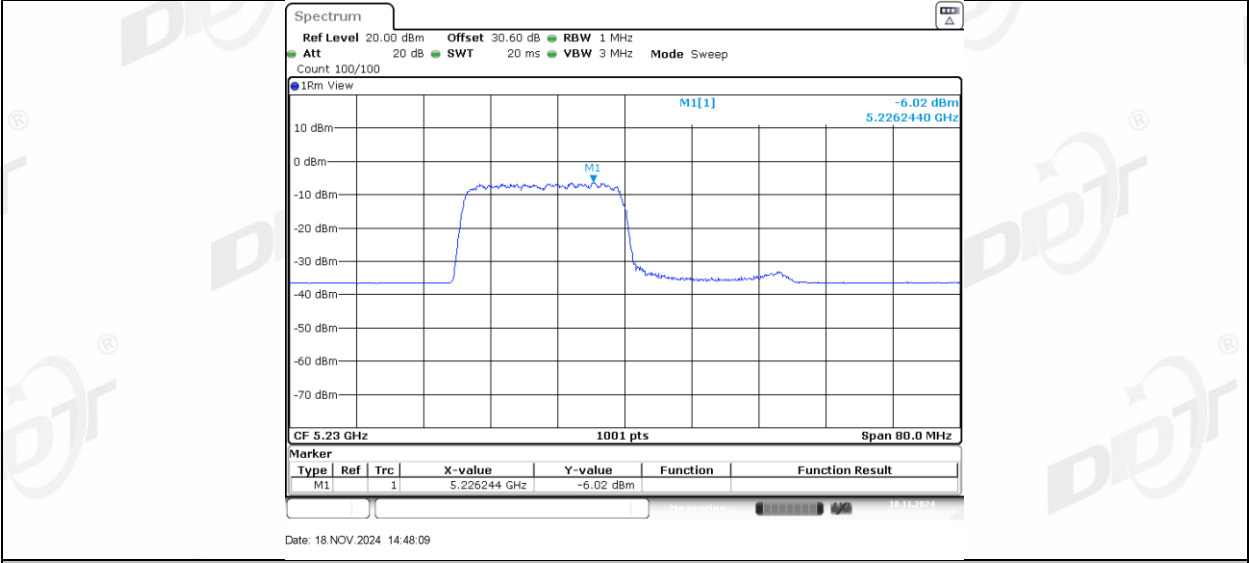
11AX40MIMO_Ant2_5230_242Tone_RU62
