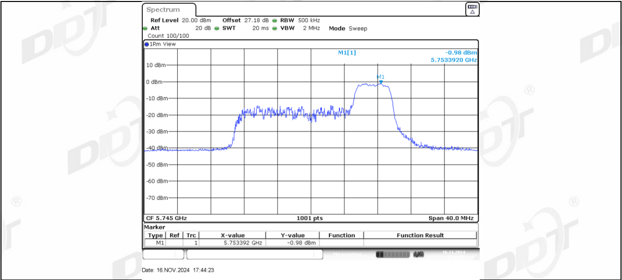
11AX20MIMO_Ant2_5745_106Tone_RU53
