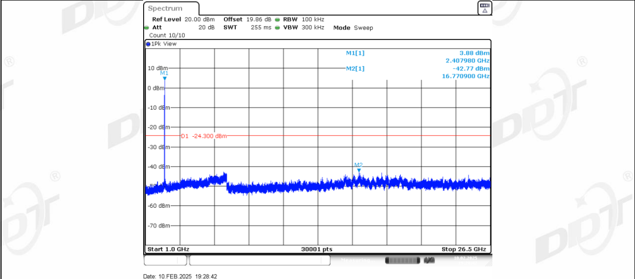
11N20MIMO_Ant2_2412_0~Reference
