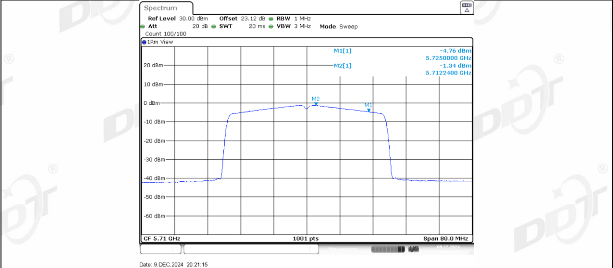
11AX40MIMO_Ant1_5710_UNII-3
