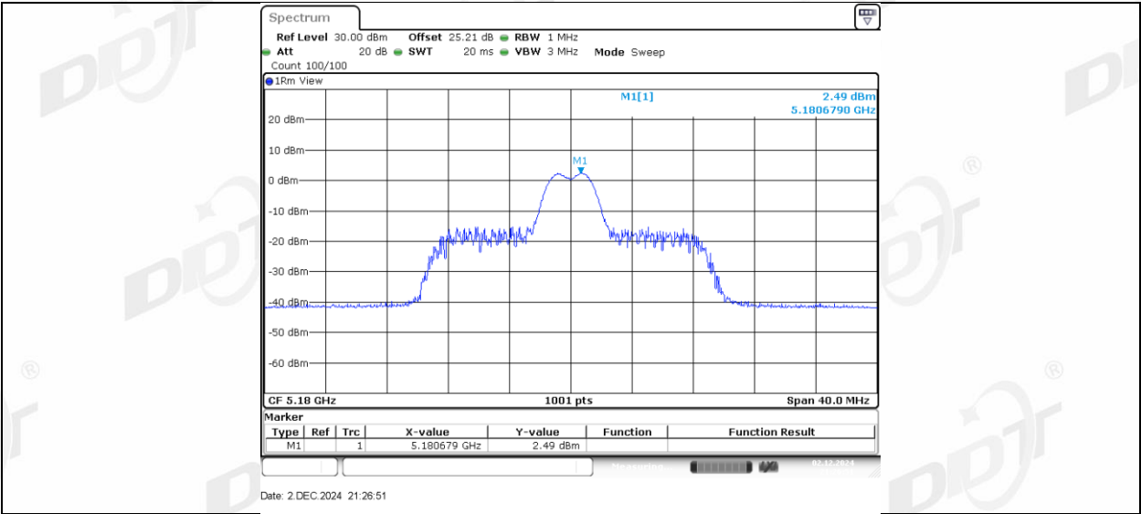
11AX20MIMO_Ant1_5180_26Tone_RU8
