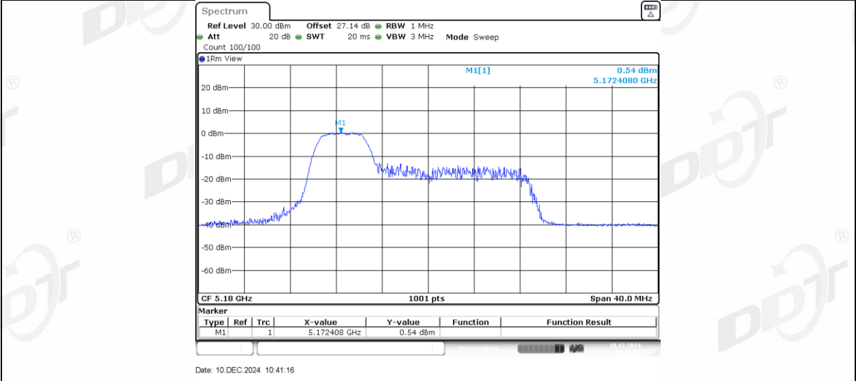
11AX20MIMO_Ant1_5180_52Tone_RU39
