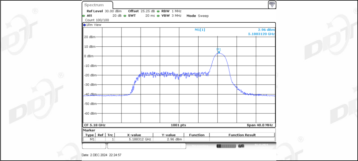
11AX20MIMO_Ant1_5180_52Tone_RU37
