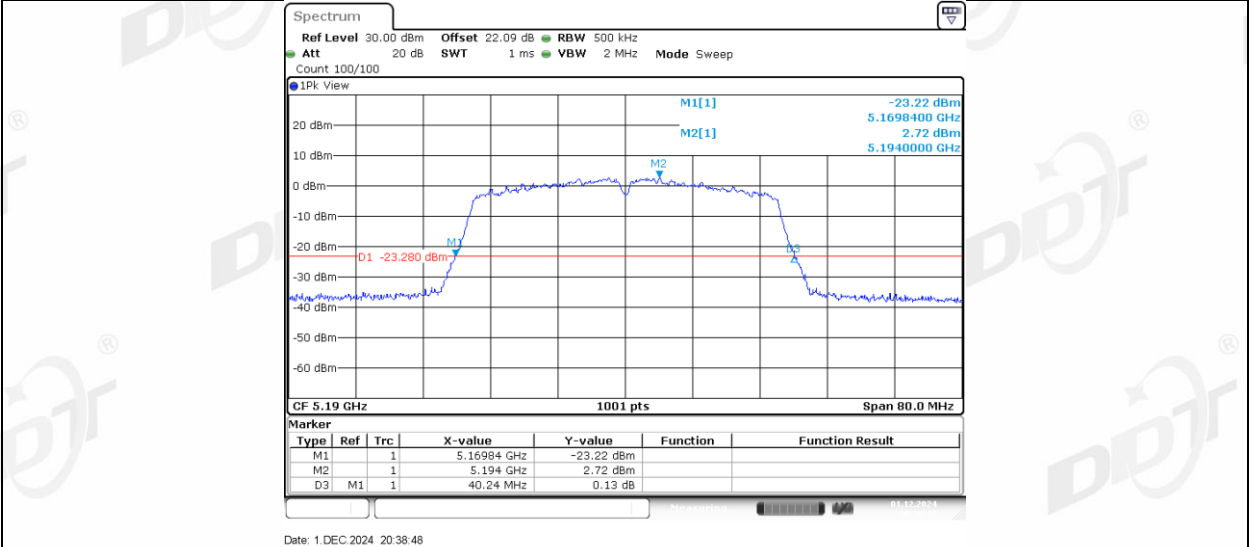
11AC40MIMO_Ant2_5190
