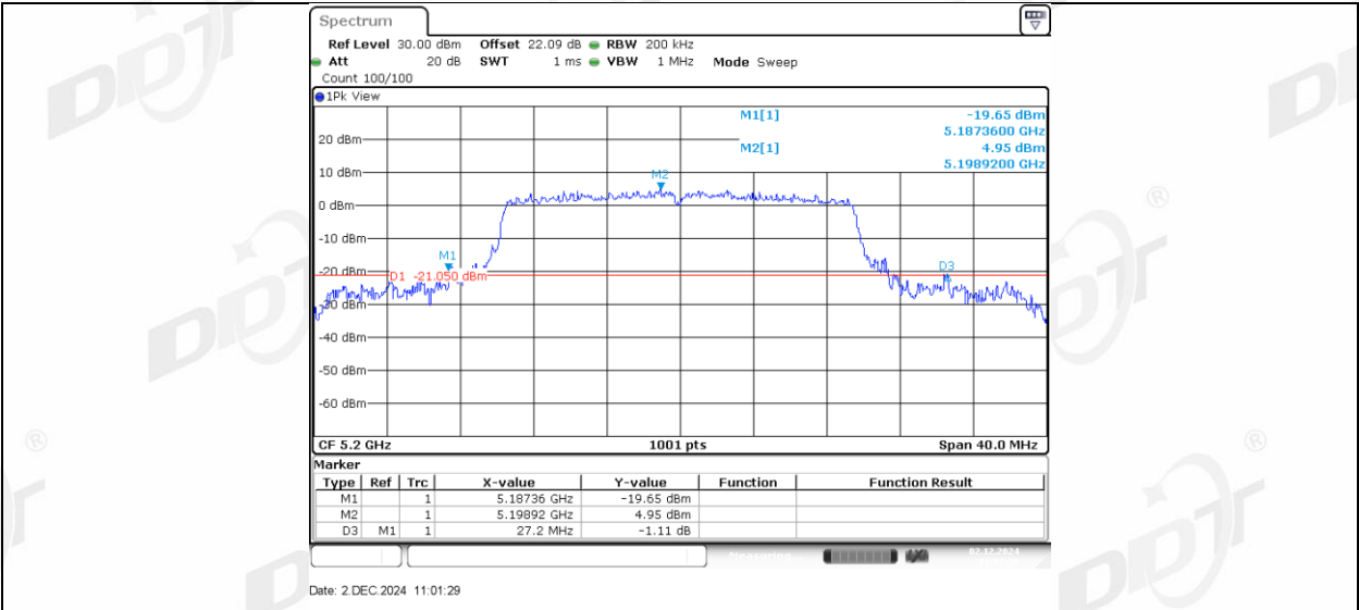
11AX20MIMO_Ant2_5200
