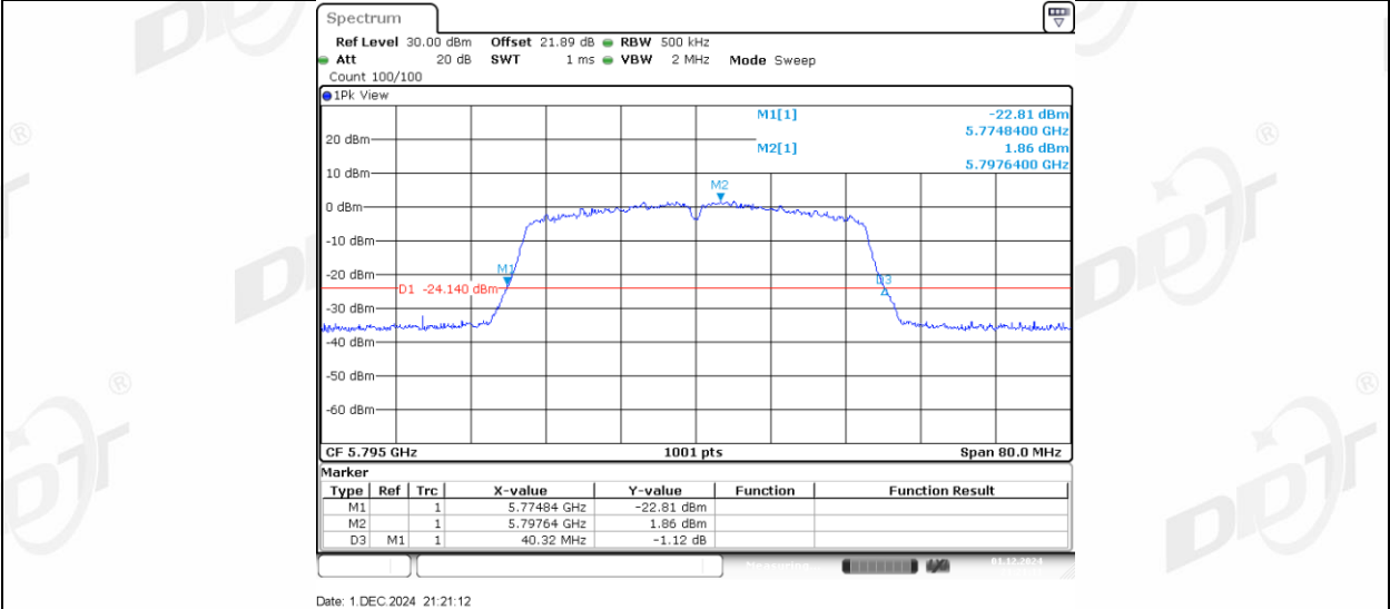
11AC40MIMO_Ant2_5795
