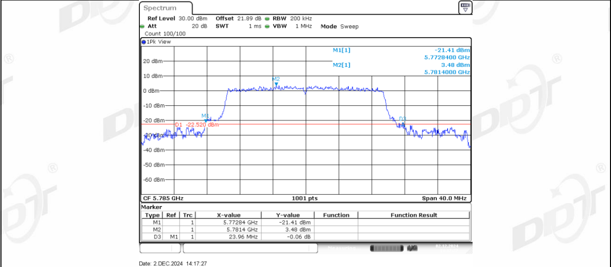
11AX20MIMO_Ant2_5785
