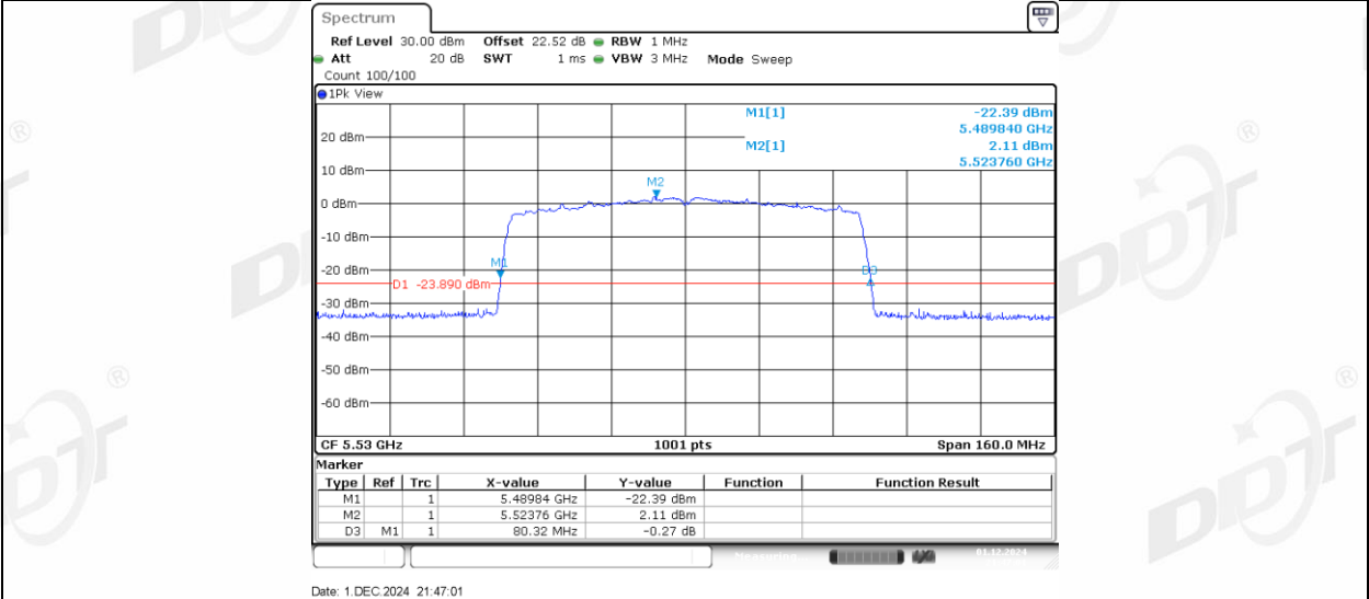
11AC80MIMO_Ant2_5530
