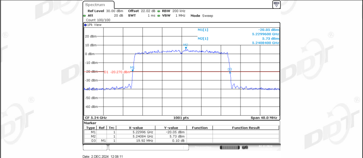
11AX20MIMO_Ant2_5240
