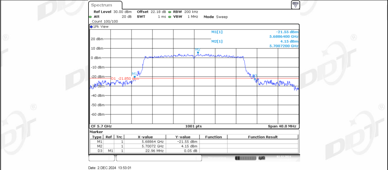
11AX20MIMO_Ant2_5700
