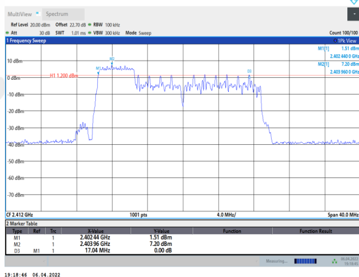
11AX20MIMO_Ant1_2412_52Tone_RU38
