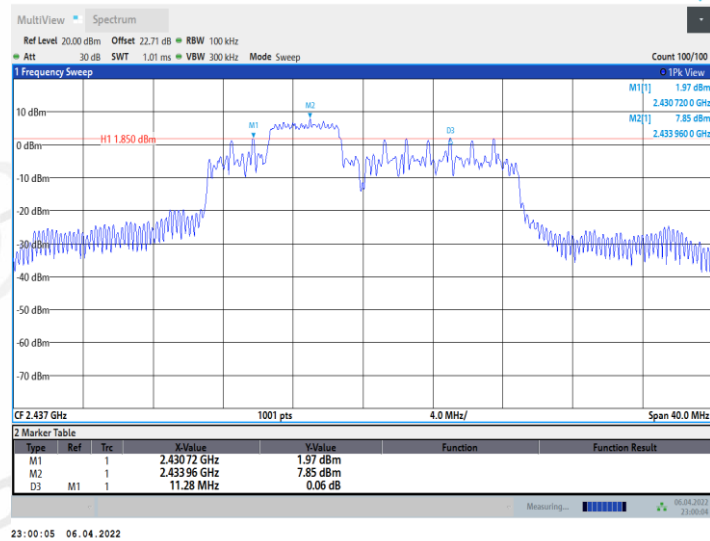
11AX20MIMO_Ant1_2437_52Tone_RU39
