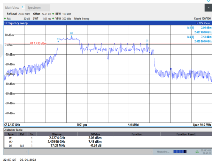
11AX20MIMO_Ant1_2437_52Tone_RU38
