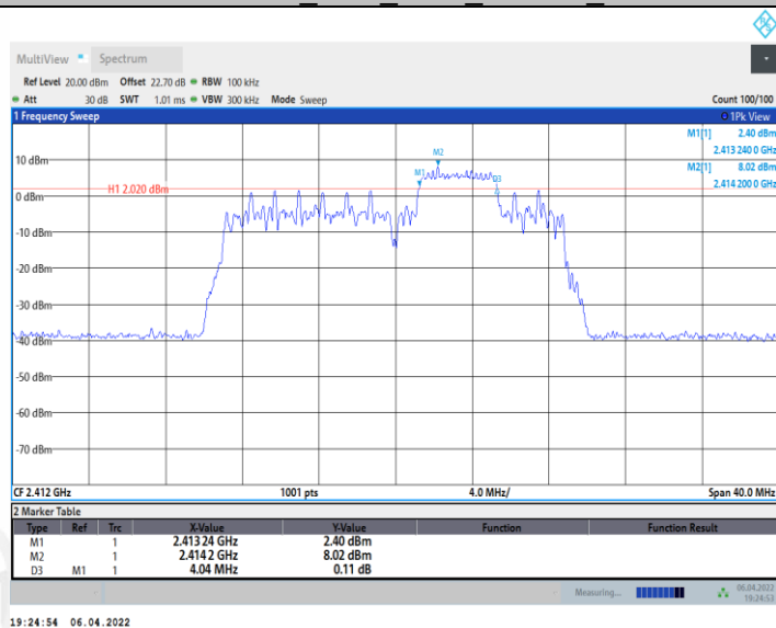
11AX20MIMO_Ant1_2412_52Tone_RU40
