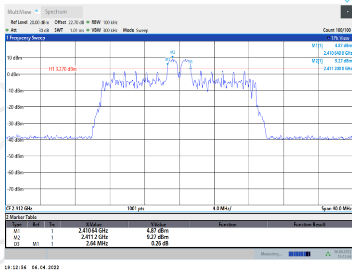
11AX20MIMO_Ant1_2412_26Tone_RU8
