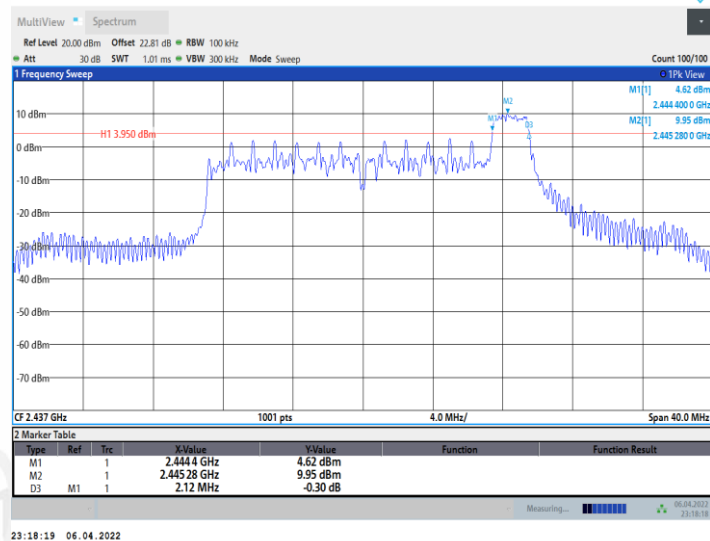
11AX20MIMO_Ant2_2437_52Tone_RU37
