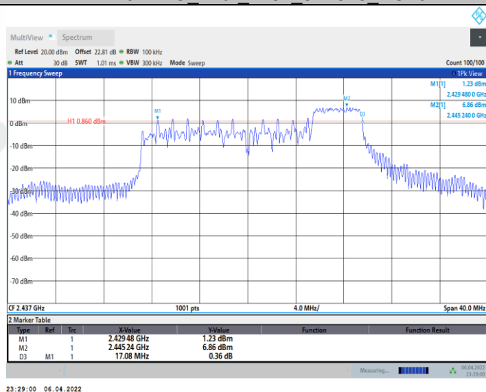
11AX20MIMO_Ant2_2437_106Tone_RU53
