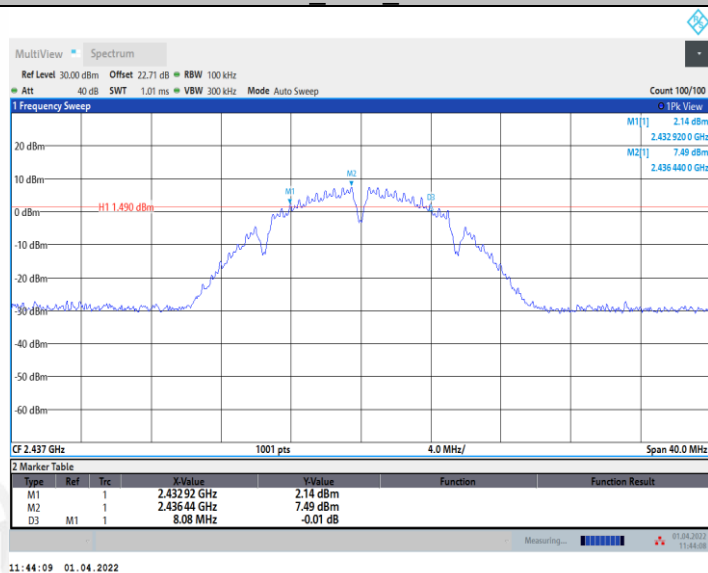
11B_Ant2_2437
