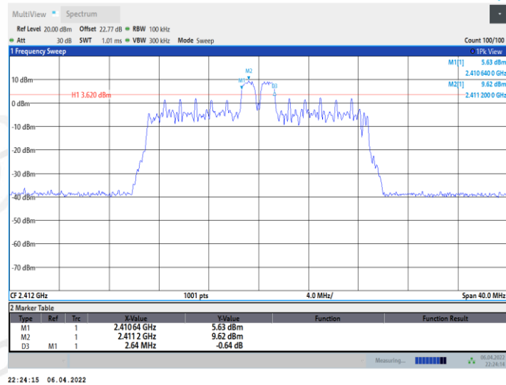
11AX20MIMO_Ant2_2412_26Tone_RU8
