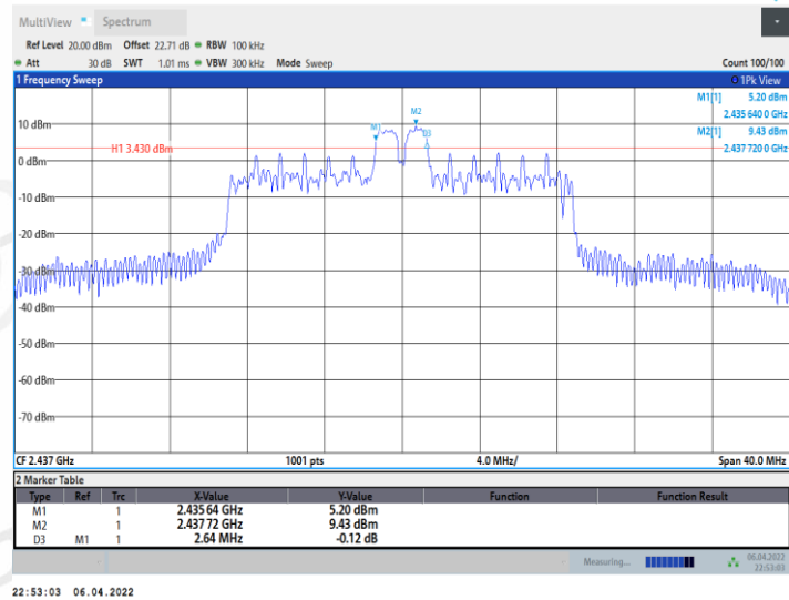
11AX20MIMO_Ant1_2437_26Tone_RU8
