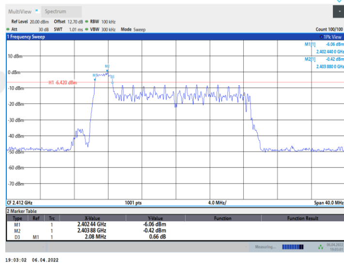
11AX20MIMO_Ant1_2412_26Tone_RU4
