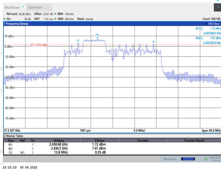
11AX20MIMO_Ant2_2437_52Tone_RU39
