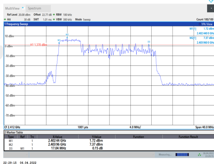
11AX20MIMO_Ant2_2412_52Tone_RU38
