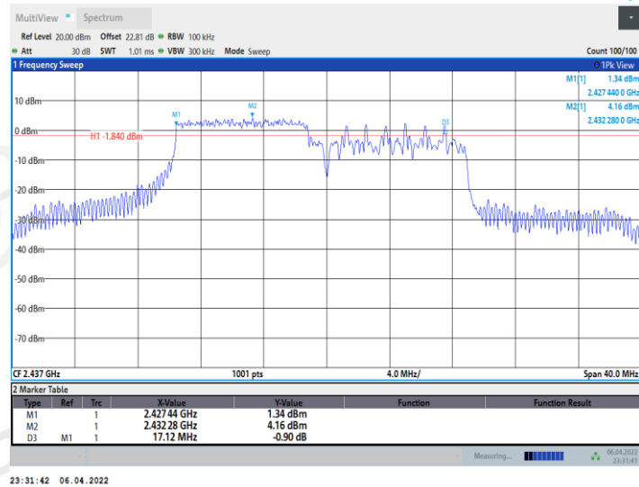
11AX20MIMO_Ant2_2437_106Tone_RU54
