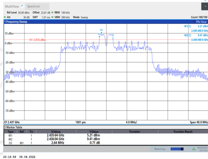
11AX20MIMO_Ant2_2437_26Tone_RU8
