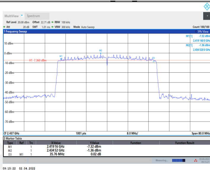
11AX40MIMO_Ant2_2437
