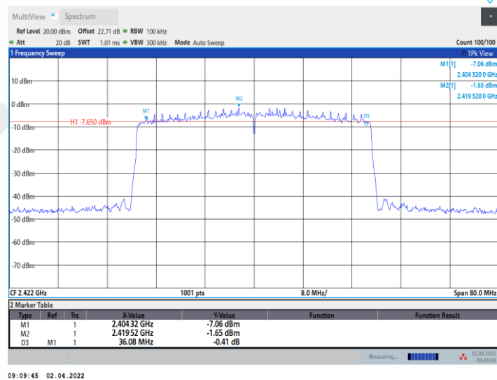
11AX40MIMO_Ant2_2422
