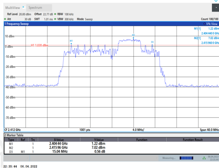
11AX20MIMO_Ant2_2412_52Tone_RU40
