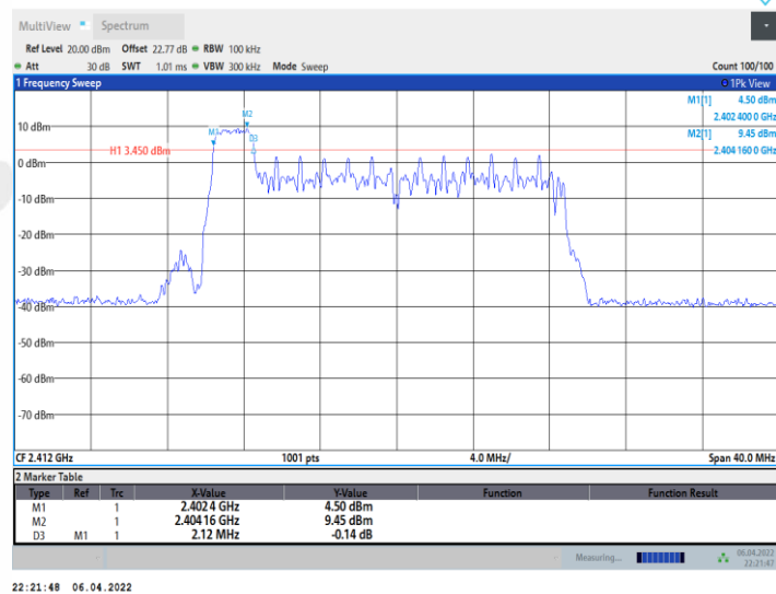
11AX20MIMO_Ant2_2412_26Tone_RU4
