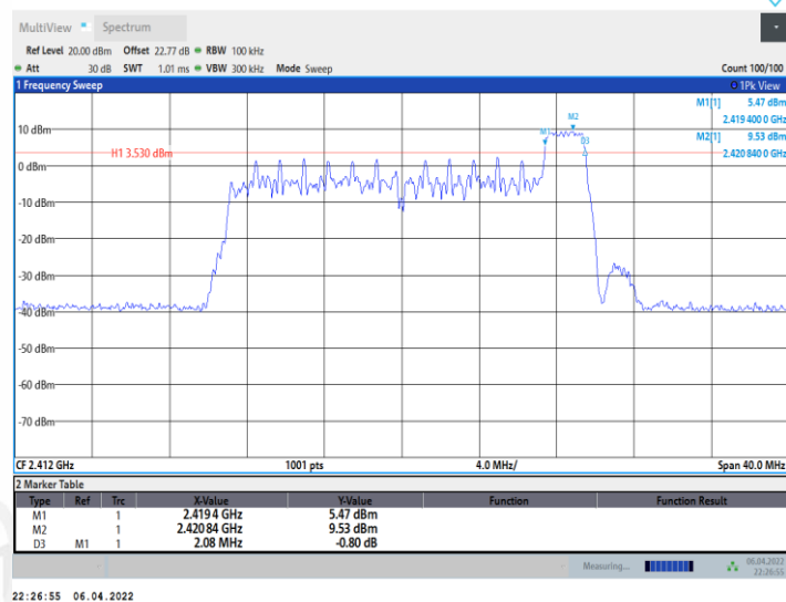
11AX20MIMO_Ant2_2412_52Tone_RU37
