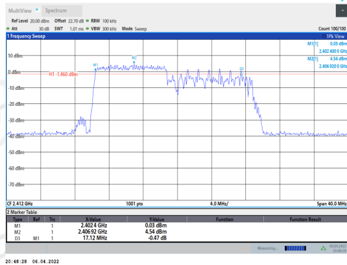
11AX20MIMO_Ant1_2412_106Tone_RU54
