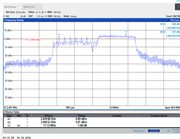
11AX20MIMO_Ant2_2437_26Tone_RU0
