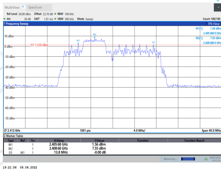
11AX20MIMO_Ant1_2412_52Tone_RU39
