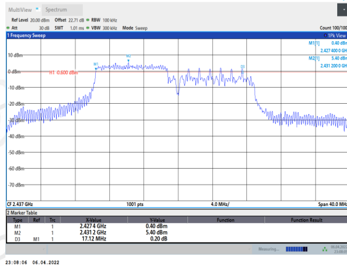
11AX20MIMO_Ant1_2437_106Tone_RU54
