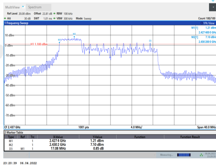
11AX20MIMO_Ant2_2437_52Tone_RU38
