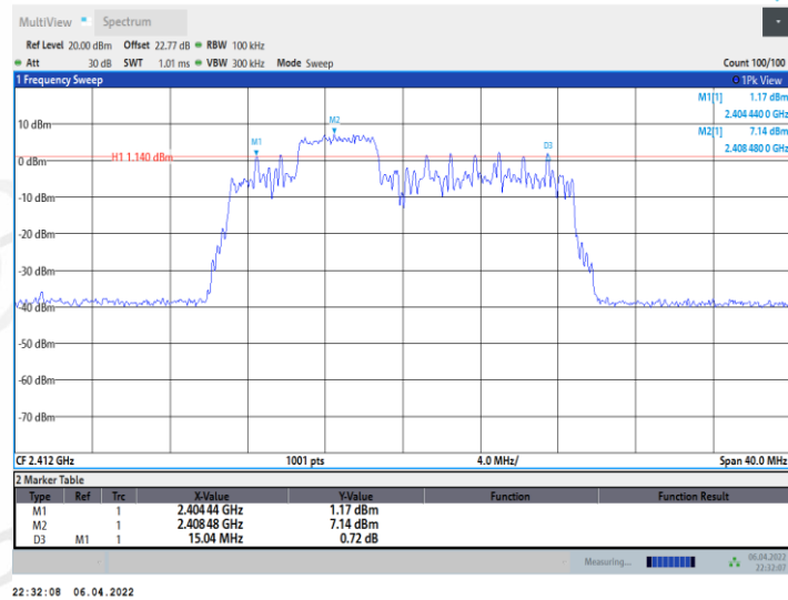
11AX20MIMO_Ant2_2412_52Tone_RU39
