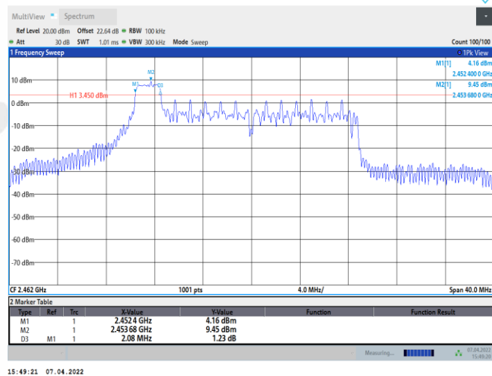
11AX20MIMO_Ant1_2462_26Tone_RU4
