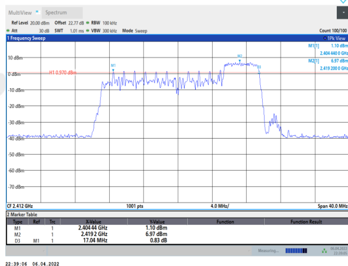
11AX20MIMO_Ant2_2412_106Tone_RU53
