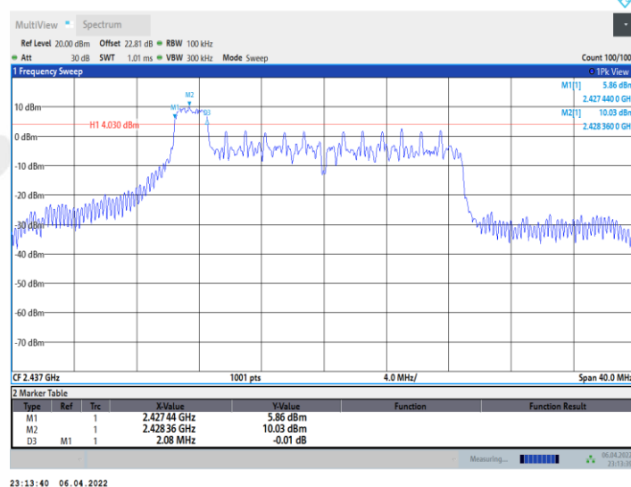
11AX20MIMO_Ant2_2437_26Tone_RU4
