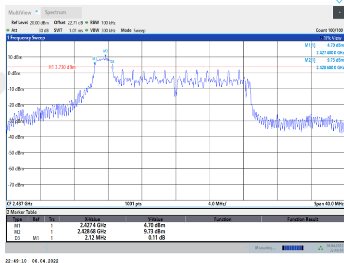
11AX20MIMO_Ant1_2437_26Tone_RU4
