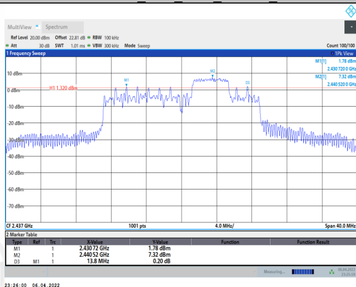
11AX20MIMO_Ant2_2437_52Tone_RU40
