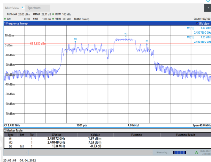
11AX20MIMO_Ant1_2437_52Tone_RU40
