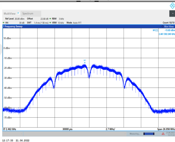
11B_Ant2_2462
