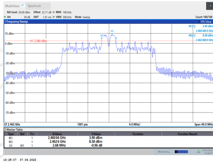
11AX20MIMO_Ant2_2462_26Tone_RU8
