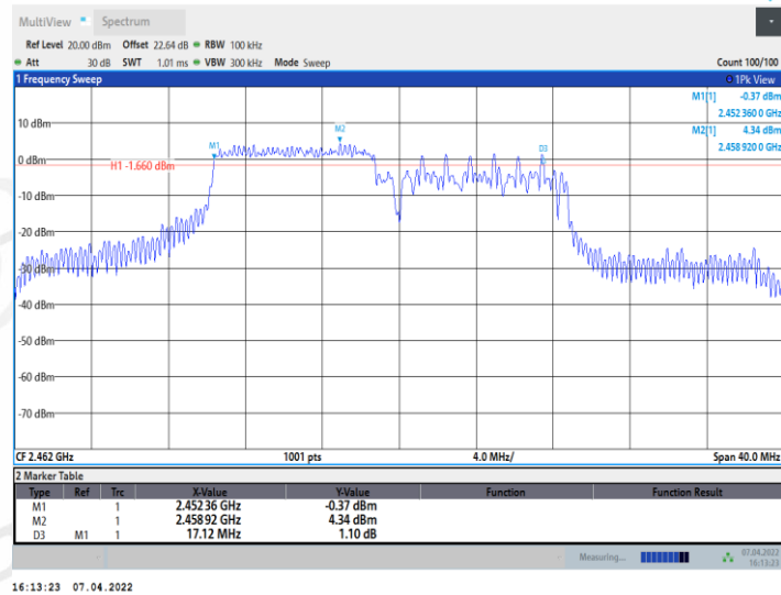
11AX20MIMO_Ant1_2462_106Tone_RU54
