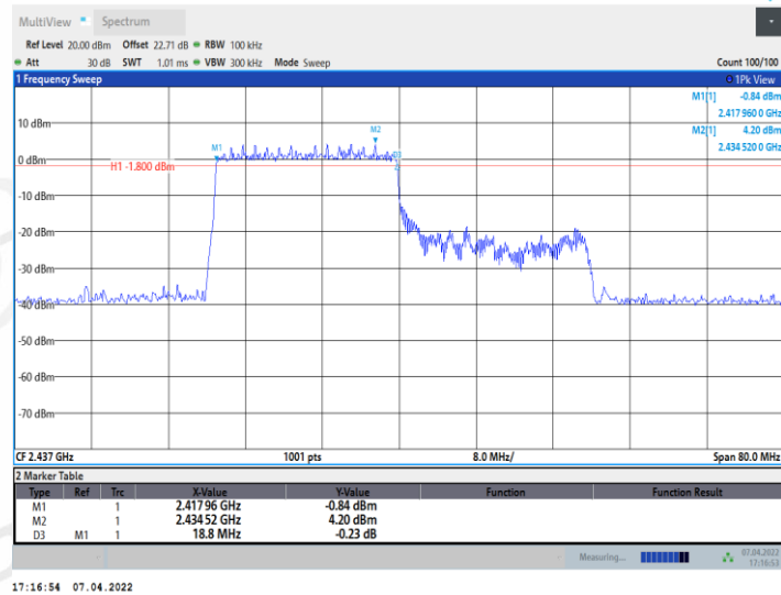
11AX40MIMO_Ant1_2437_242Tone_RU62
