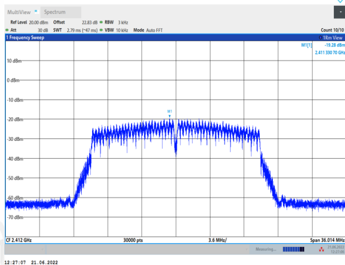
11N20MIMO_Ant2_2412
