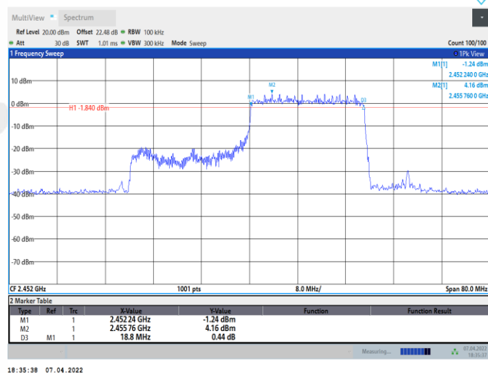
11AX40MIMO_Ant2_2452_242Tone_RU61
