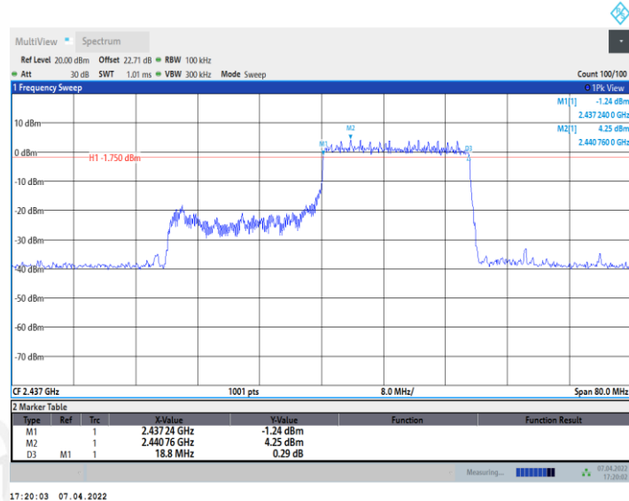
11AX40MIMO_Ant2_2437_242Tone_RU61
