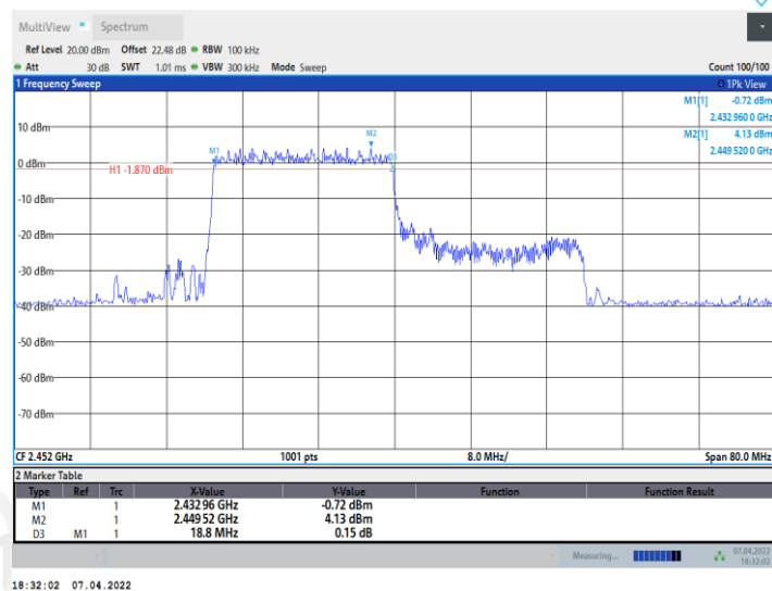
11AX40MIMO_Ant1_2452_242Tone_RU62
