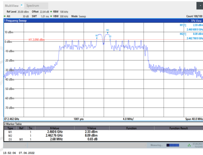
11AX20MIMO_Ant1_2462_26Tone_RU8
