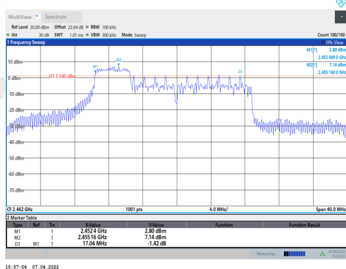
11AX20MIMO_Ant1_2462_52Tone_RU38
