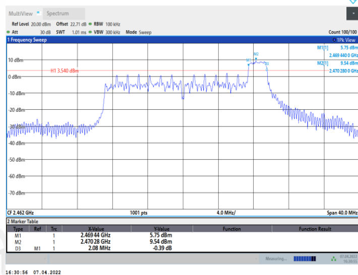
11AX20MIMO_Ant2_2462_52Tone_RU37
