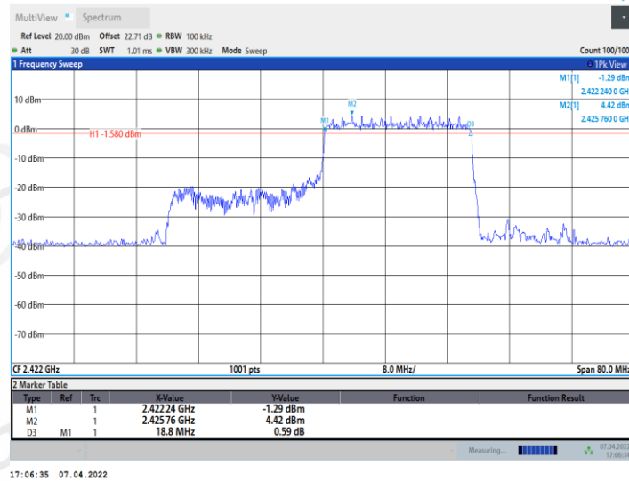
11AX40MIMO_Ant2_2422_242Tone_RU61
