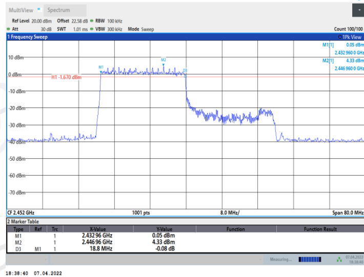
11AX40MIMO_Ant2_2452_242Tone_RU62
