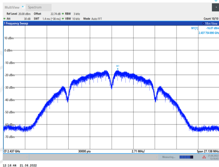
11B_Ant2_2437
