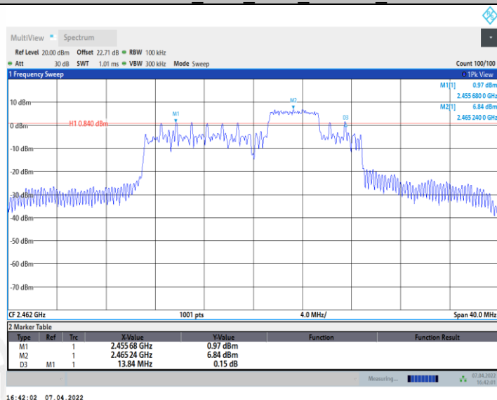
11AX20MIMO_Ant2_2462_52Tone_RU40
