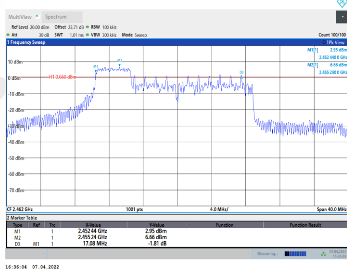
11AX20MIMO_Ant2_2462_52Tone_RU38
