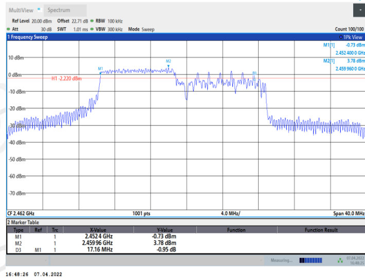
11AX20MIMO_Ant2_2462_106Tone_RU54
