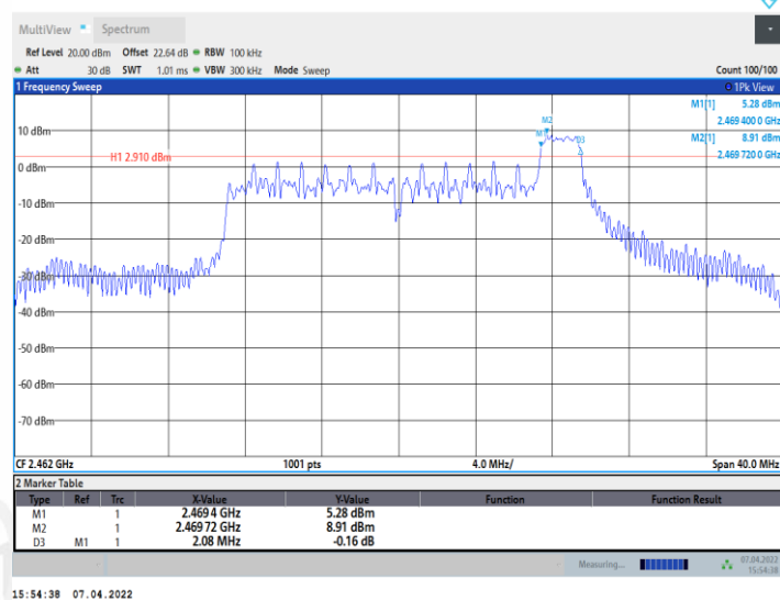
11AX20MIMO_Ant1_2462_52Tone_RU37
