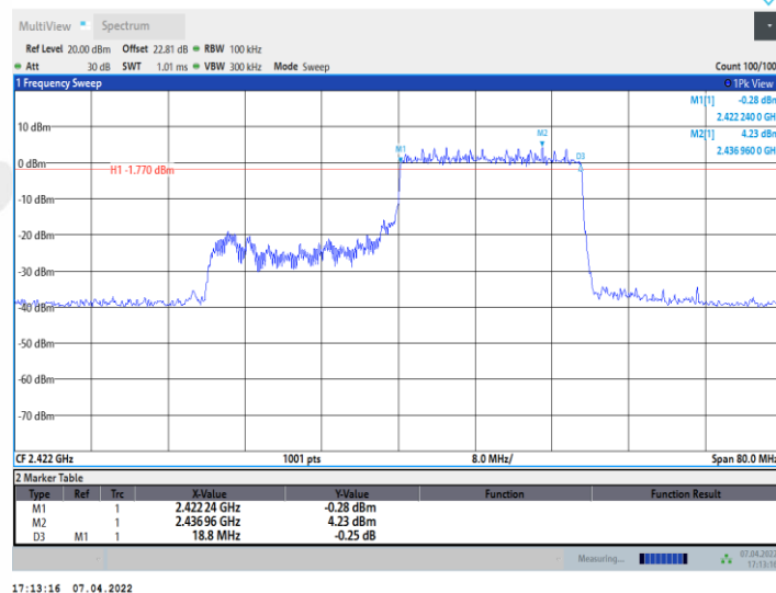
11AX40MIMO_Ant1_2437_242Tone_RU61
