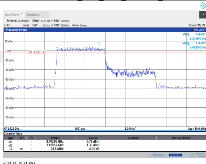
11AX40MIMO_Ant1_2422_242Tone_RU62
