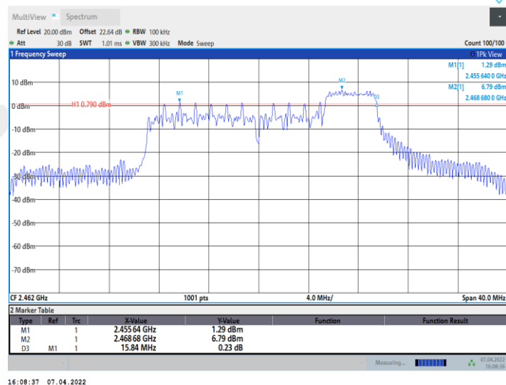
11AX20MIMO_Ant1_2462_106Tone_RU53
