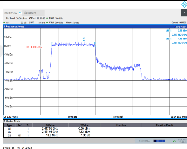
11AX40MIMO_Ant2_2437_242Tone_RU62
