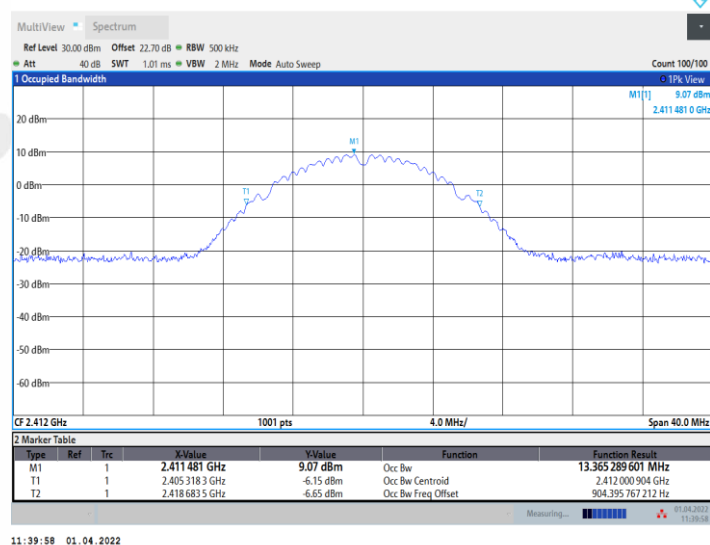
11B_Ant1_2412
