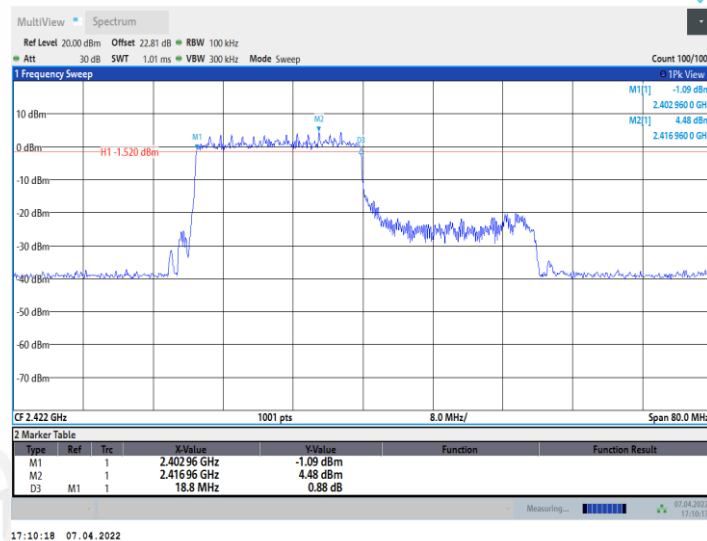
11AX40MIMO_Ant2_2422_242Tone_RU62
