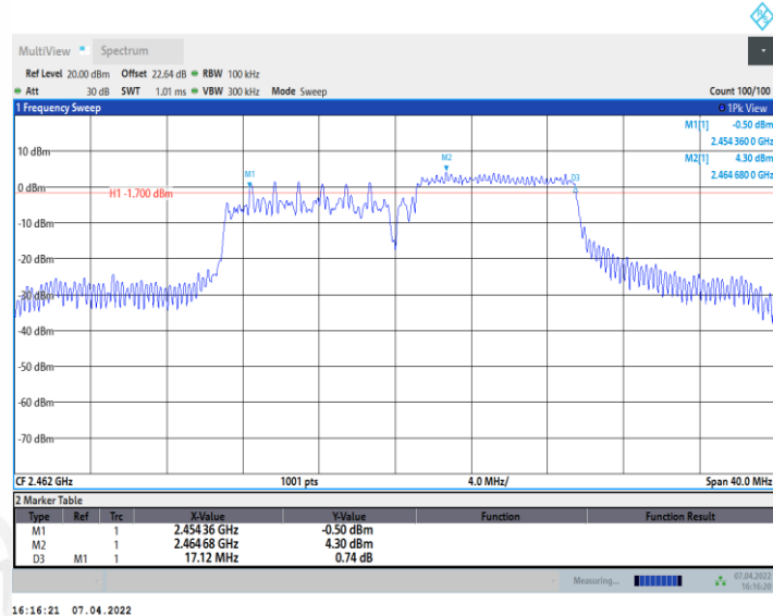
11AX20MIMO_Ant2_2462_26Tone_RU0
