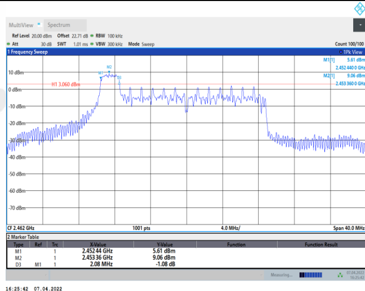
11AX20MIMO_Ant2_2462_26Tone_RU4
