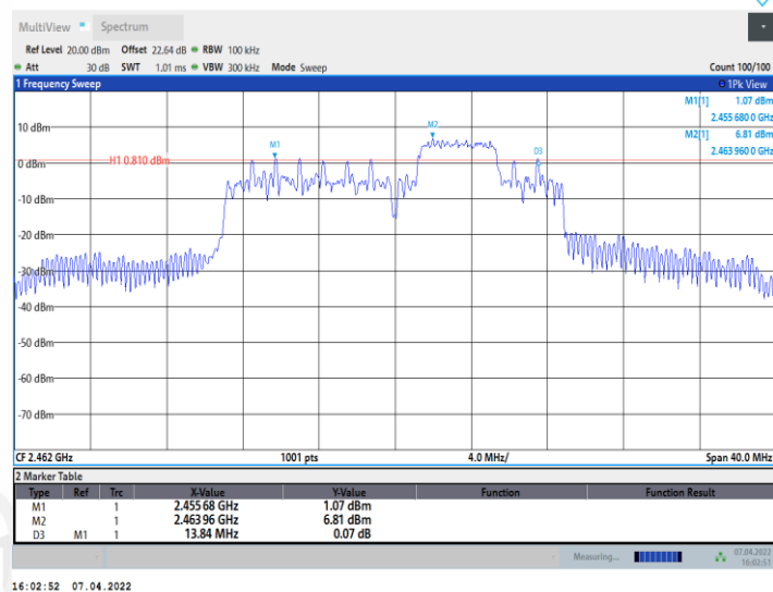
11AX20MIMO_Ant1_2462_52Tone_RU40
