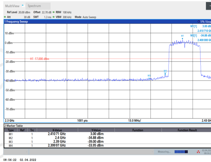
11AX20MIMO_Ant2_Low_2412
