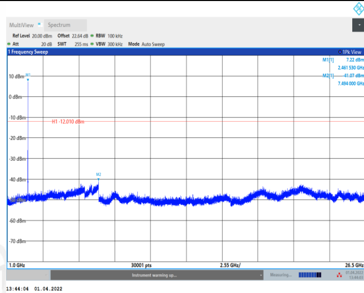
11B_Ant2_2462_0~Reference
