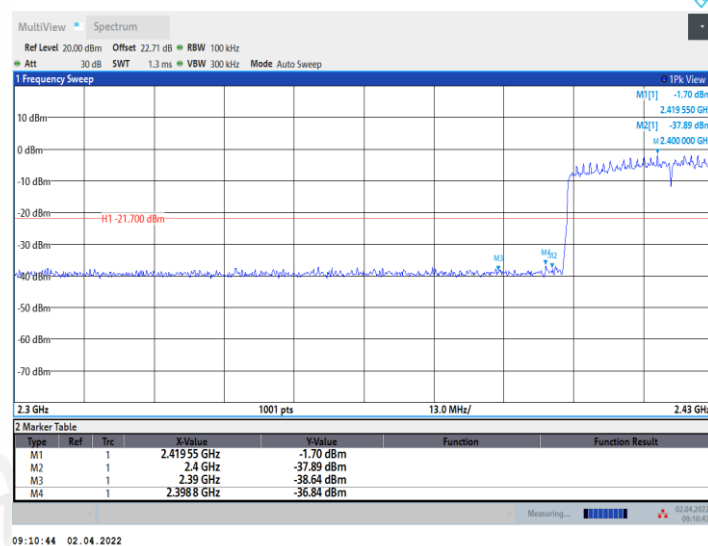
11AX40MIMO_Ant2_Low_2422
