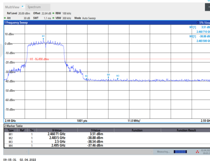
11AX20MIMO_Ant2_High_2462
