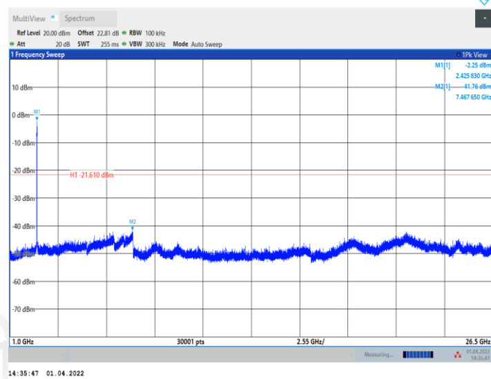
11N40MIMO_Ant1_2437_0~Reference
