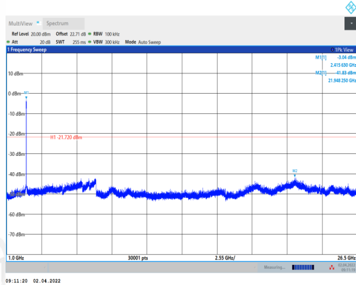
11AX40MIMO_Ant2_2422_0~Reference
