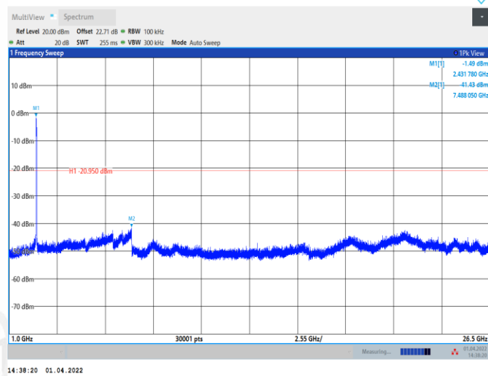
11N40MIMO_Ant2_2437_0~Reference
