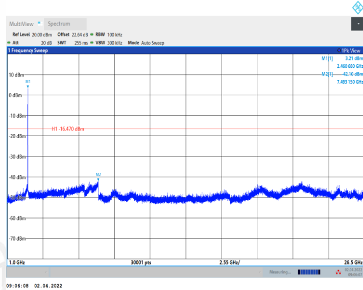
11AX20MIMO_Ant2_2462_0~Reference
