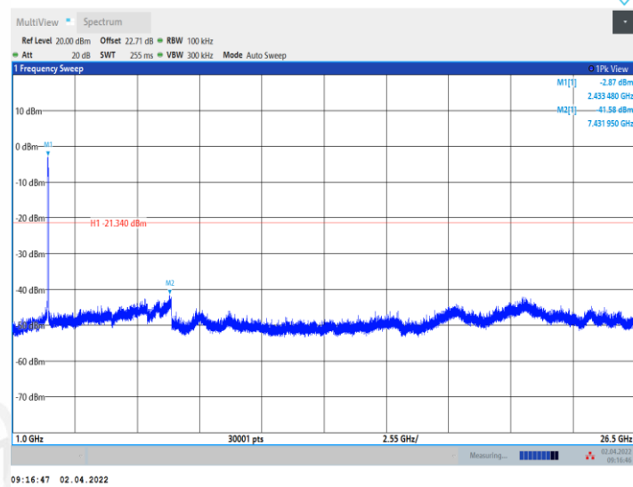
11AX40MIMO_Ant2_2437_0~Reference
