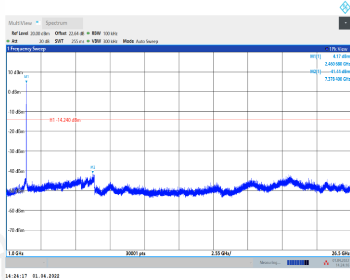
11N20MIMO_Ant2_2462_0~Reference
