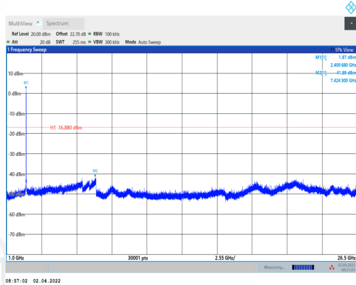
11AX20MIMO_Ant2_2412_0~Reference
