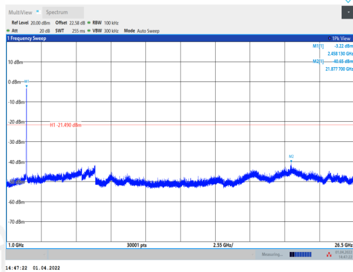
11AX20MIMO_Ant1_2412_0~Reference
