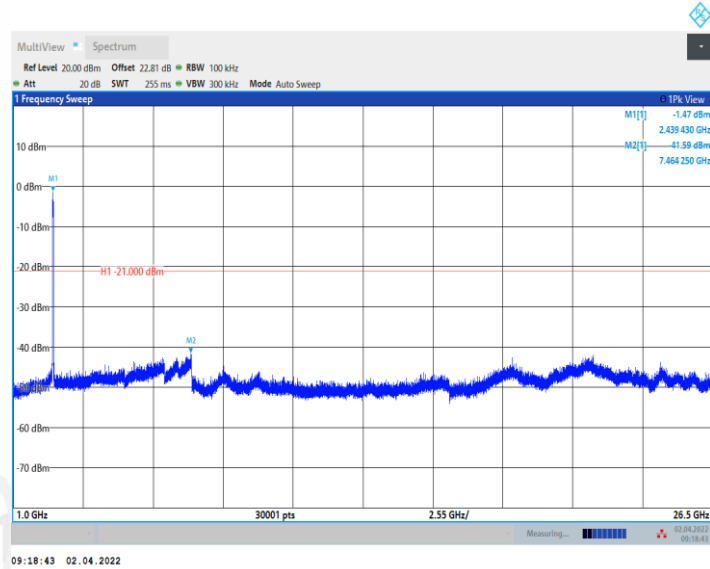
11AX40MIMO_Ant1_2452_0~Reference
