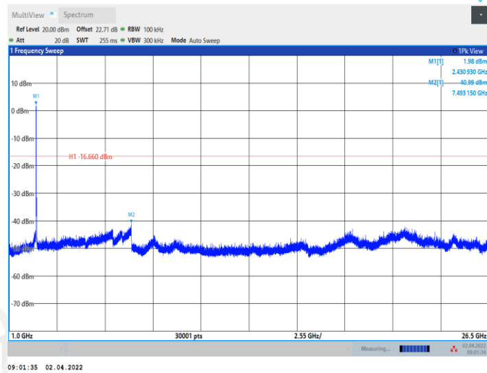
11AX20MIMO_Ant2_2437_0~Reference
