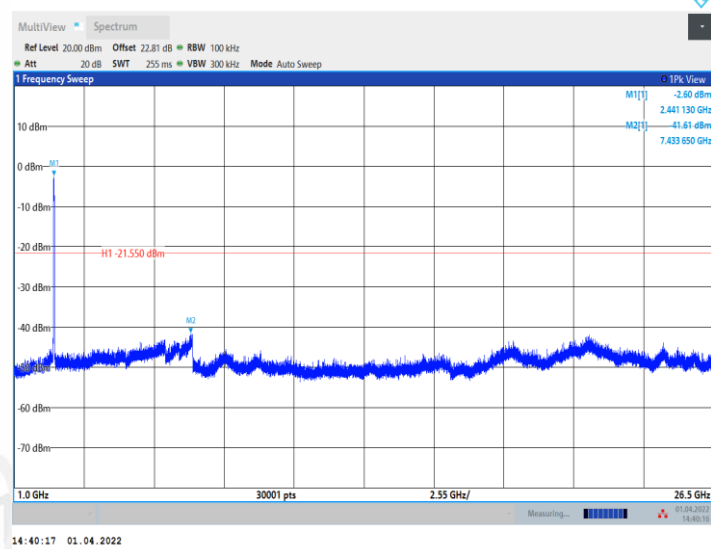
11N40MIMO_Ant1_2452_0~Reference
