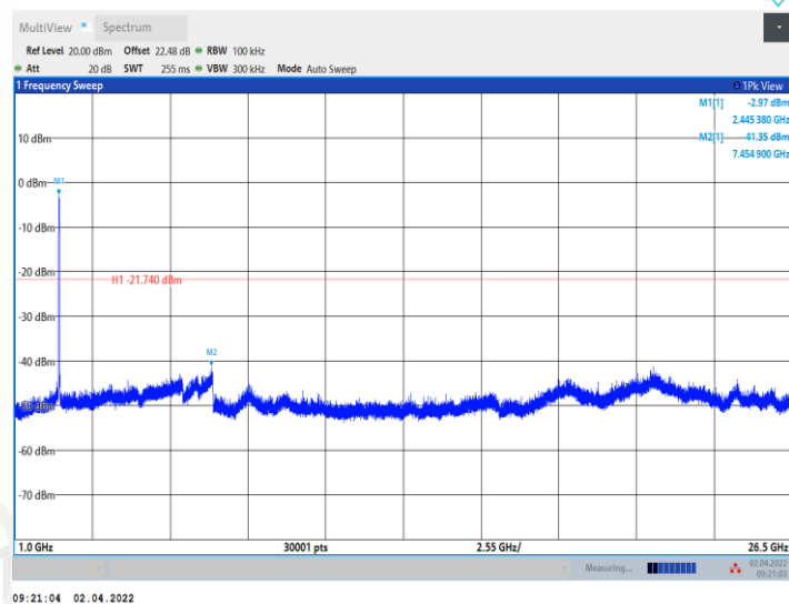
11AX40MIMO_Ant2_2452_0~Reference
