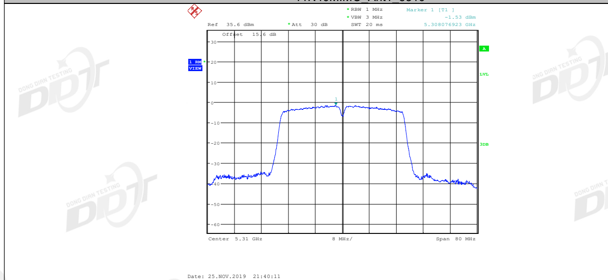
11N40MIMO Ant2 5310
