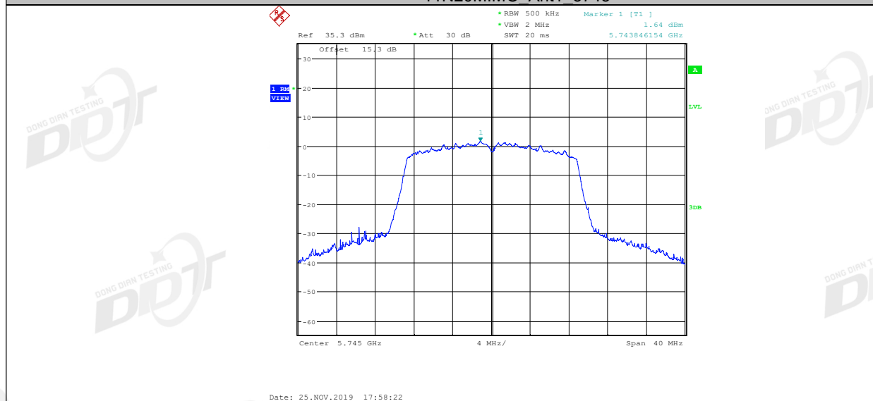
11N20MIMO_Ant2_5745
