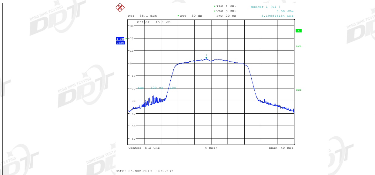
11N20MIMO Ant2 5200
