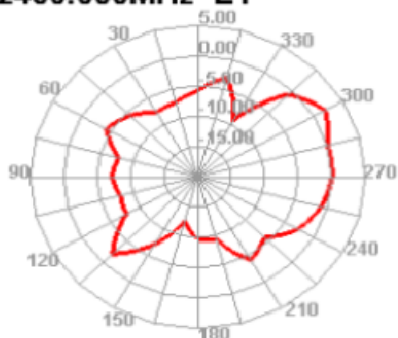
2450.000MHz E1
