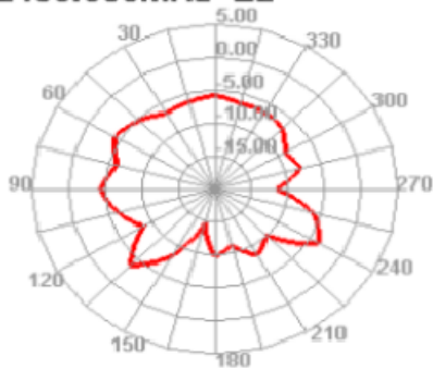
2450.000MHz E2
