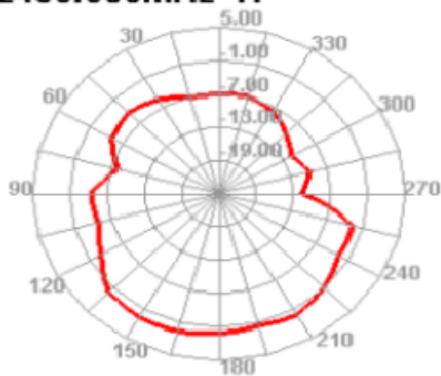
2450.000MHz H
