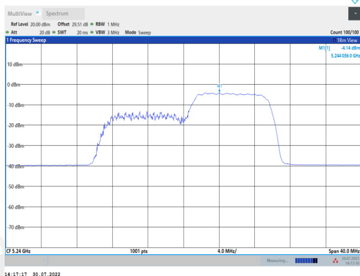
11AX20MIMO_Ant2_5240_26Tone_RU0
