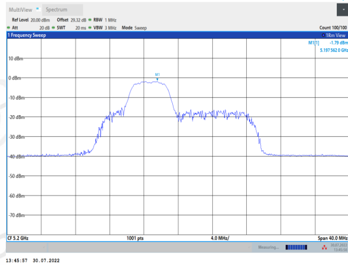
11AX20MIMO_Ant2_5200_52Tone_RU39
