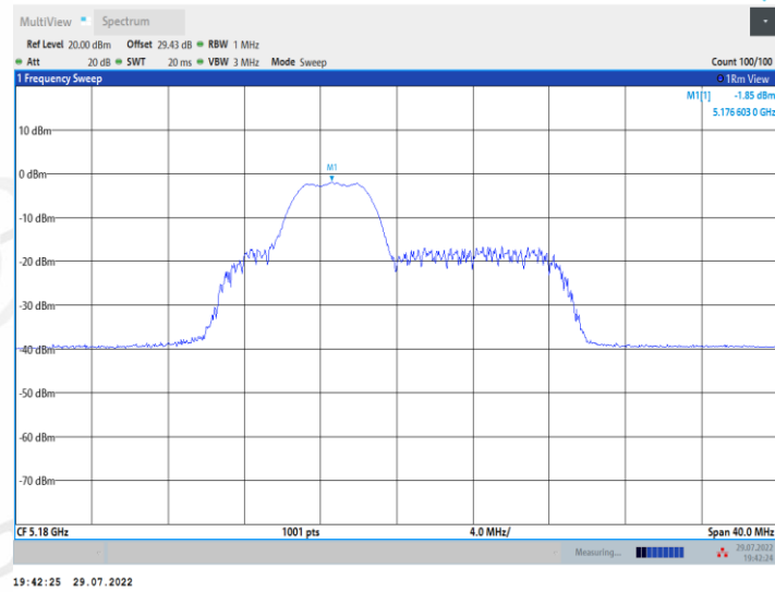
11AX20MIMO_Ant2_5180_52Tone_RU39
