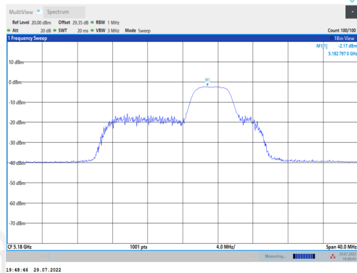
11AX20MIMO_Ant2_5180_52Tone_RU40
