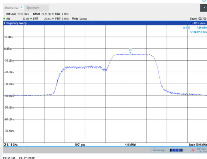
11AX20MIMO_Ant2_5180_26Tone_RU0
