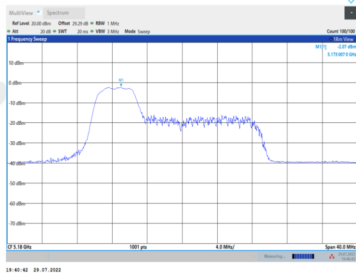
11AX20MIMO_Ant2_5180_52Tone_RU38
