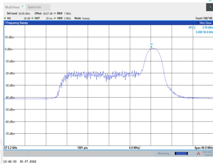
11AX20MIMO_Ant2_5200_52Tone_RU37
