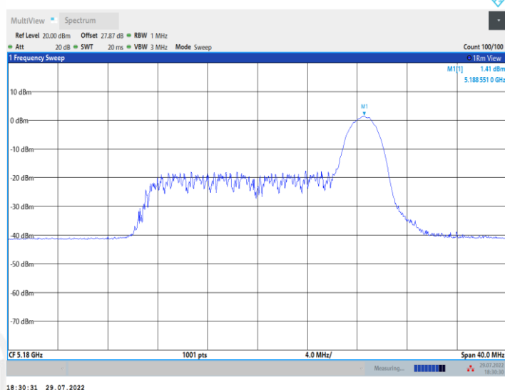
11AX20MIMO_Ant1_5180_52Tone_RU37
