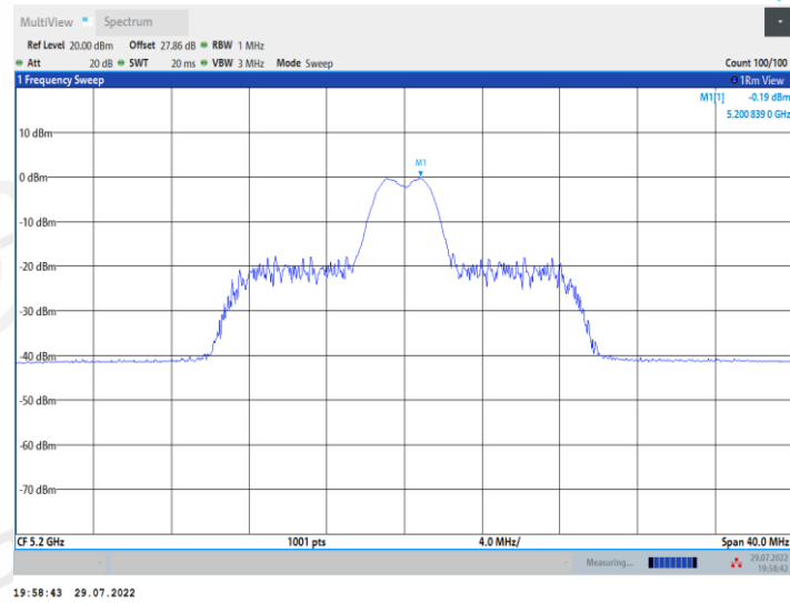
11AX20MIMO_Ant1_5200_26Tone_RU8
