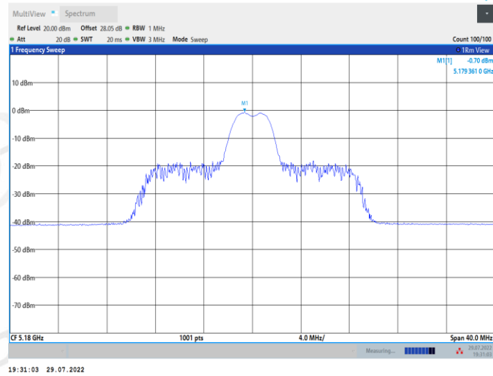
11AX20MIMO_Ant2_5180_26Tone_RU8
