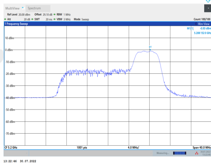
11AX20MIMO_Ant1_5200_106Tone_RU53
