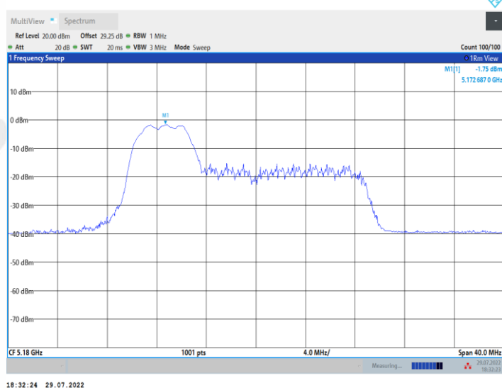
11AX20MIMO_Ant1_5180_52Tone_RU38
