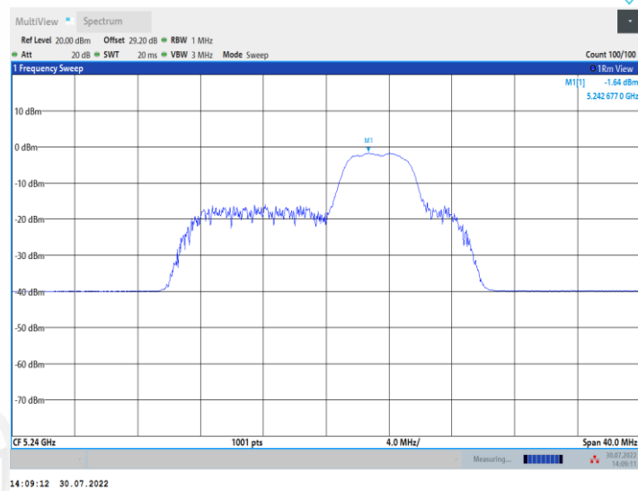
11AX20MIMO_Ant1_5240_52Tone_RU40
