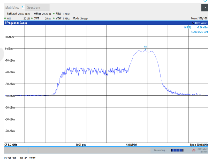
11AX20MIMO_Ant2_5200_106Tone_RU53
