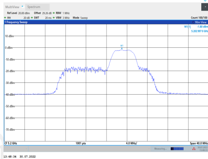
11AX20MIMO_Ant2_5200_52Tone_RU40
