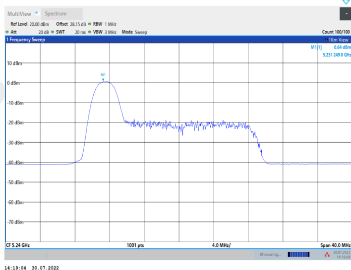
11AX20MIMO_Ant2_5240_26Tone_RU4
