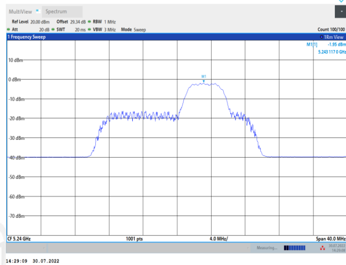
11AX20MIMO_Ant2_5240_52Tone_RU40
