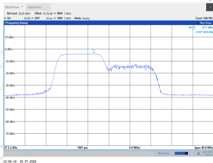
11AX20MIMO_Ant2_5200_106Tone_RU54
