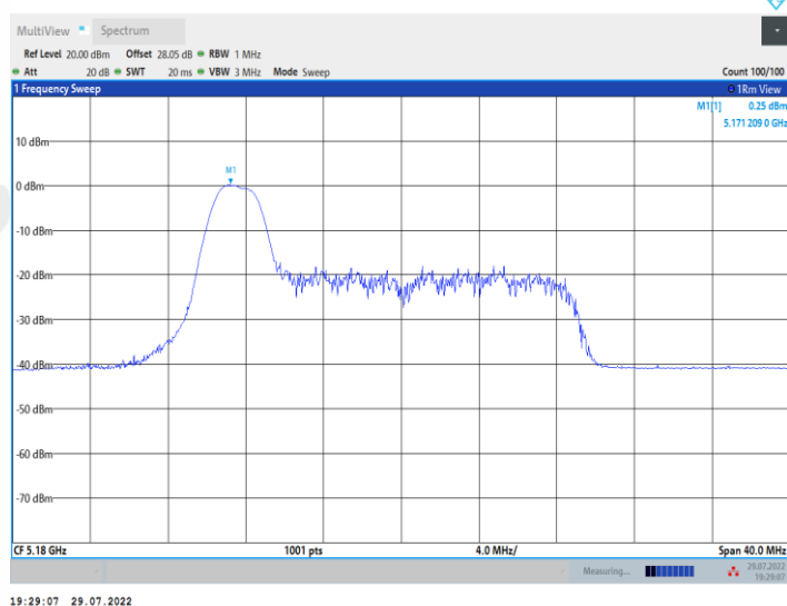
11AX20MIMO_Ant2_5180_26Tone_RU4
