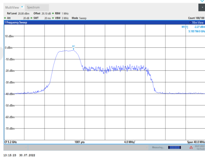
11AX20MIMO_Ant1_5200_52Tone_RU38
