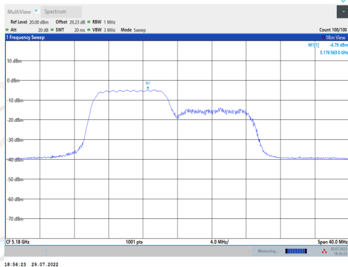
11AX20MIMO_Ant1_5180_106Tone_RU54
