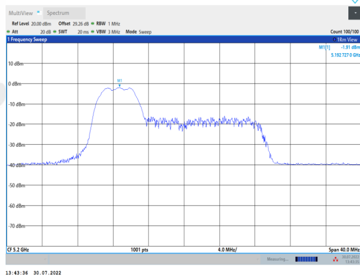
11AX20MIMO_Ant2_5200_52Tone_RU38
