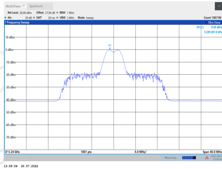
11AX20MIMO_Ant1_5240_26Tone_RU8
