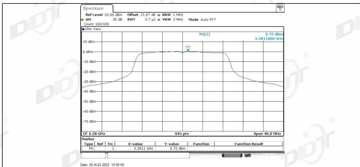
11N20MIMO Ant2 5280
