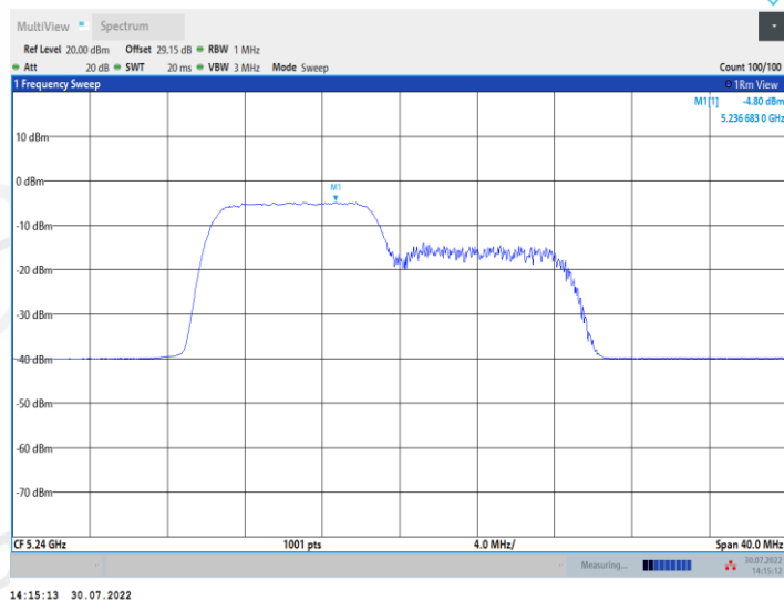
11AX20MIMO_Ant1_5240_106Tone_RU54
