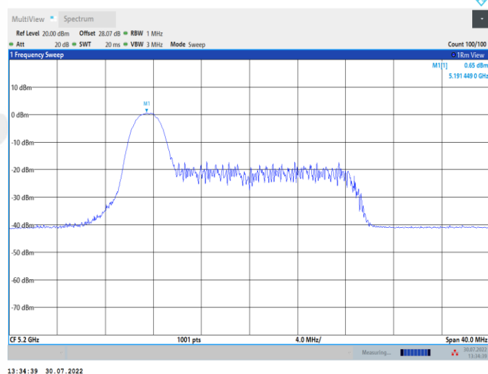
11AX20MIMO_Ant2_5200_26Tone_RU4
