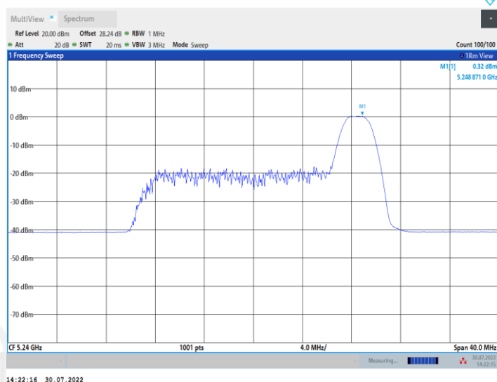
11AX20MIMO_Ant2_5240_52Tone_RU37
