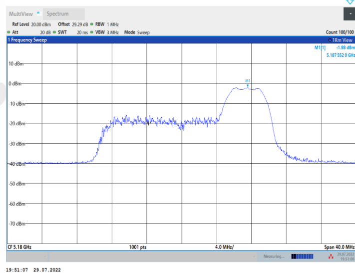
11AX20MIMO_Ant2_5180_106Tone_RU53
