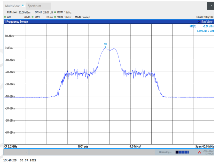
11AX20MIMO_Ant2_5200_26Tone_RU8
