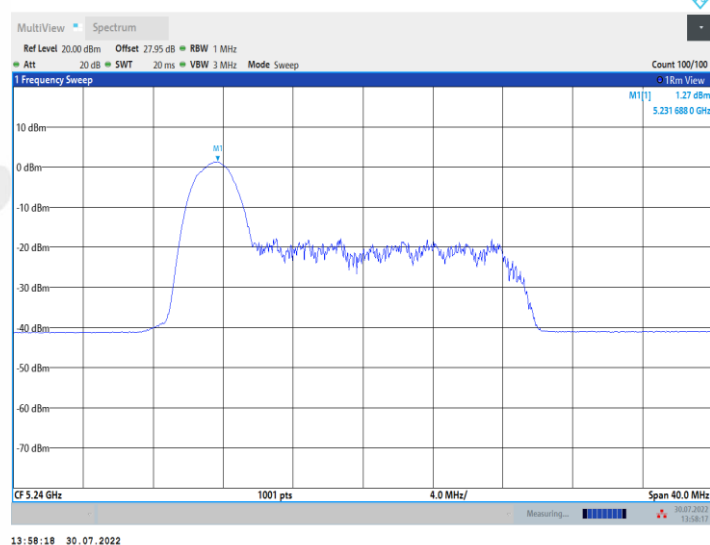
11AX20MIMO_Ant1_5240_26Tone_RU4
