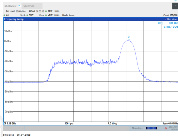
11AX20MIMO_Ant2_5180_52Tone_RU37
