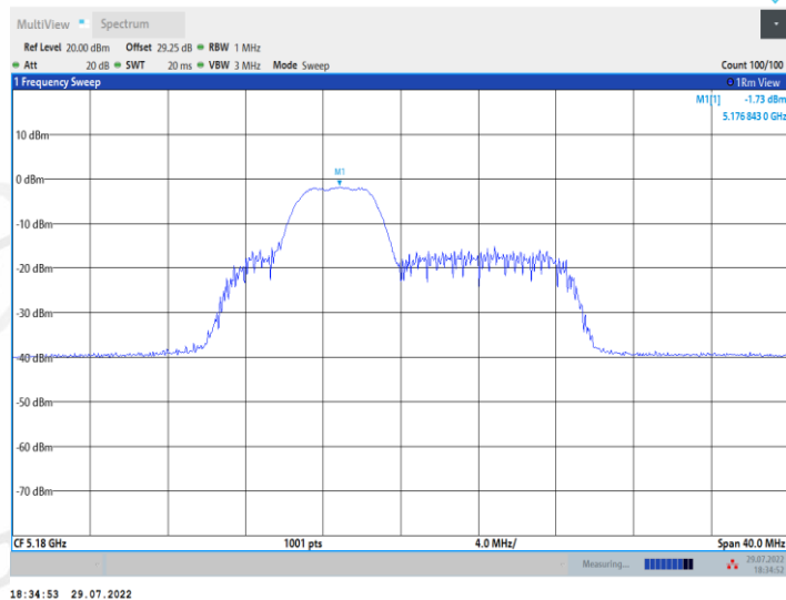
11AX20MIMO_Ant1_5180_52Tone_RU39
