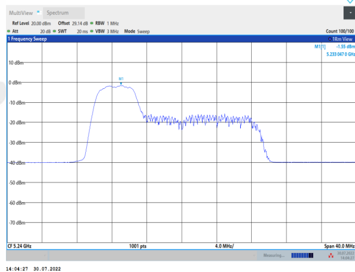
11AX20MIMO_Ant1_5240_52Tone_RU38
