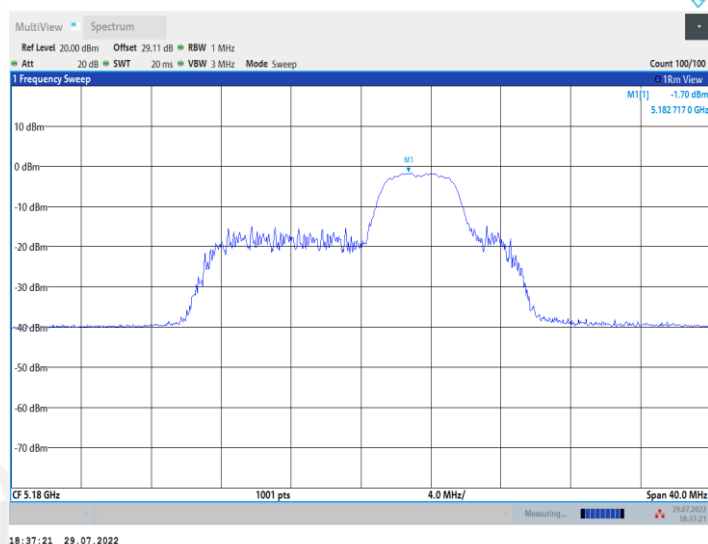
11AX20MIMO_Ant1_5180_52Tone_RU40
