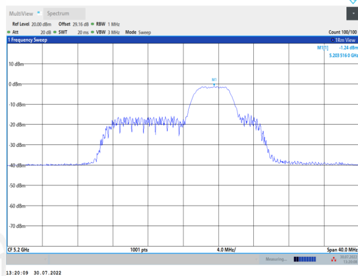
11AX20MIMO_Ant1_5200_52Tone_RU40
