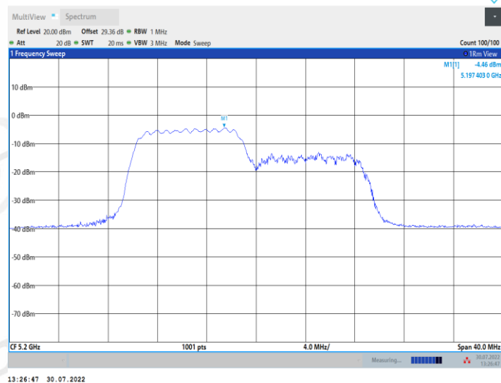
11AX20MIMO_Ant1_5200_106Tone_RU54
