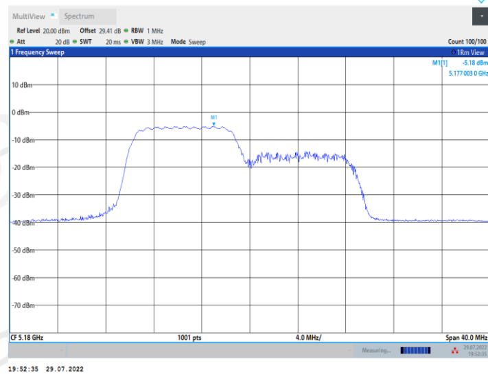
11AX20MIMO_Ant2_5180_106Tone_RU54
