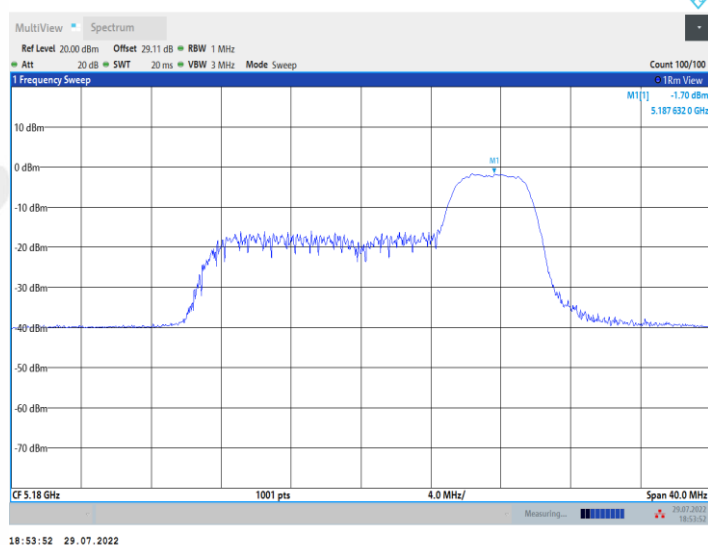
11AX20MIMO_Ant1_5180_106Tone_RU53
