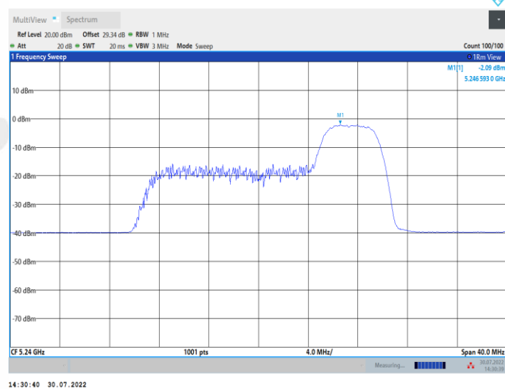
11AX20MIMO_Ant2_5240_106Tone_RU53
