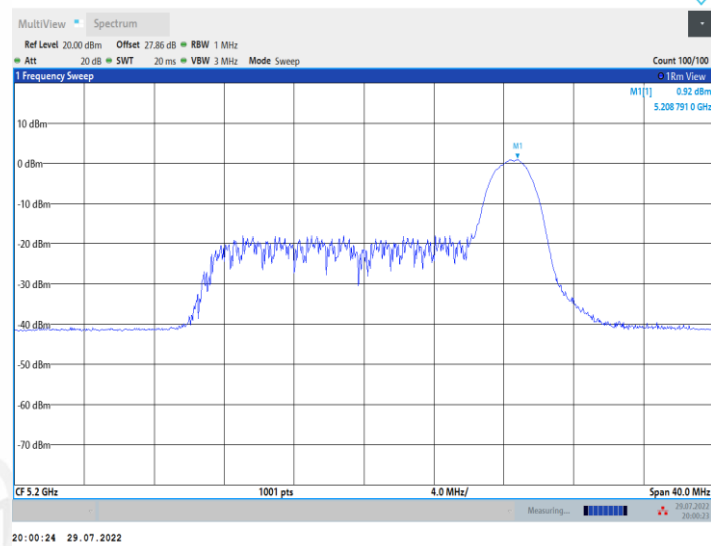
11AX20MIMO_Ant1_5200_52Tone_RU37
