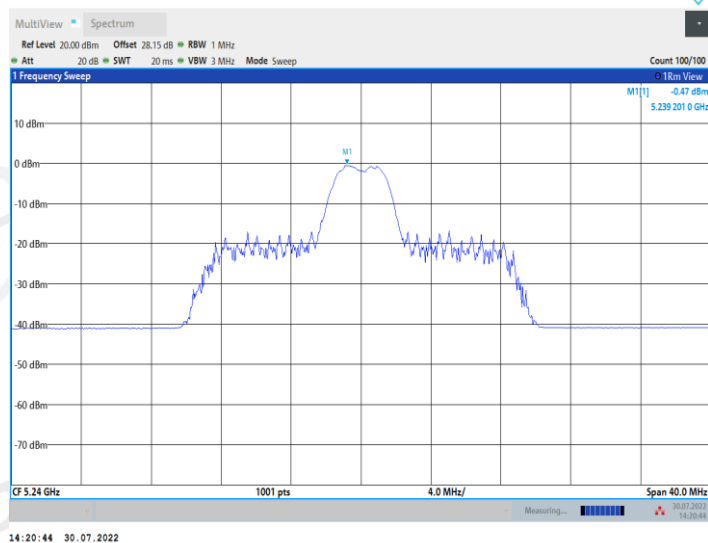
11AX20MIMO_Ant2_5240_26Tone_RU8
