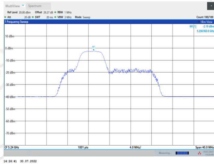
11AX20MIMO_Ant2_5240_52Tone_RU39
