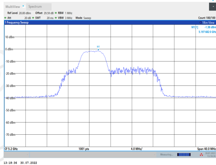
11AX20MIMO_Ant1_5200_52Tone_RU39
