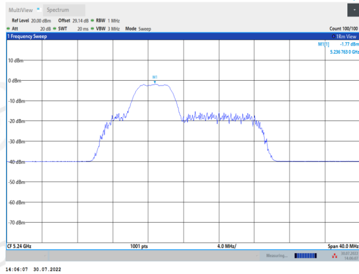
11AX20MIMO_Ant1_5240_52Tone_RU39
