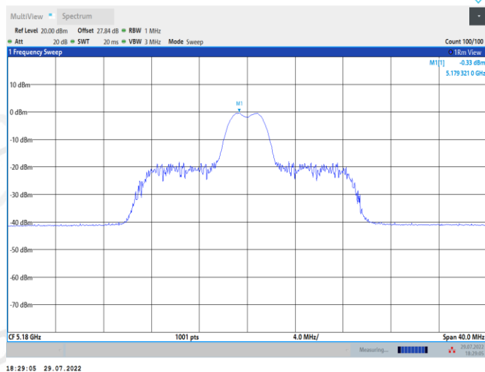
11AX20MIMO_Ant1_5180_26Tone_RU8
