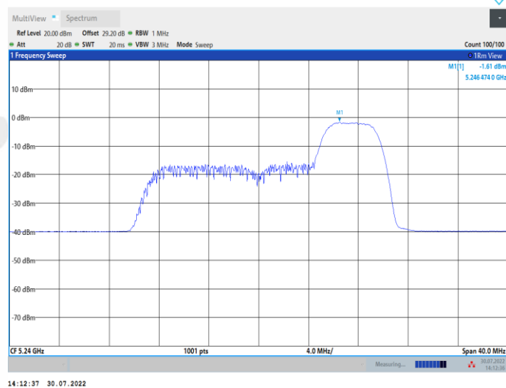
11AX20MIMO_Ant1_5240_106Tone_RU53
