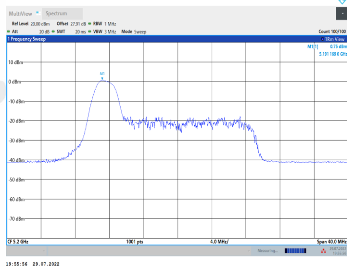
11AX20MIMO_Ant1_5200_26Tone_RU4
