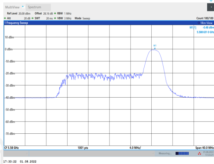
11AX20MIMO_Ant1_5580_52Tone_RU37
