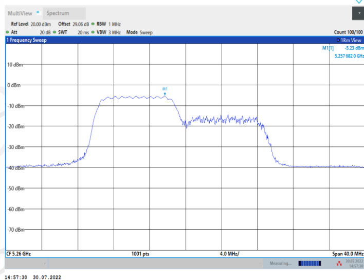
11AX20MIMO_Ant1_5260_106Tone_RU54
