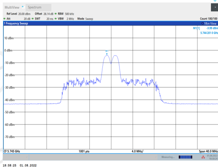
11AX20MIMO_Ant1_5745_26Tone_RU8
