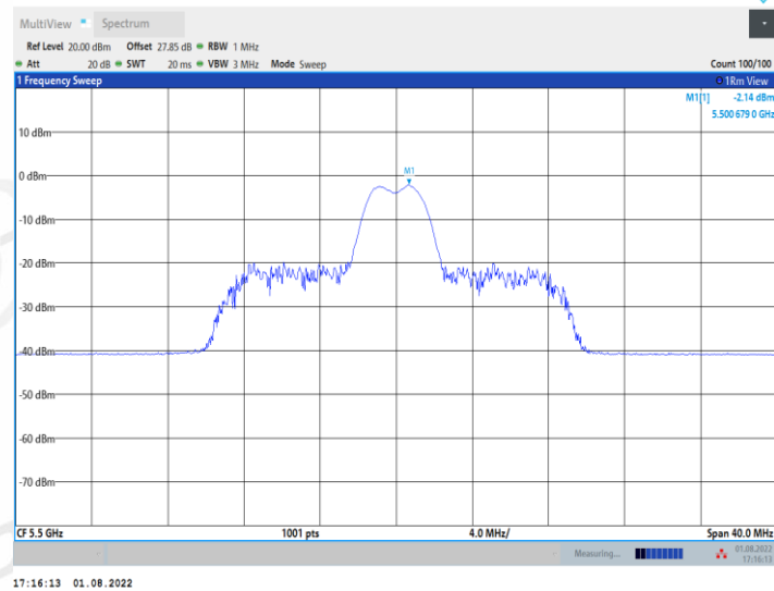
11AX20MIMO_Ant2_5500_26Tone_RU8
