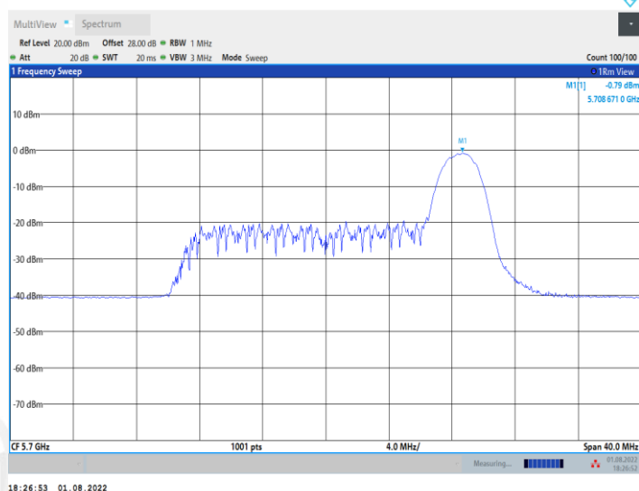
11AX20MIMO_Ant2_5700_52Tone_RU37
