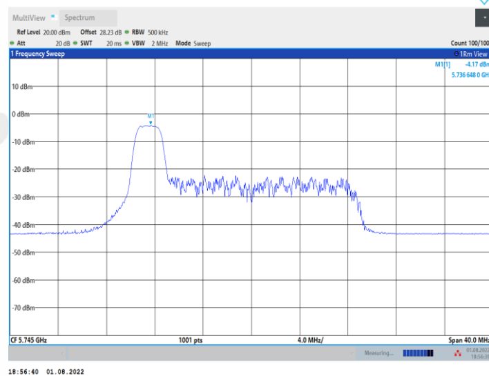
11AX20MIMO_Ant1_5745_26Tone_RU4
