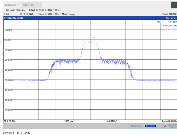
11AX20MIMO_Ant1_5260_26Tone_RU8
