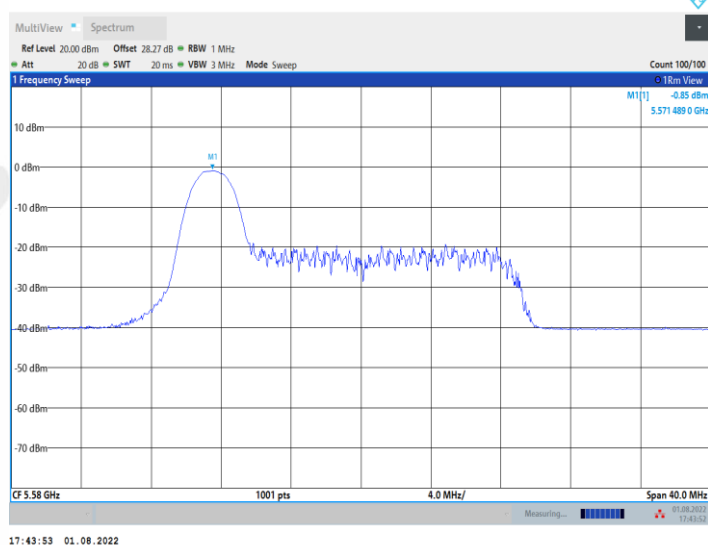
11AX20MIMO_Ant2_5580_26Tone_RU4
