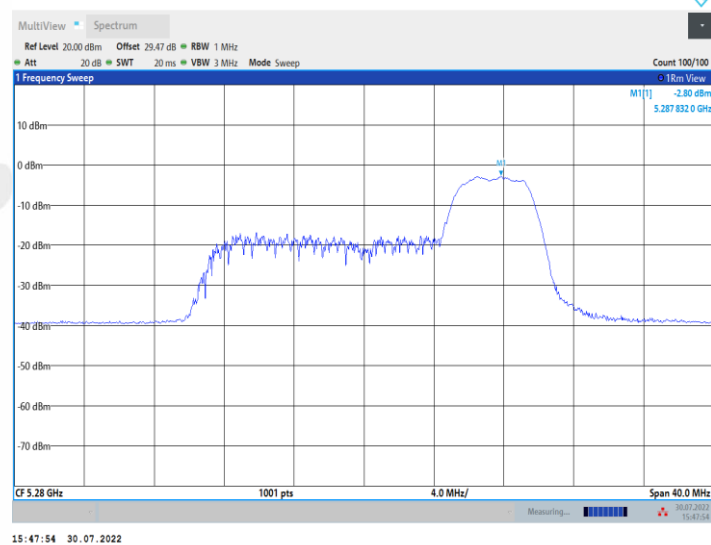
11AX20MIMO_Ant2_5280_106Tone_RU53
