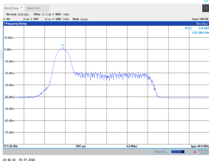
11AX20MIMO_Ant1_5260_26Tone_RU4
