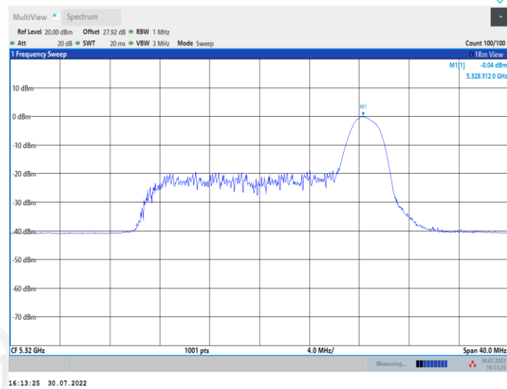
11AX20MIMO_Ant2_5320_52Tone_RU37
