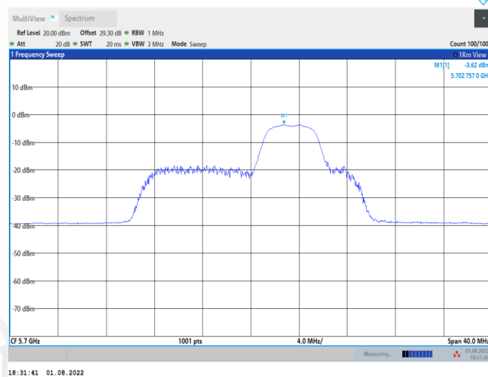
11AX20MIMO_Ant2_5700_52Tone_RU40
