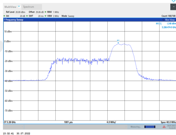
11AX20MIMO_Ant1_5280_106Tone_RU53
