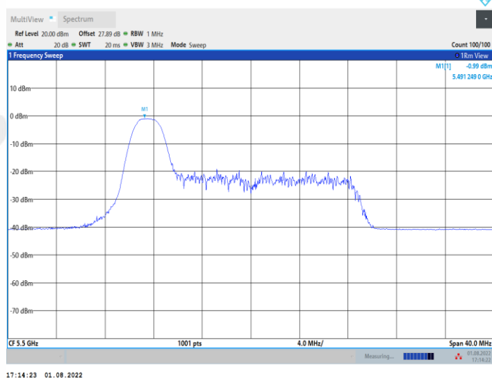
11AX20MIMO_Ant2_5500_26Tone_RU4
