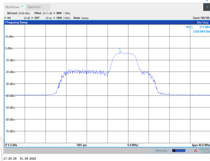
11AX20MIMO_Ant2_5500_52Tone_RU40
