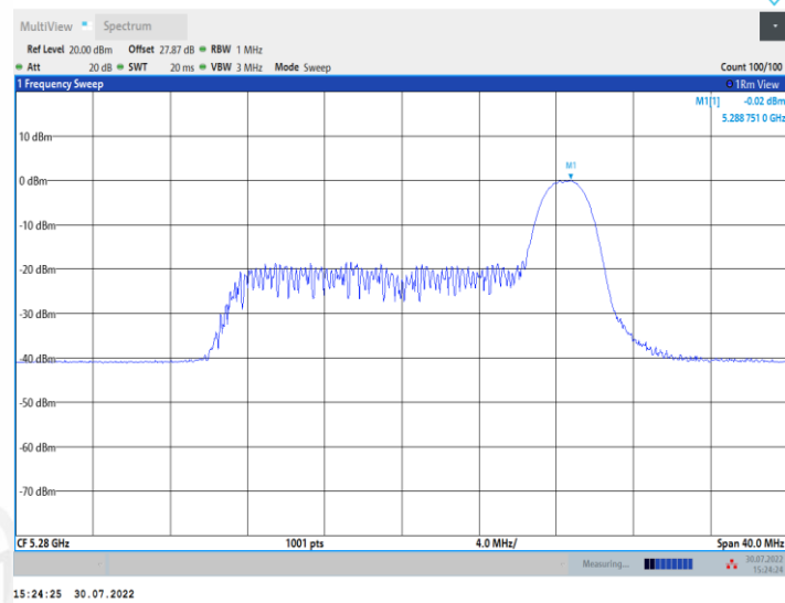
11AX20MIMO_Ant1_5280_52Tone_RU37
