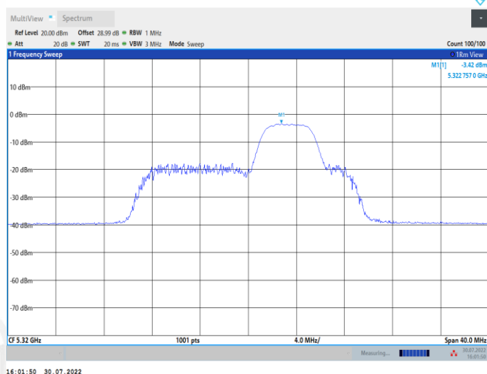
11AX20MIMO_Ant1_5320_52Tone_RU40
