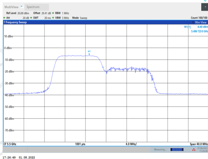
11AX20MIMO_Ant2_5500_106Tone_RU54
