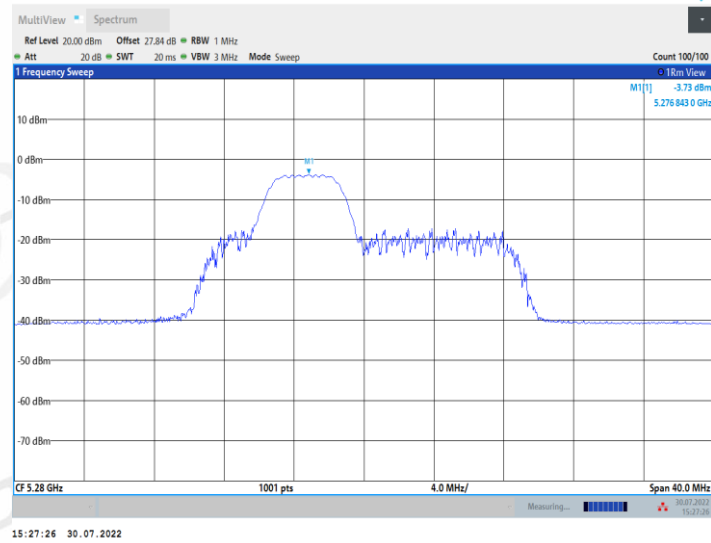
11AX20MIMO_Ant1_5280_52Tone_RU39
