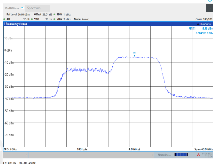
11AX20MIMO_Ant2_5500_26Tone_RU0
