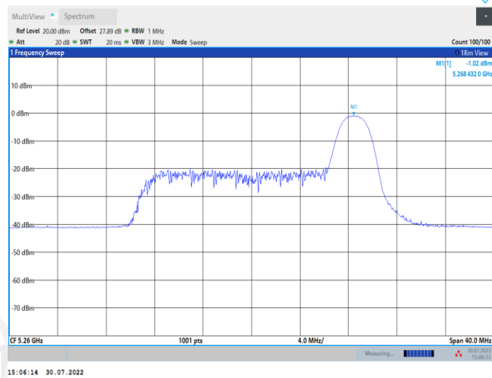
11AX20MIMO_Ant2_5260_52Tone_RU37
