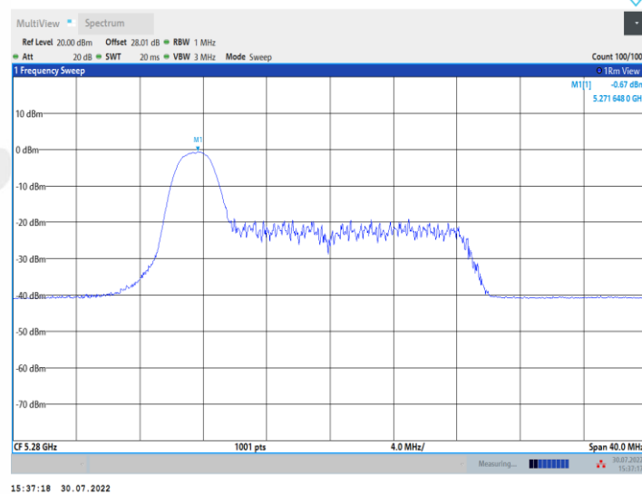
11AX20MIMO_Ant2_5280_26Tone_RU4
