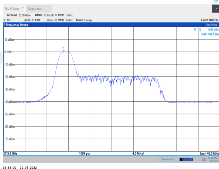
11AX20MIMO_Ant1_5500_26Tone_RU4
