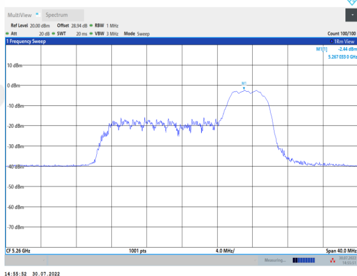
11AX20MIMO_Ant1_5260_106Tone_RU53
