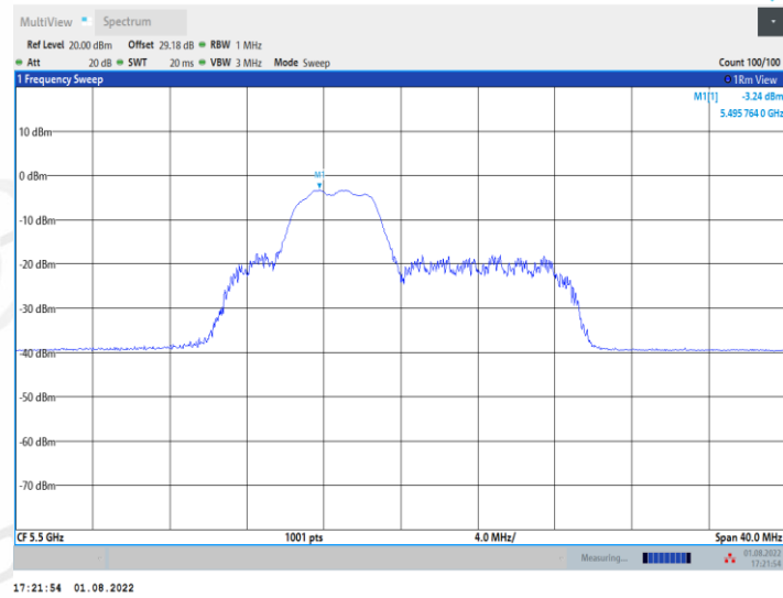
11AX20MIMO_Ant2_5500_52Tone_RU39
