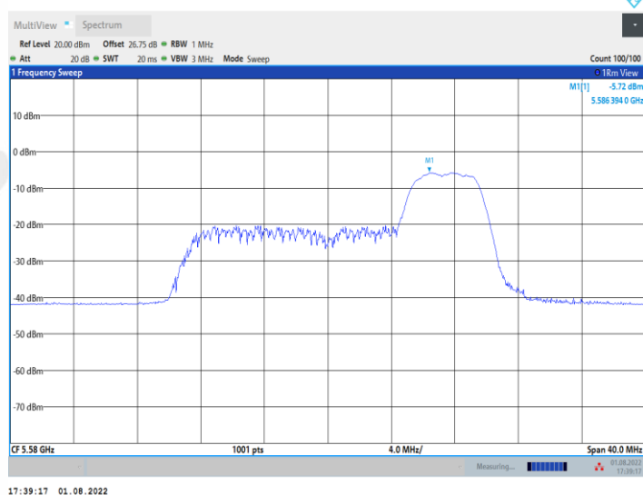
11AX20MIMO_Ant1_5580_106Tone_RU53
