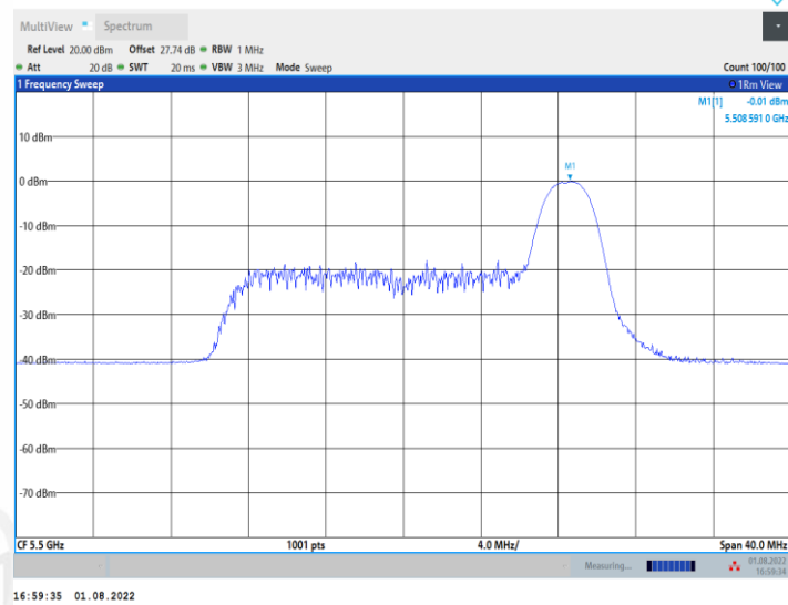
11AX20MIMO_Ant1_5500_52Tone_RU37
