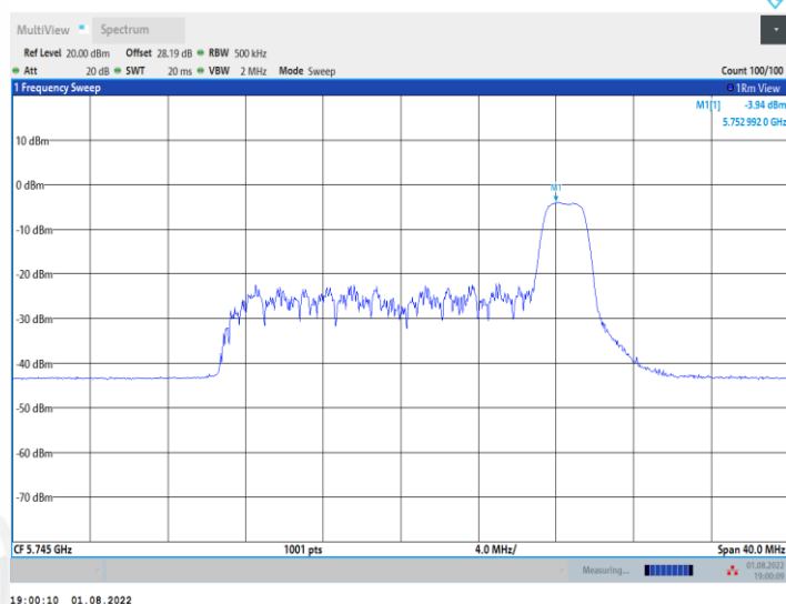
11AX20MIMO_Ant1_5745_52Tone_RU37
