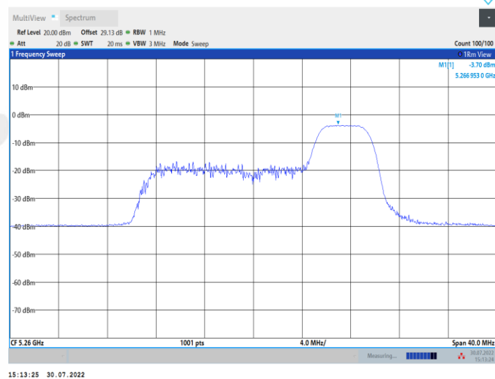
11AX20MIMO_Ant2_5260_106Tone_RU53
