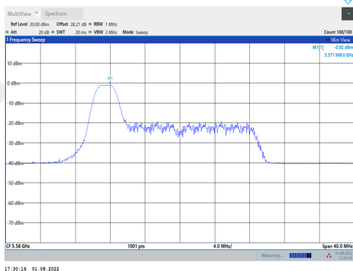
11AX20MIMO_Ant1_5580_26Tone_RU4
