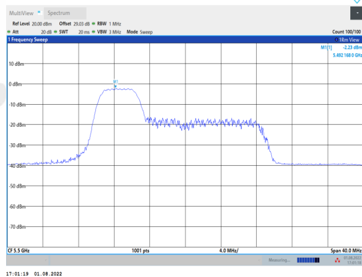
11AX20MIMO_Ant1_5500_52Tone_RU38
