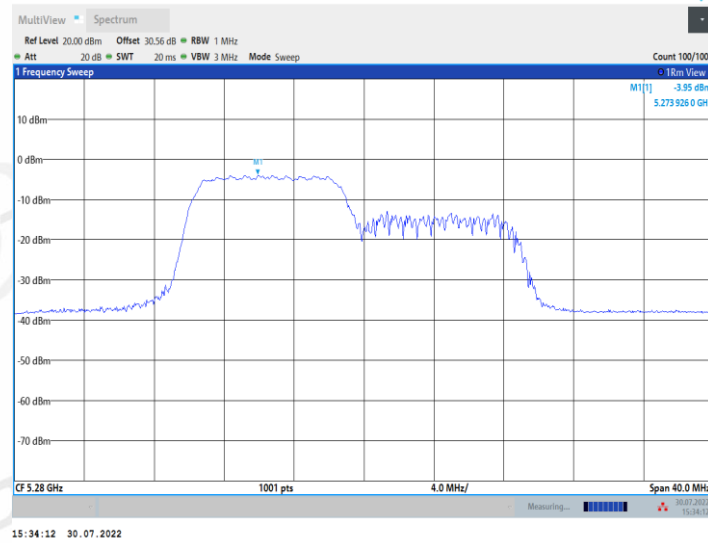
11AX20MIMO_Ant1_5280_106Tone_RU54
