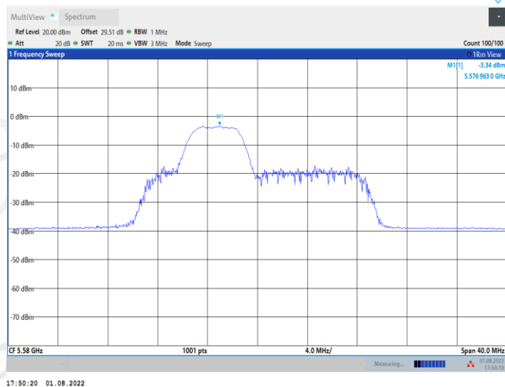
11AX20MIMO_Ant2_5580_52Tone_RU39
