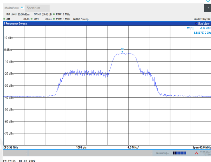
11AX20MIMO_Ant1_5580_52Tone_RU40
