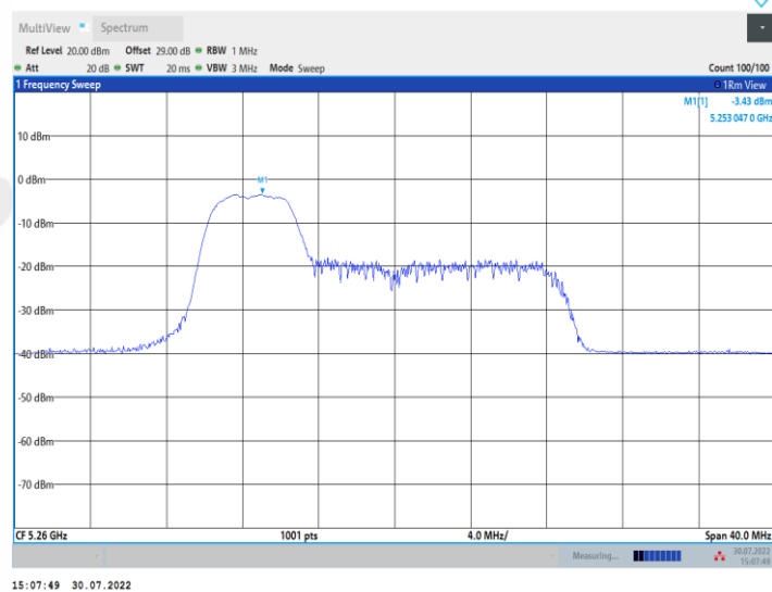
11AX20MIMO_Ant2_5260_52Tone_RU38
