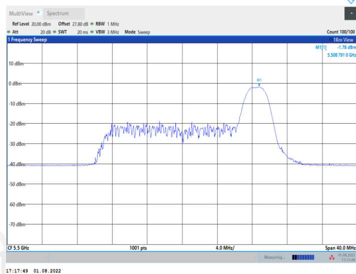
11AX20MIMO_Ant2_5500_52Tone_RU37
