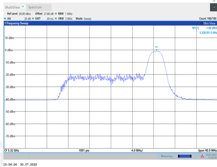
11AX20MIMO_Ant1_5320_52Tone_RU37
