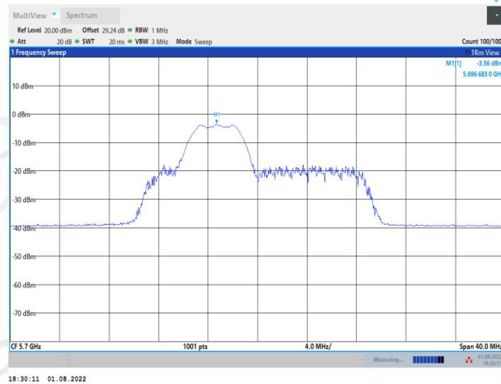
11AX20MIMO_Ant2_5700_52Tone_RU39
