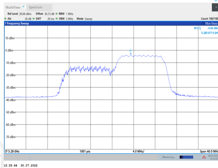
11AX20MIMO_Ant2_5280_26Tone_RU54
