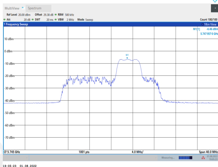
11AX20MIMO_Ant1_5745_52Tone_RU40
