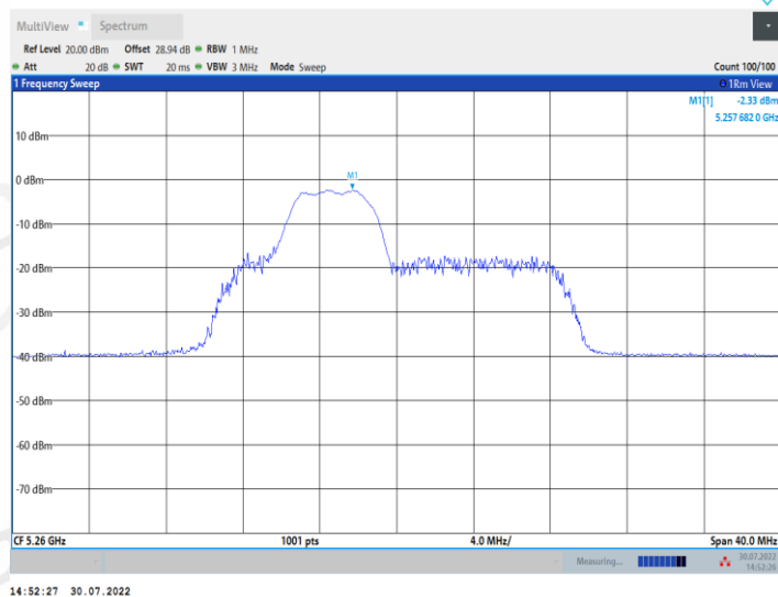
11AX20MIMO_Ant1_5260_52Tone_RU39
