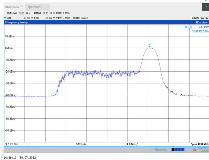
11AX20MIMO_Ant1_5260_52Tone_RU37
