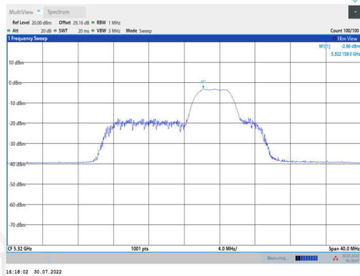
11AX20MIMO_Ant2_5320_52Tone_RU40
