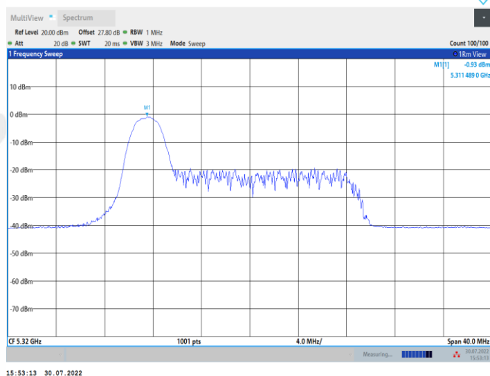
11AX20MIMO_Ant1_5320_26Tone_RU4
