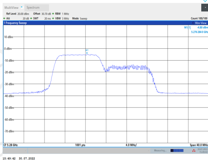
11AX20MIMO_Ant2_5280_106Tone_RU54
