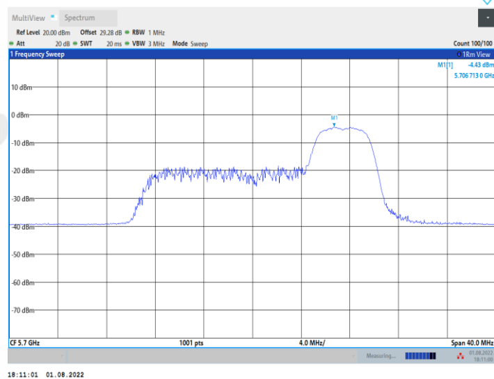
11AX20MIMO_Ant1_5700_106Tone_RU53
