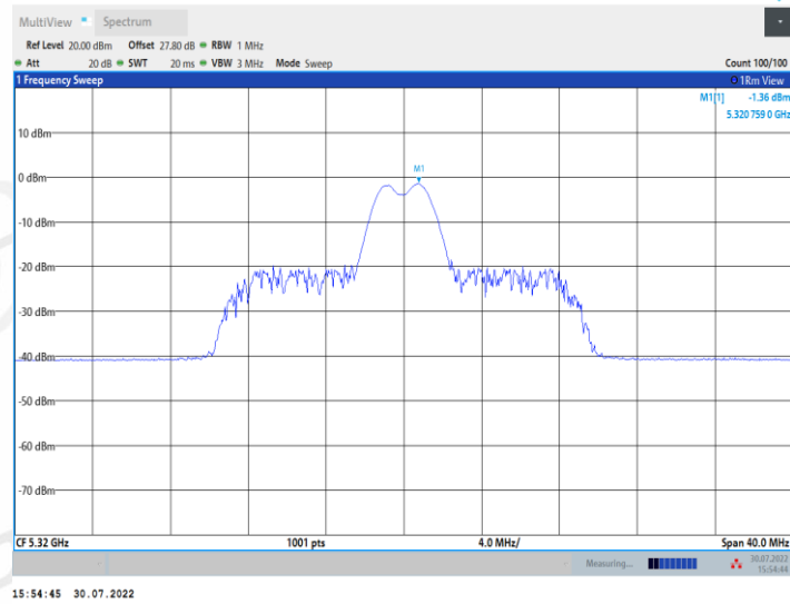
11AX20MIMO_Ant1_5320_26Tone_RU8
