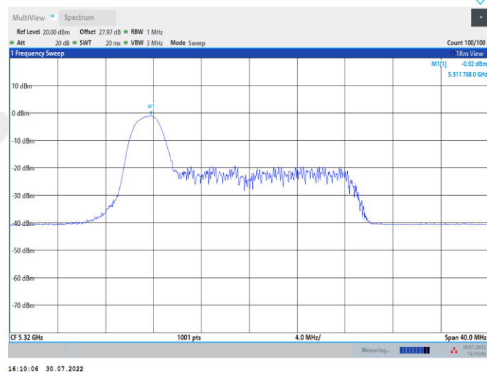
11AX20MIMO_Ant2_5320_26Tone_RU4
