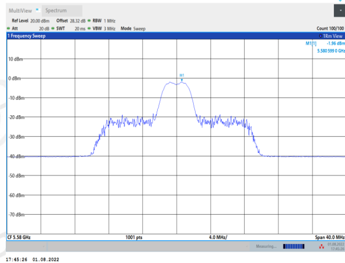
11AX20MIMO_Ant2_5580_26Tone_RU8
