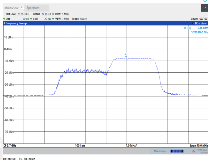
11AX20MIMO_Ant2_5700_26Tone_RU0
