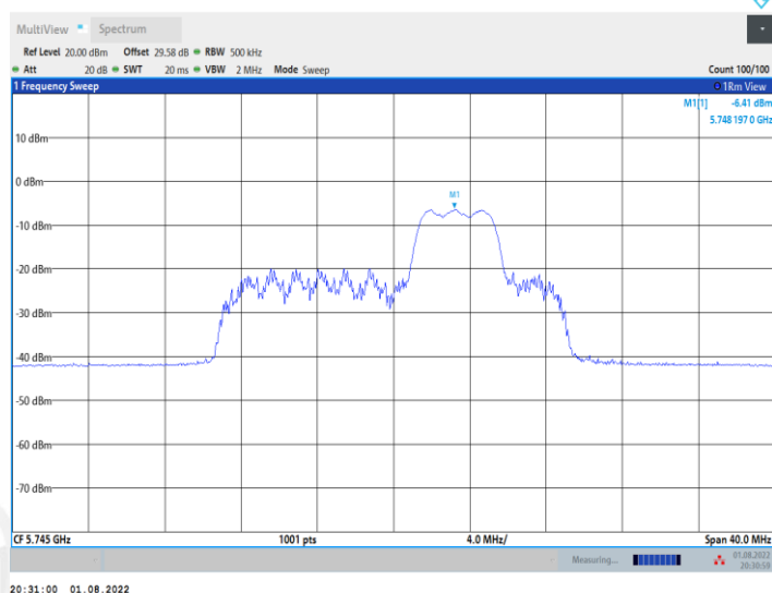
11AX20MIMO_Ant2_5745_52Tone_RU40
