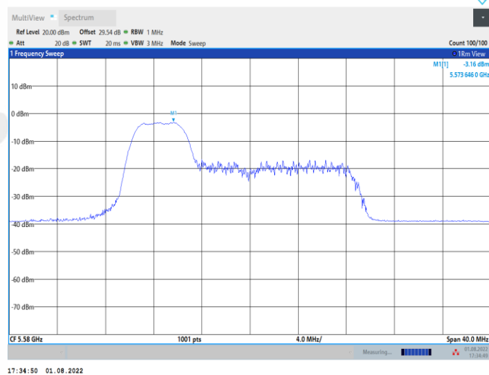
11AX20MIMO_Ant1_5580_52Tone_RU38
