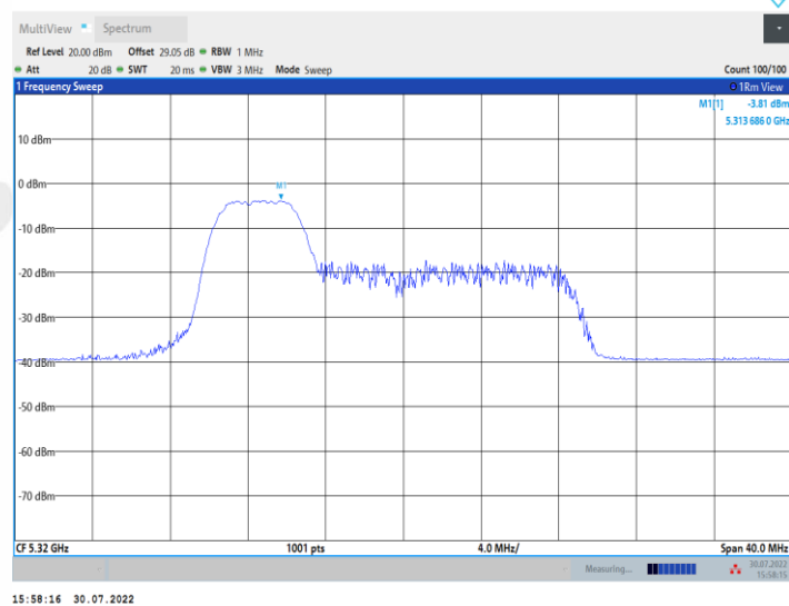
11AX20MIMO_Ant1_5320_52Tone_RU38
