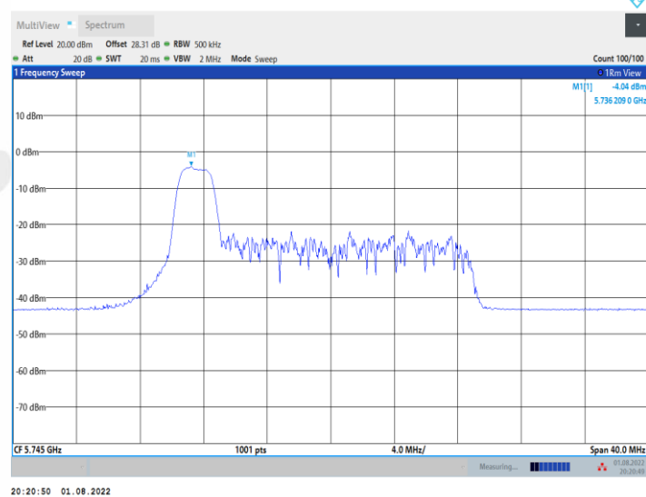
11AX20MIMO_Ant2_5745_26Tone_RU4
