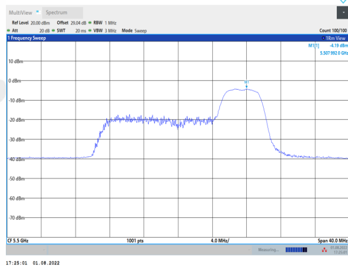
11AX20MIMO_Ant2_5500_106Tone_RU53
