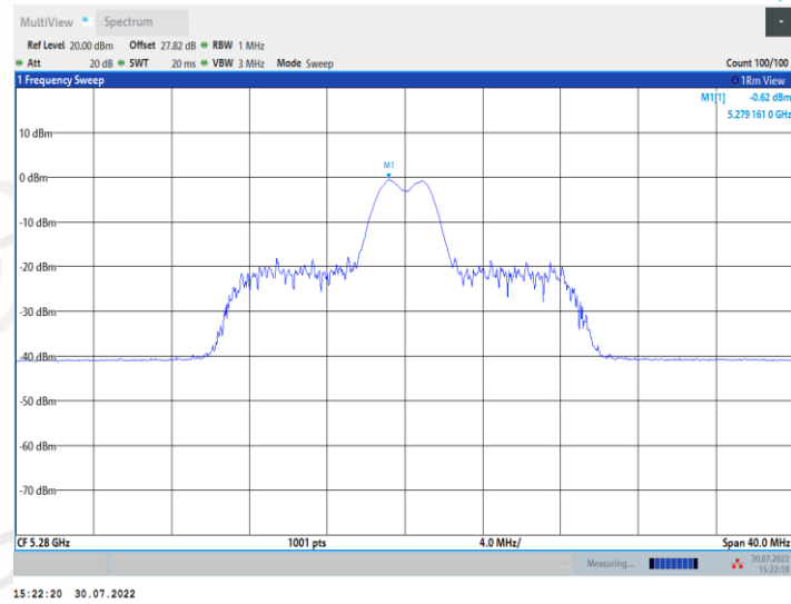
11AX20MIMO_Ant1_5280_26Tone_RU8
