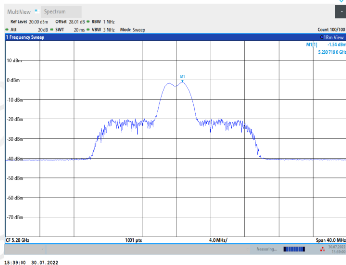
11AX20MIMO_Ant2_5280_26Tone_RU8
