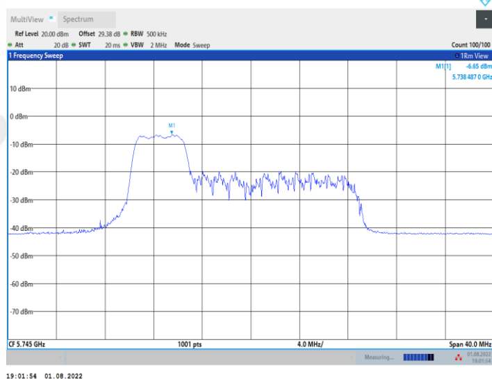
11AX20MIMO_Ant1_5745_52Tone_RU38
