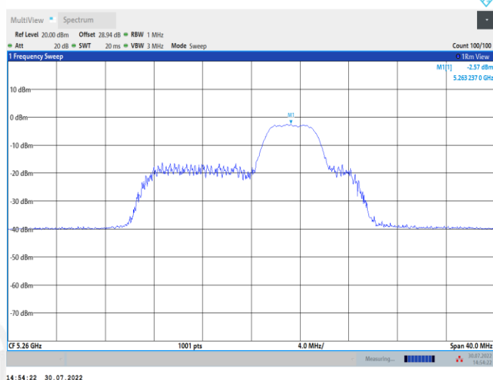
11AX20MIMO_Ant1_5260_52Tone_RU40
