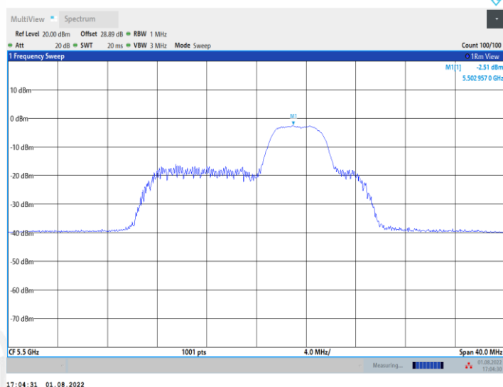
11AX20MIMO_Ant1_5500_52Tone_RU40
