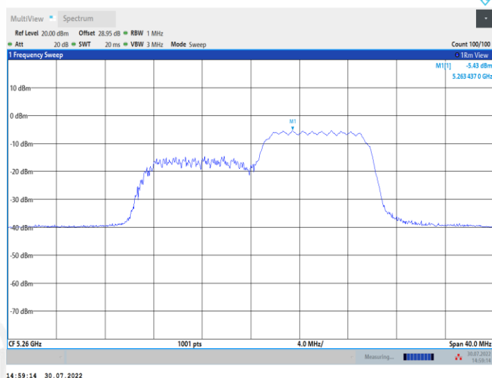
11AX20MIMO_Ant2_5260_26Tone_RU0
