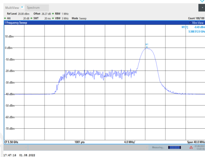
11AX20MIMO_Ant2_5580_52Tone_RU37
