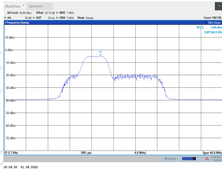
11AX20MIMO_Ant1_5700_52Tone_RU39
