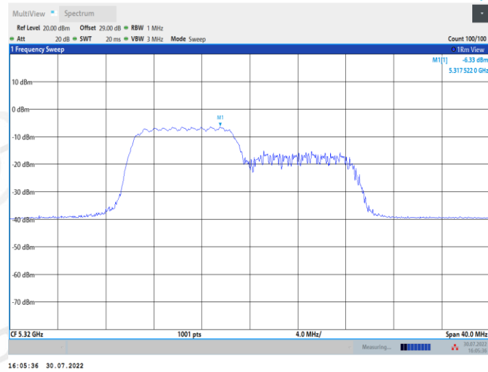
11AX20MIMO_Ant1_5320_106Tone_RU54
