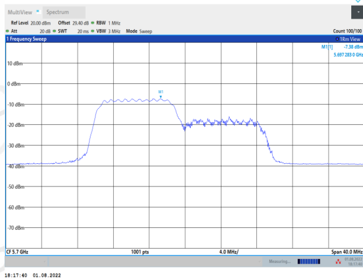
11AX20MIMO_Ant1_5700_106Tone_RU54
