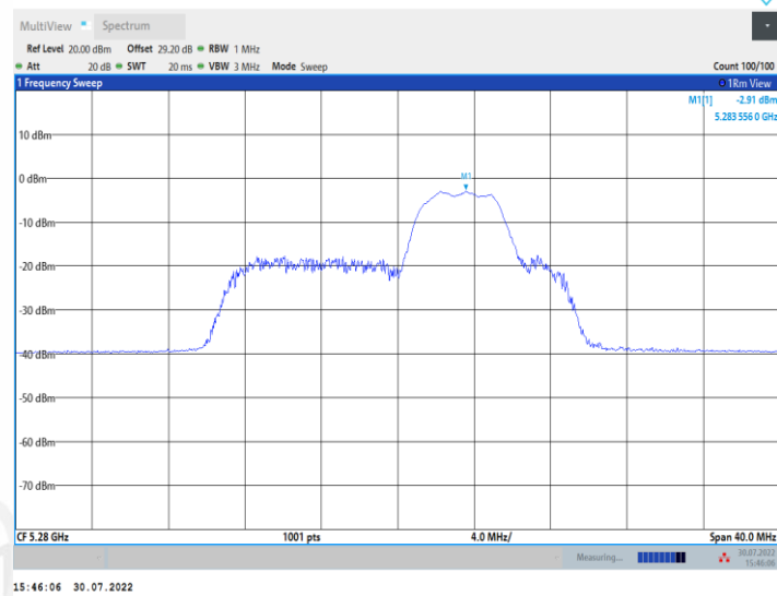
11AX20MIMO_Ant2_5280_52Tone_RU40
