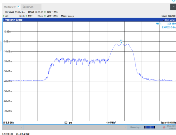
11AX20MIMO_Ant1_5500_106Tone_RU53
