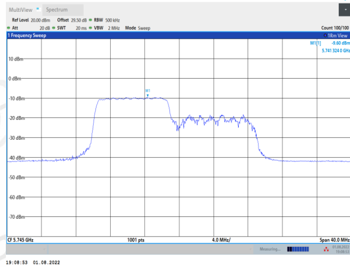
11AX20MIMO_Ant1_5745_106Tone_RU54
