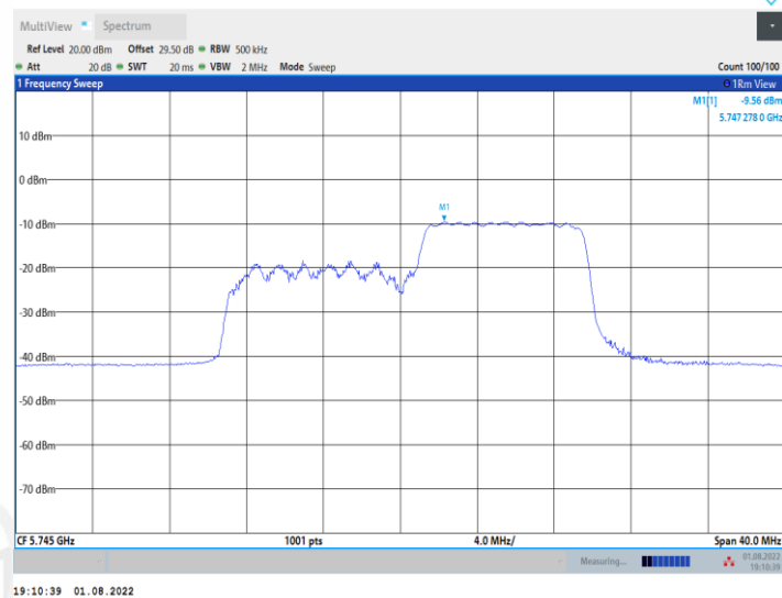
11AX20MIMO_Ant2_5745_26Tone_RU0
