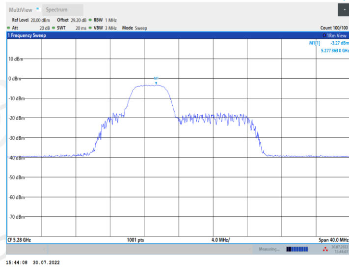
11AX20MIMO_Ant2_5280_52Tone_RU39
