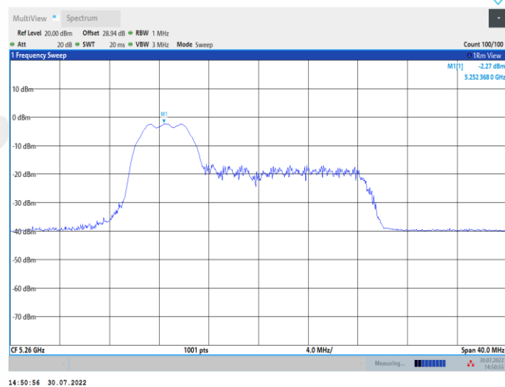
11AX20MIMO_Ant1_5260_52Tone_RU38
