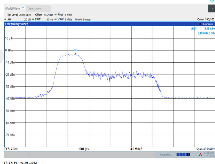
11AX20MIMO_Ant2_5500_52Tone_RU38
