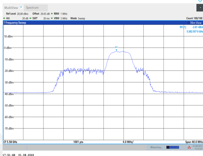
11AX20MIMO_Ant2_5580_52Tone_RU40
