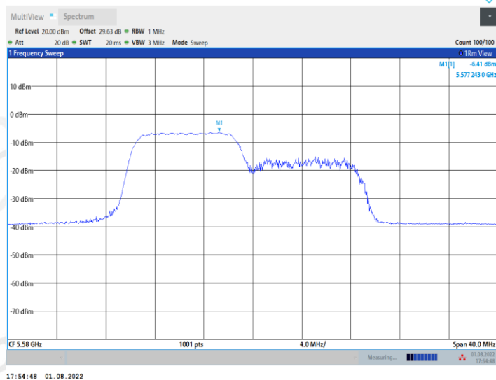
11AX20MIMO_Ant2_5580_106Tone_RU54
