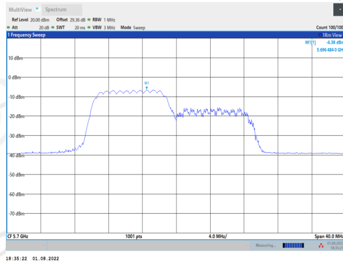
11AX20MIMO_Ant2_5700_106Tone_RU54
