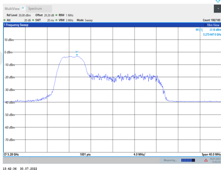
11AX20MIMO_Ant2_5280_52Tone_RU38
