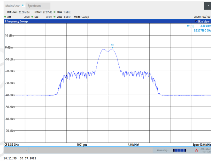
11AX20MIMO_Ant2_5320_26Tone_RU8
