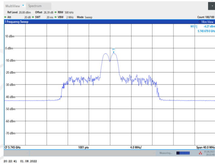
11AX20MIMO_Ant2_5745_26Tone_RU8
