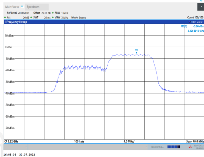
11AX20MIMO_Ant2_5320_26Tone_RU0
