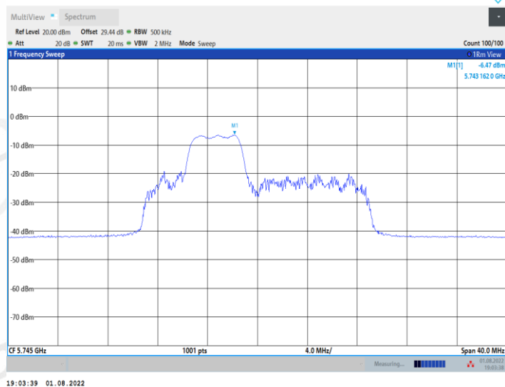
11AX20MIMO_Ant1_5745_52Tone_RU39
