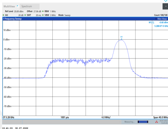
11AX20MIMO_Ant2_5280_52Tone_RU37
