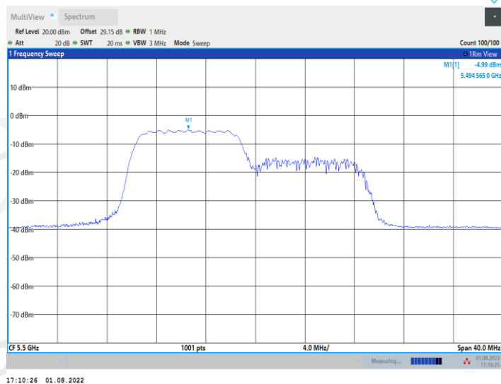
11AX20MIMO_Ant1_5500_106Tone_RU54
