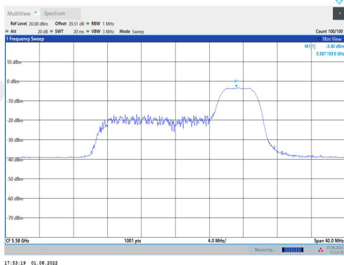
11AX20MIMO_Ant2_5580_106Tone_RU53
