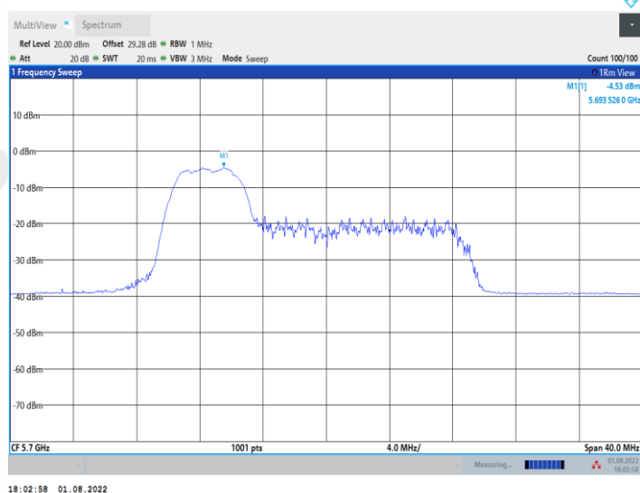
11AX20MIMO_Ant1_5700_52Tone_RU38
