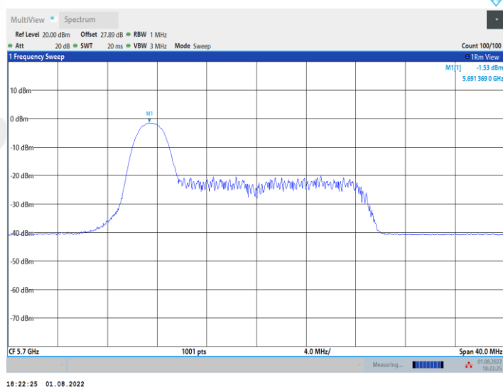
11AX20MIMO_Ant2_5700_26Tone_RU4
