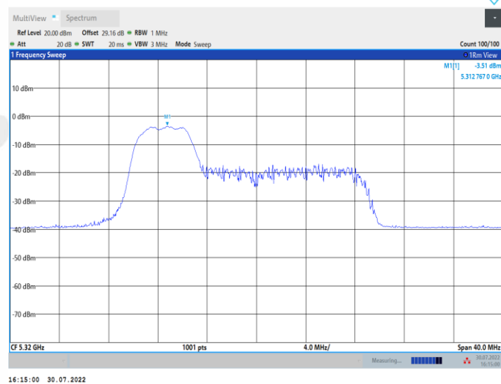
11AX20MIMO_Ant2_5320_52Tone_RU38
