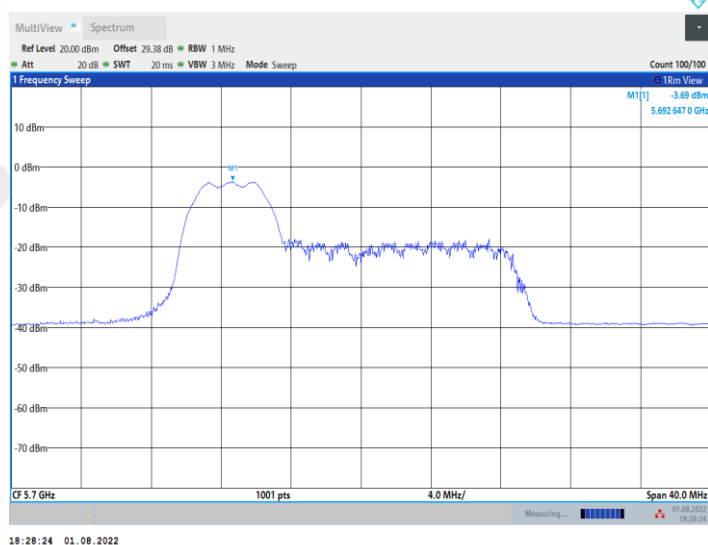
11AX20MIMO_Ant2_5700_52Tone_RU38
