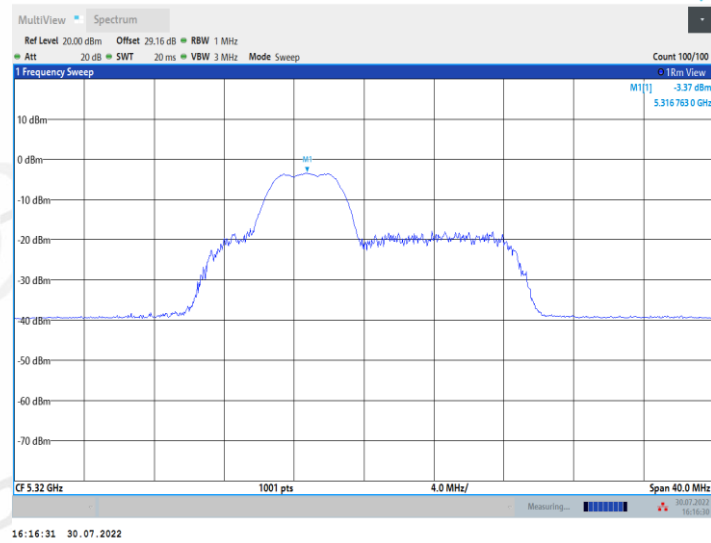
11AX20MIMO_Ant2_5320_52Tone_RU39
