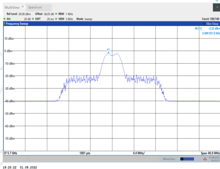
11AX20MIMO_Ant2_5700_26Tone_RU8
