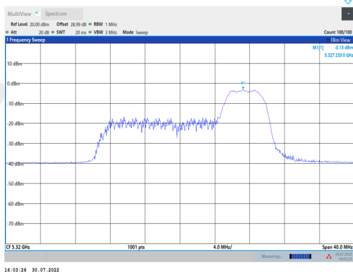
11AX20MIMO_Ant1_5320_106Tone_RU53
