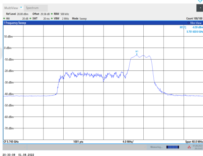
11AX20MIMO_Ant2_5745_106Tone_RU53
