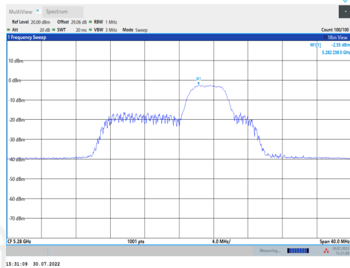
11AX20MIMO_Ant1_5280_52Tone_RU40
