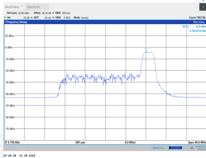
11AX20MIMO_Ant2_5745_52Tone_RU37
