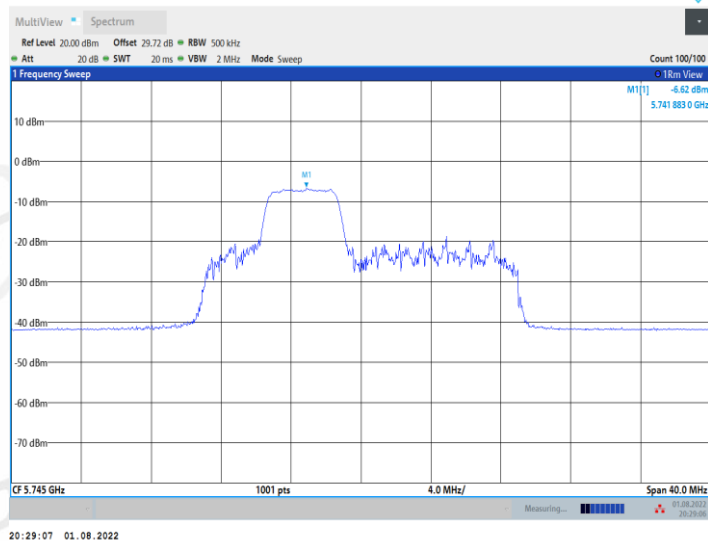
11AX20MIMO_Ant2_5745_52Tone_RU39
