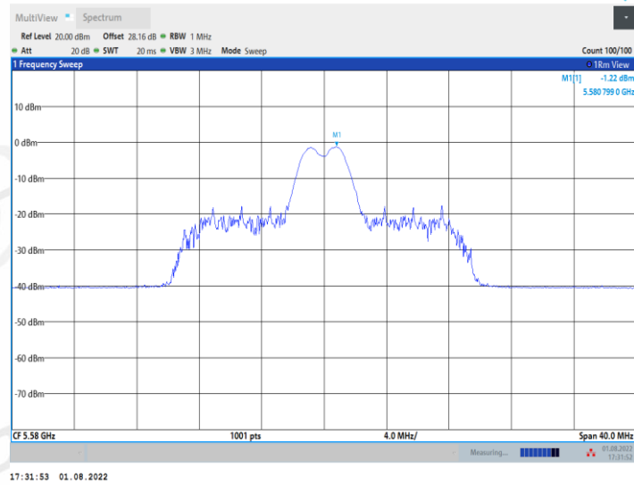
11AX20MIMO_Ant1_5580_26Tone_RU8
