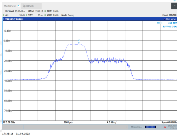
11AX20MIMO_Ant1_5580_52Tone_RU39
