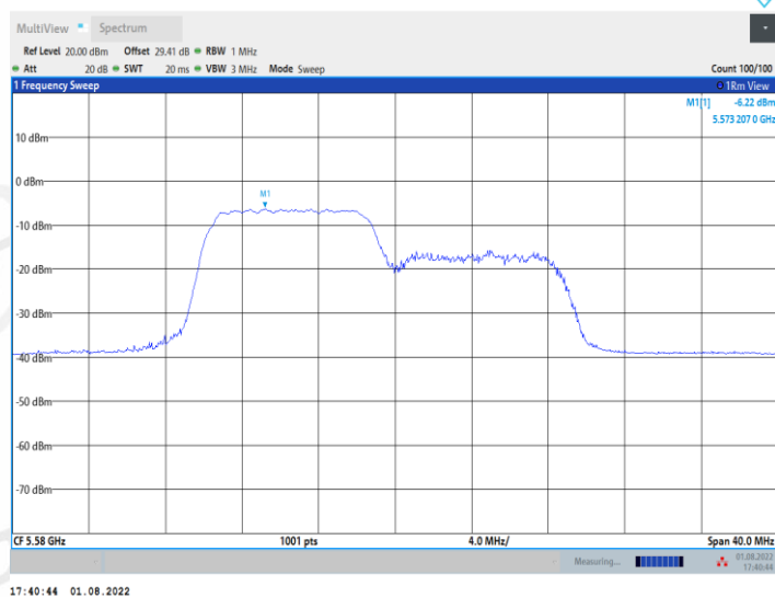
11AX20MIMO_Ant1_5580_106Tone_RU54
