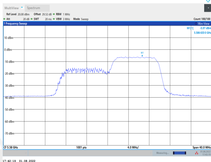
11AX20MIMO_Ant2_5580_26Tone_RU0
