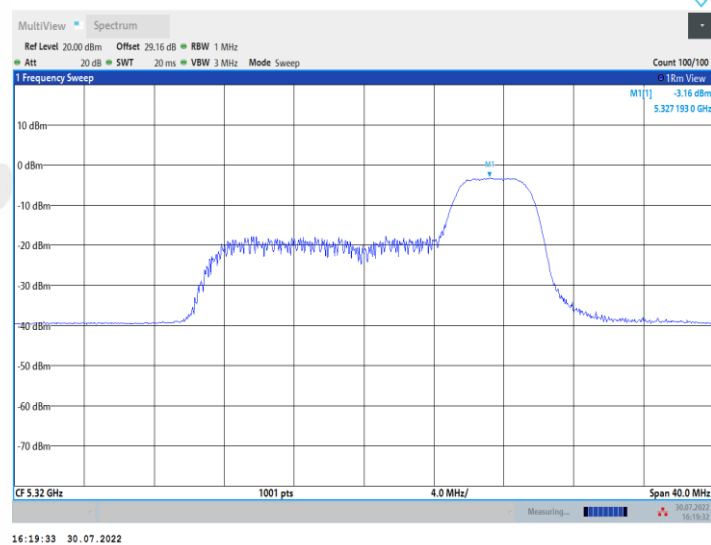
11AX20MIMO_Ant2_5320_106Tone_RU53
