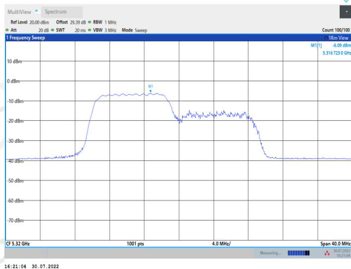
11AX20MIMO_Ant2_5320_106Tone_RU54
