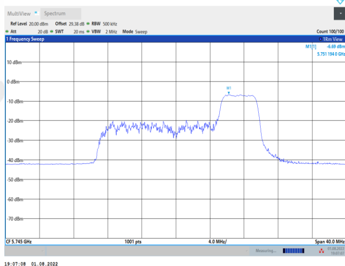
11AX20MIMO_Ant1_5745_106Tone_RU53
