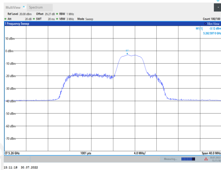
11AX20MIMO_Ant2_5260_52Tone_RU40
