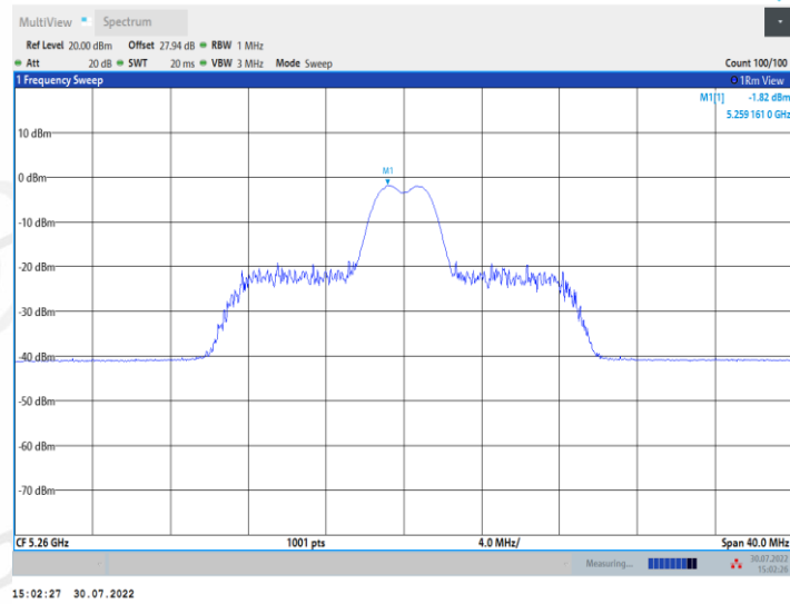
11AX20MIMO_Ant2_5260_26Tone_RU8
