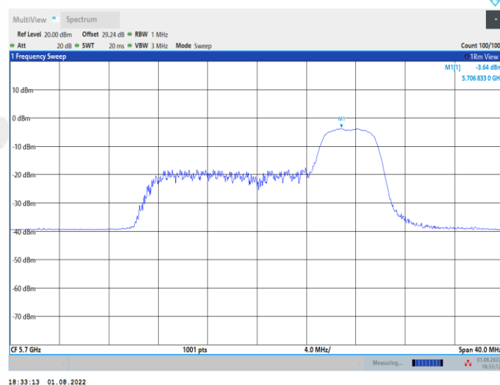
11AX20MIMO_Ant2_5700_106Tone_RU53
