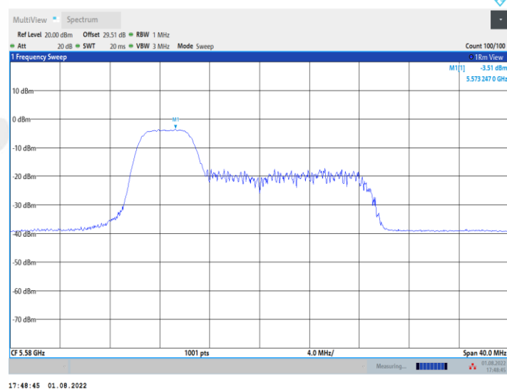
11AX20MIMO_Ant2_5580_52Tone_RU38
