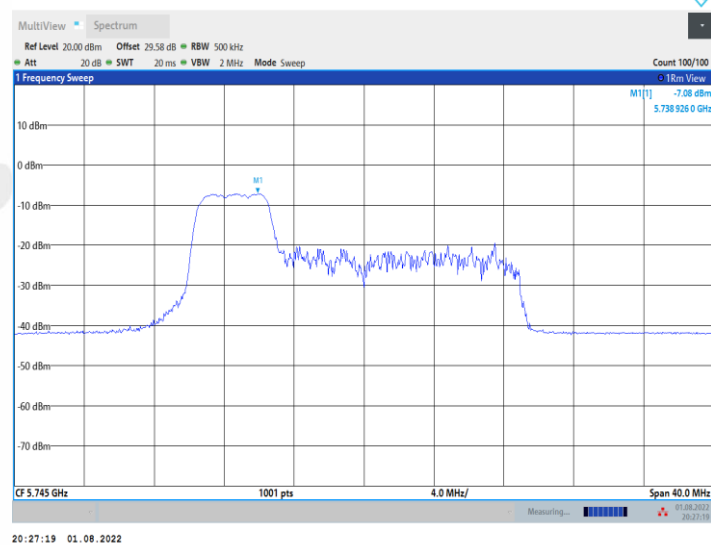
11AX20MIMO_Ant2_5745_52Tone_RU38
