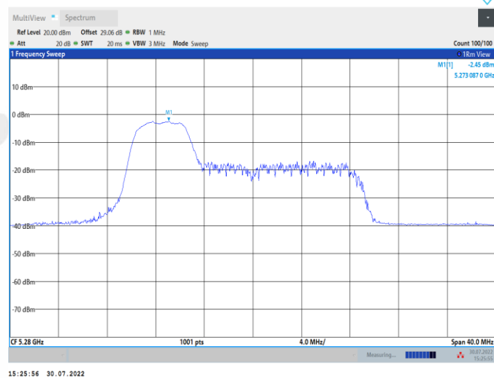
11AX20MIMO_Ant1_5280_52Tone_RU38
