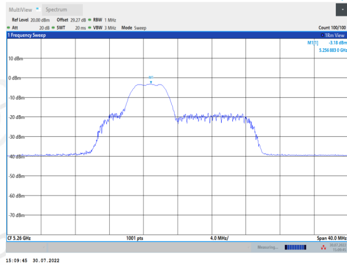
11AX20MIMO_Ant2_5260_52Tone_RU39
