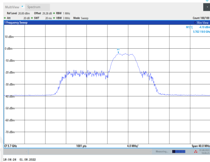
11AX20MIMO_Ant1_5700_52Tone_RU40
