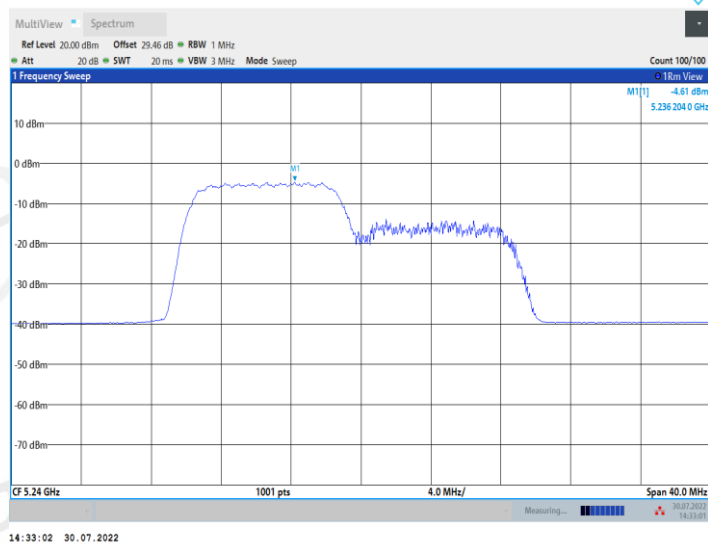
11AX20MIMO_Ant2_5240_106Tone_RU54
