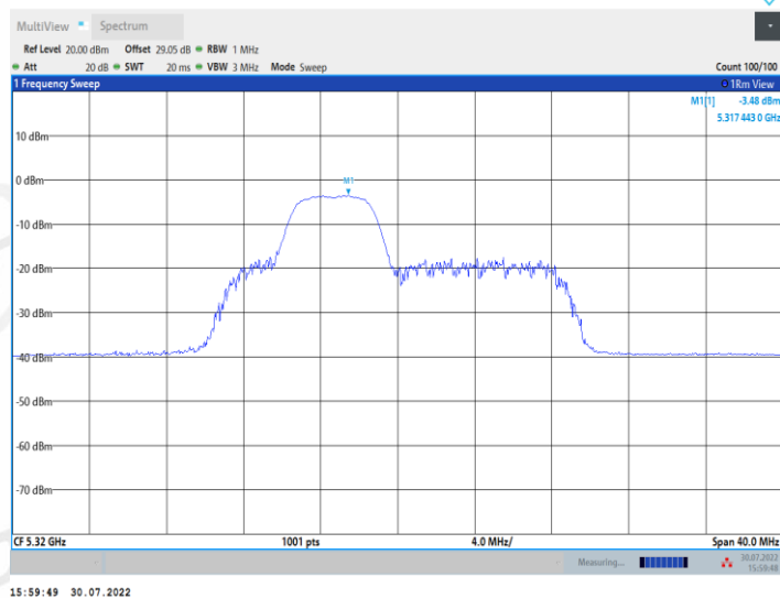
11AX20MIMO_Ant1_5320_52Tone_RU39
