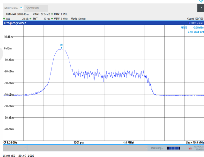
11AX20MIMO_Ant2_5260_26Tone_RU4
