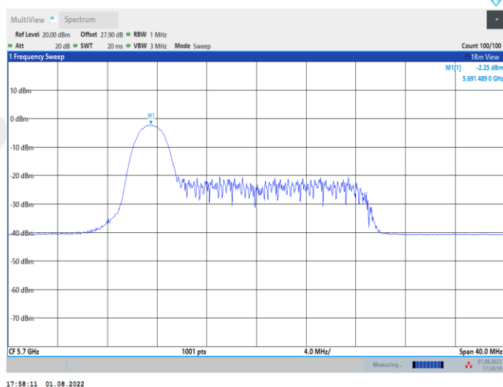
11AX20MIMO_Ant1_5700_26Tone_RU4
