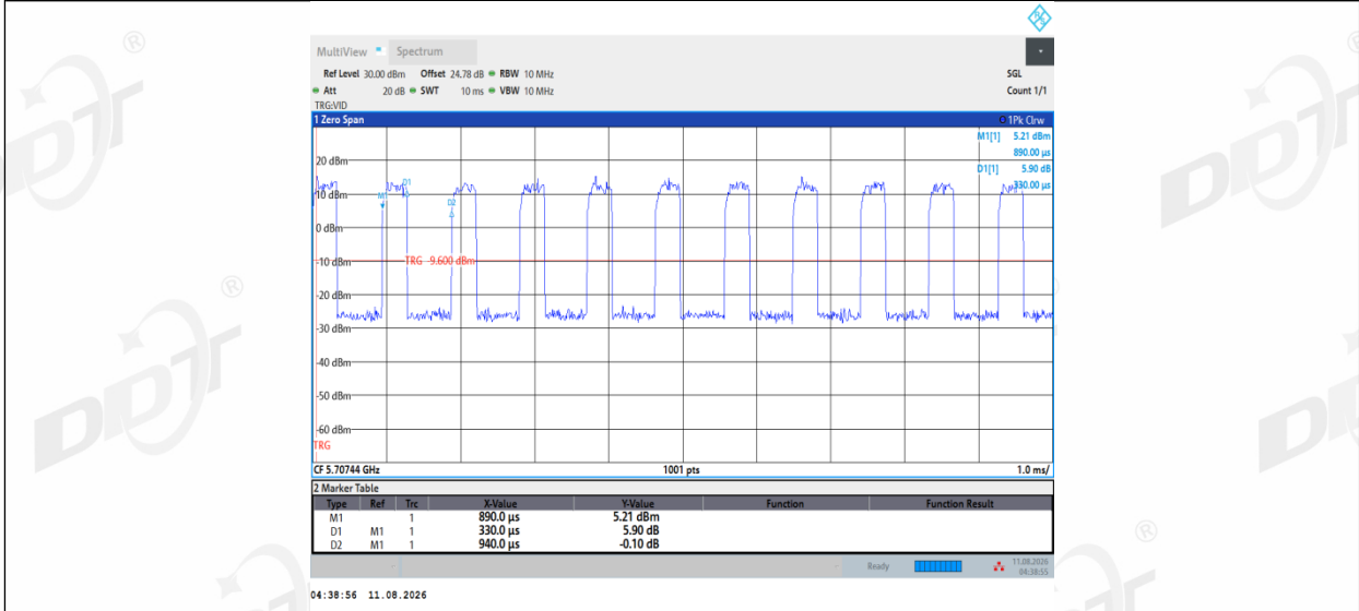
11AX20MIMO_Ant2_5700_106Tone_RU54
