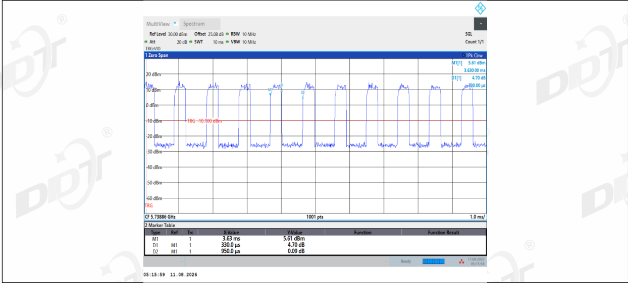
11AX20MIMO_Ant1_5745_106Tone_RU53
