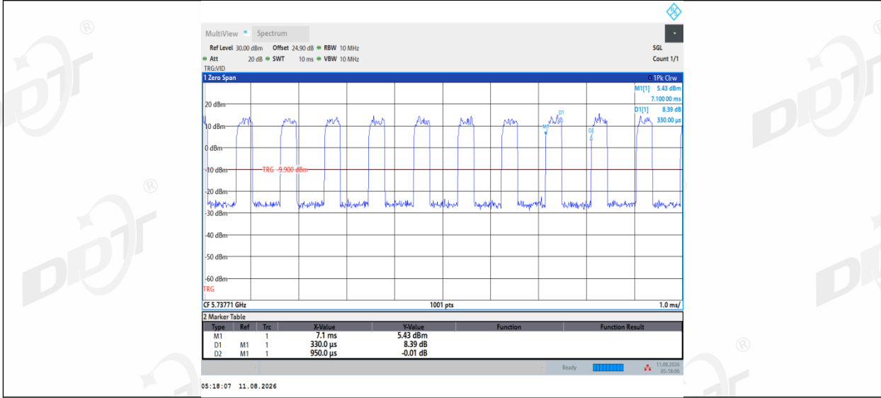
11AX20MIMO_Ant2_5745_106Tone_RU53
