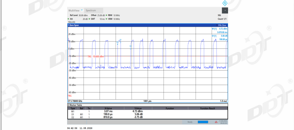
11AX20MIMO_Ant2_5700_26Tone_RU8
