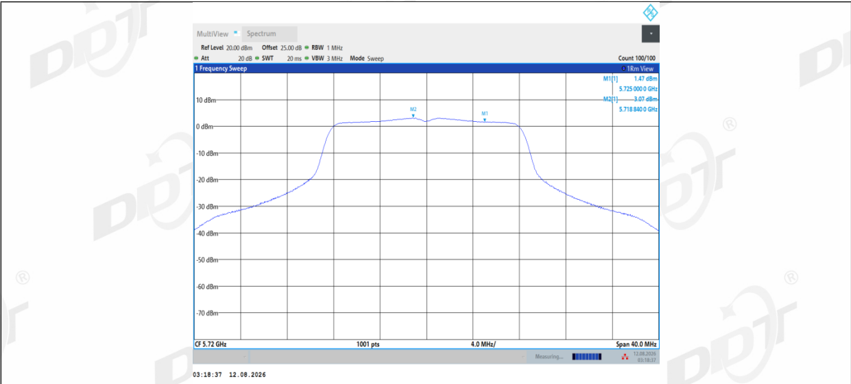
11A_Ant2_5720_UNII-2C
