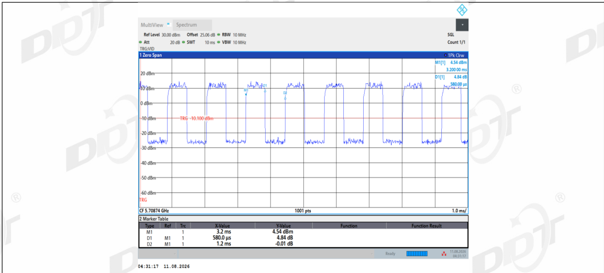
11AX20MIMO_Ant1_5700_52Tone_RU40
