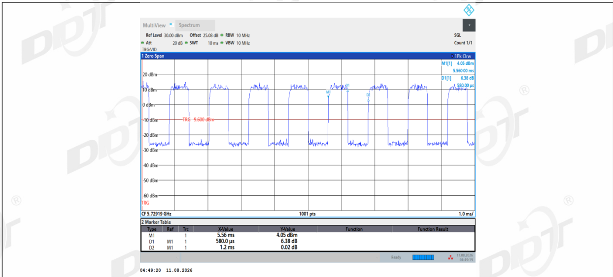
11AX20MIMO_Ant1_5720_52Tone_RU40
