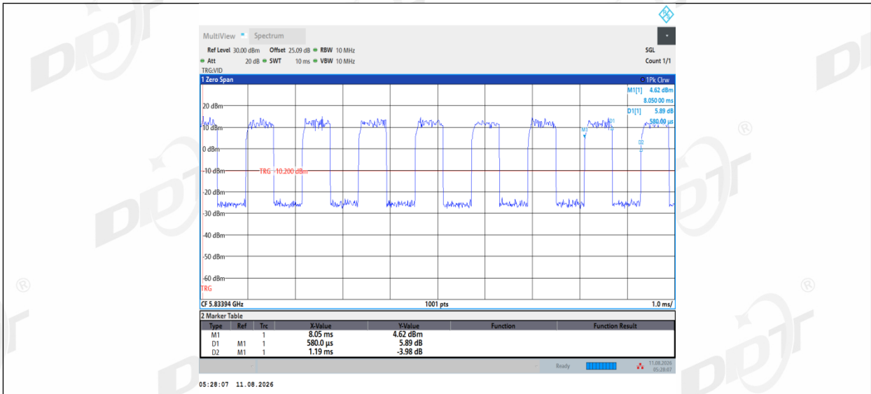
11AX20MIMO_Ant1_5825_52Tone_RU40
