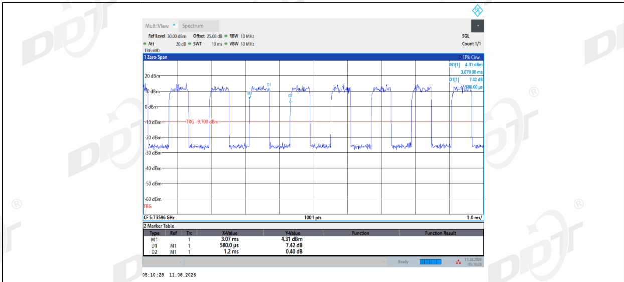
11AX20MIMO_Ant1_5745_52Tone_RU37
