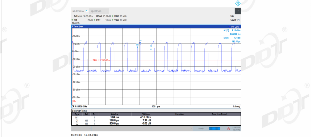
11AX20MIMO_Ant2_5825_26Tone_RU8
