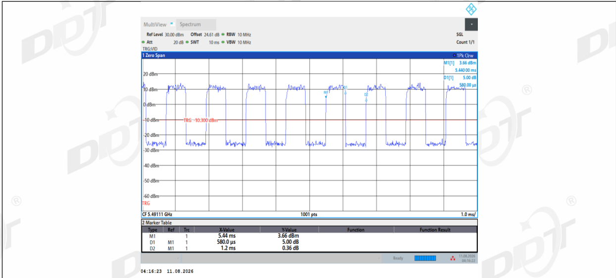
11AX20MIMO_Ant2_5500_52Tone_RU37
