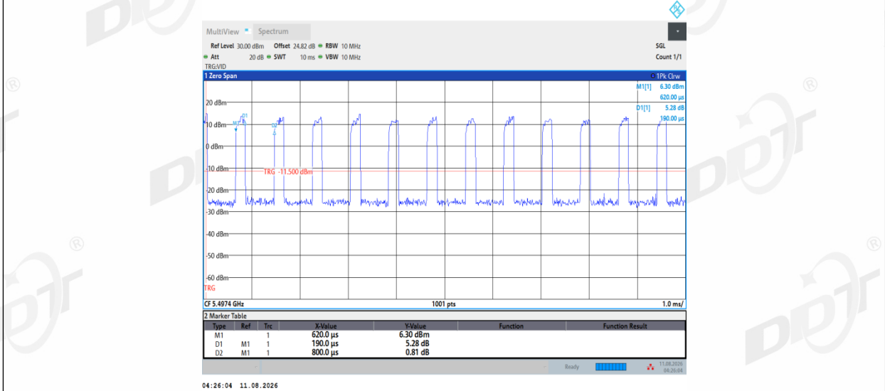
11AX20MIMO_Ant2_5500_26Tone_RU0
