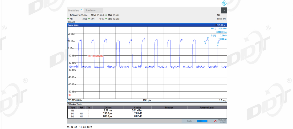
11AX20MIMO_Ant2_5720_26Tone_RU8
