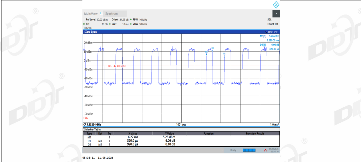
11AX20MIMO_Ant2_5825_106Tone_RU54
