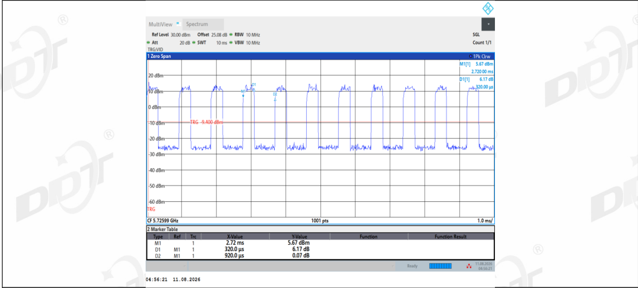
11AX20MIMO_Ant1_5720_106Tone_RU54
