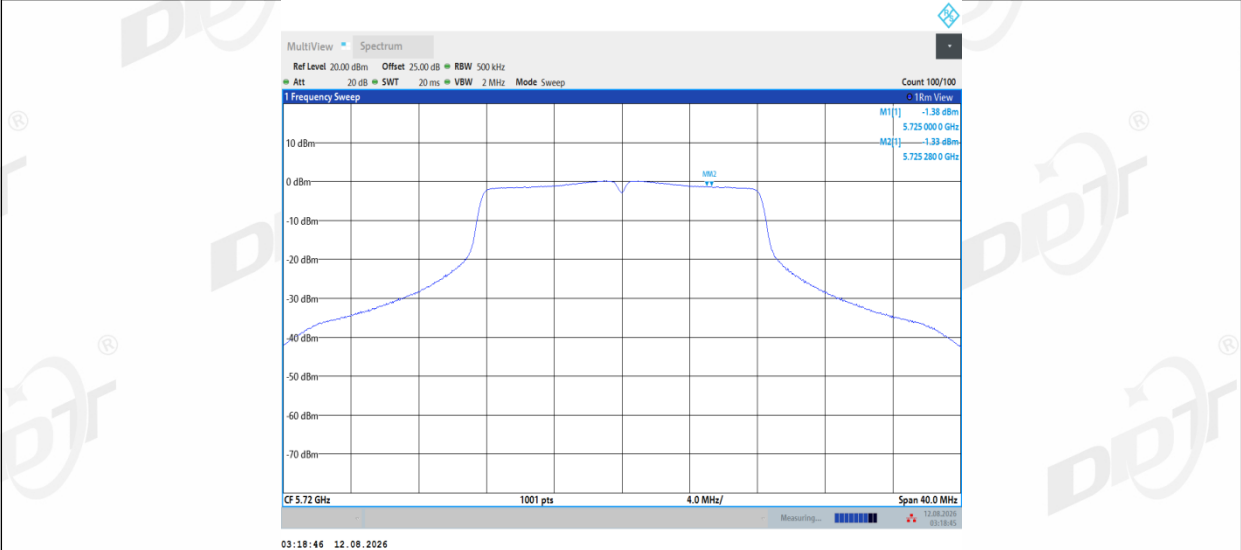
11A_Ant2_5720_UNII-3
