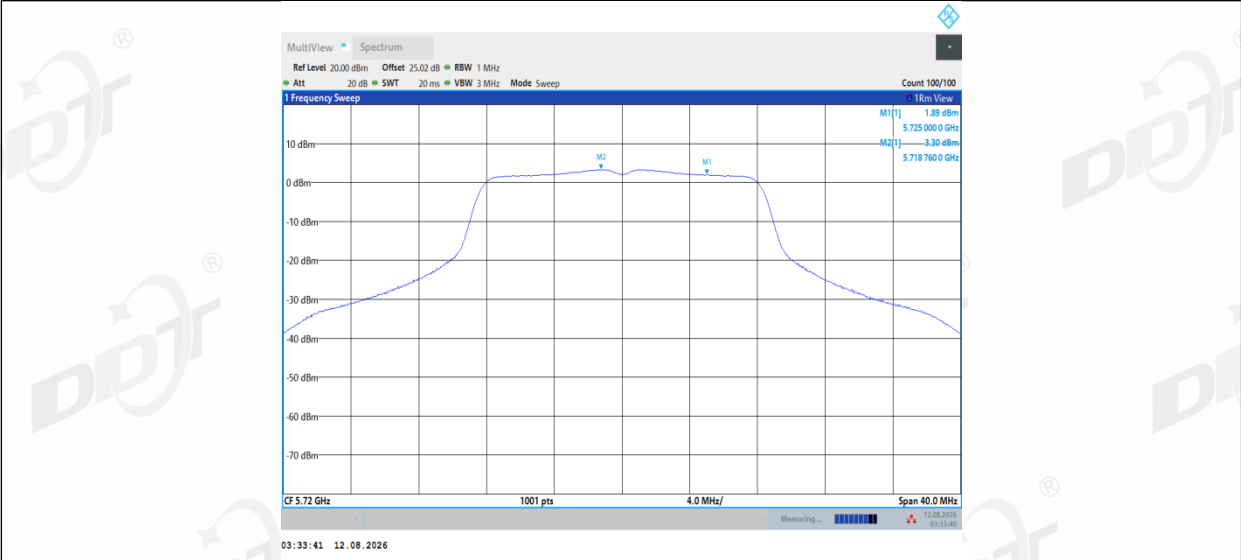
11A_Ant1_5720_UNII-3
