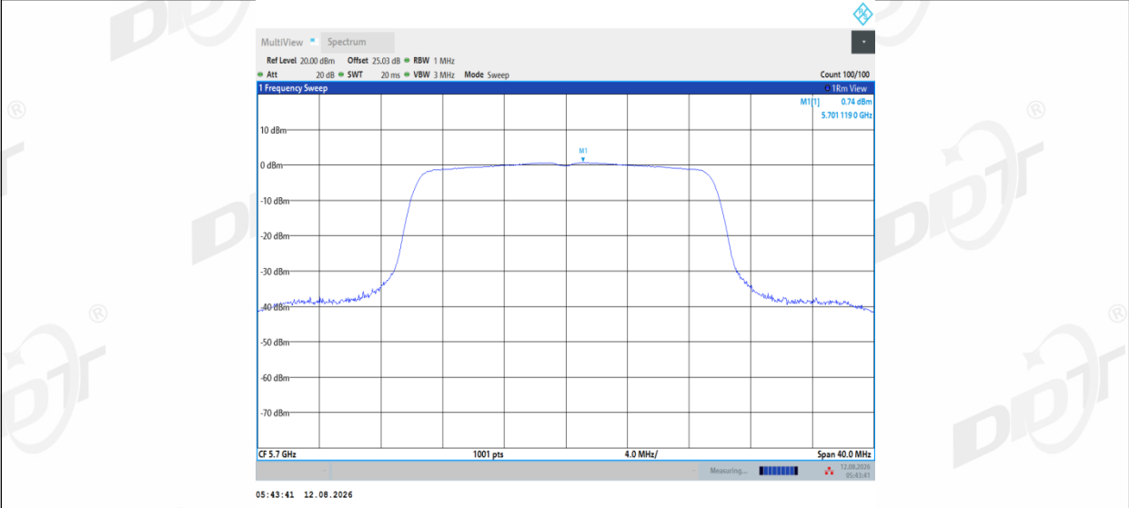
11AX20MIMO_Ant2_5700
