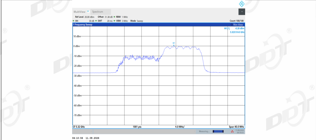
11AX20MIMO_Ant2_5320_26Tone_RU8
