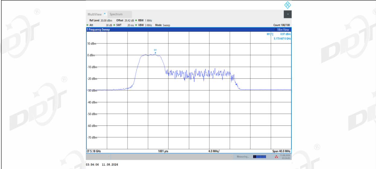
11AX20MIMO_Ant2_5180_106Tone_RU53
