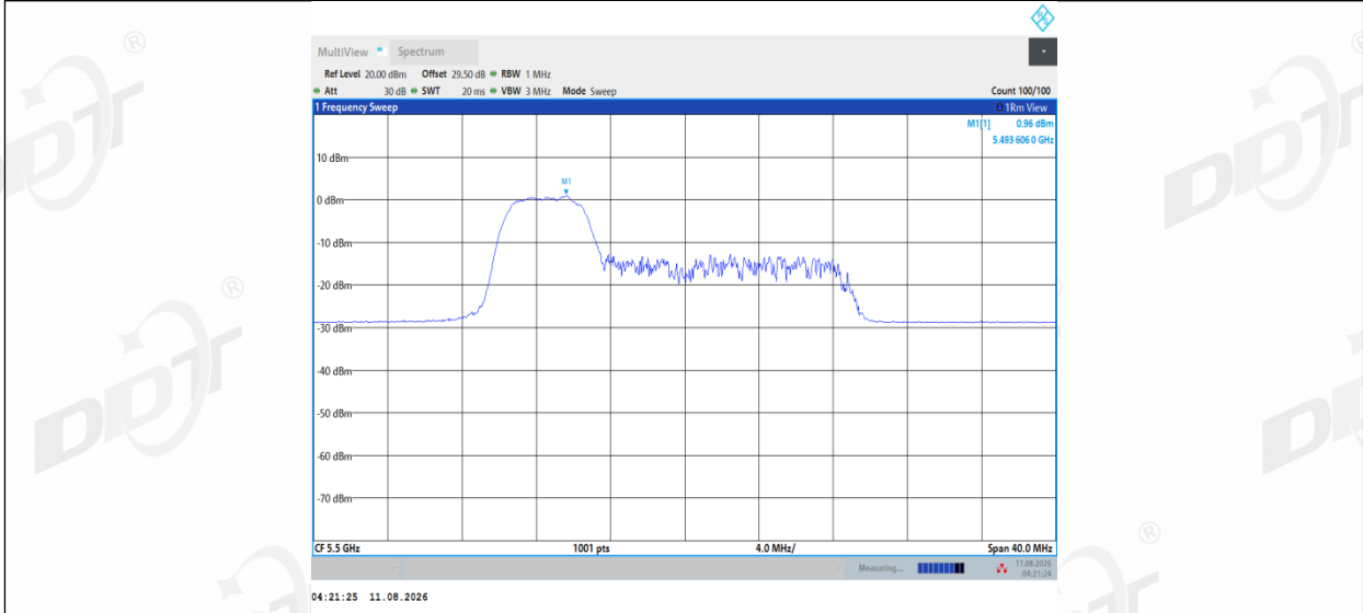
11AX20MIMO_Ant1_5500_106Tone_RU53
