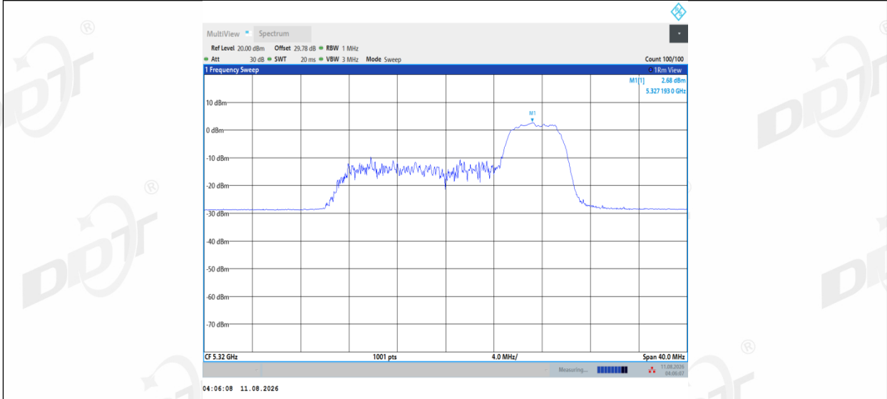
11AX20MIMO_Ant1_5320_106Tone_RU54
