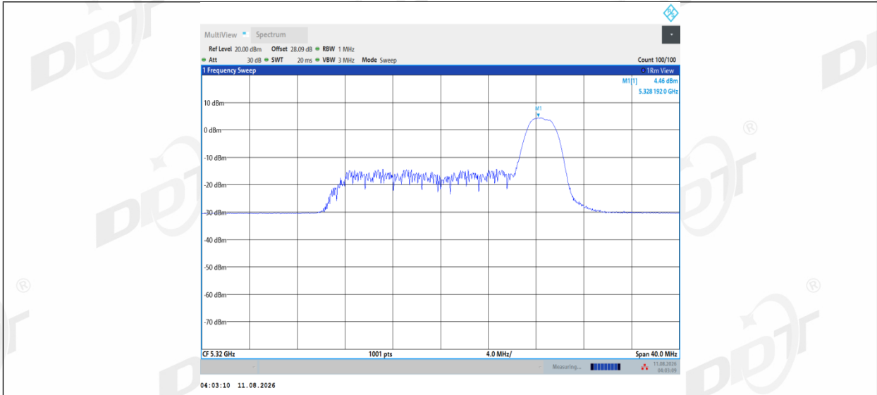
11AX20MIMO_Ant2_5320_52Tone_RU40
