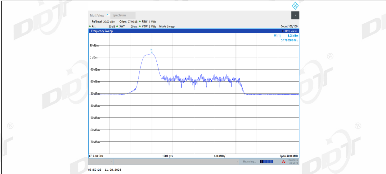
11AX20MIMO_Ant2_5180_52Tone_RU37
