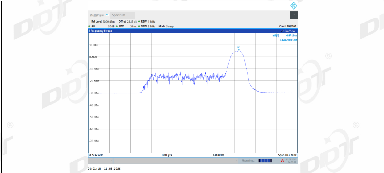
11AX20MIMO_Ant1_5320_52Tone_RU40
