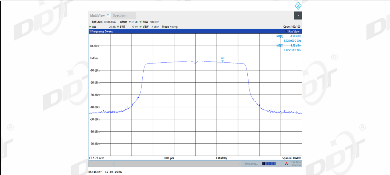
11AX20MIMO_Ant2_5720_UNII-3
