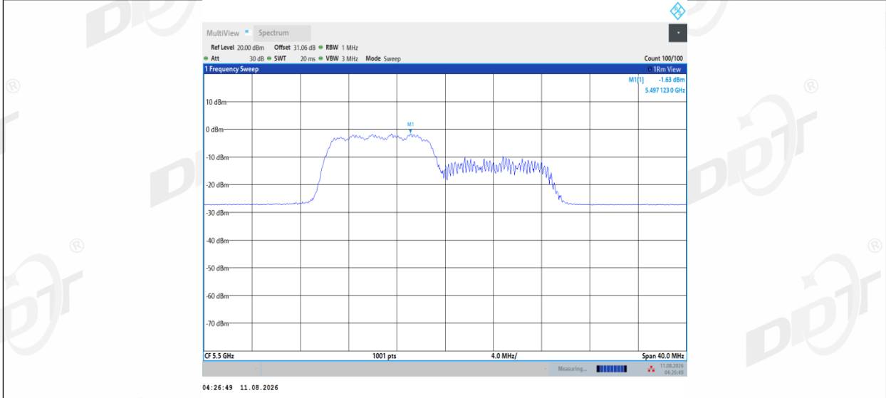
11AX20MIMO_Ant2_5500_26Tone_RU0
