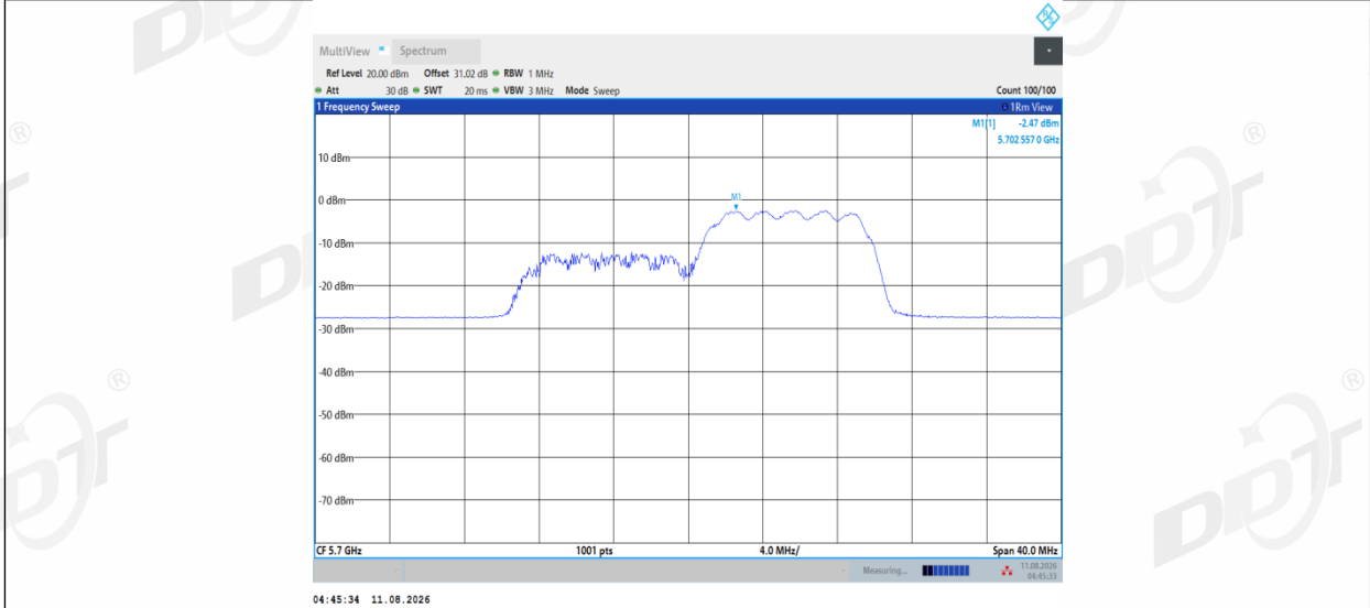
11AX20MIMO_Ant1_5720_UNII-2C_26Tone_RU8
