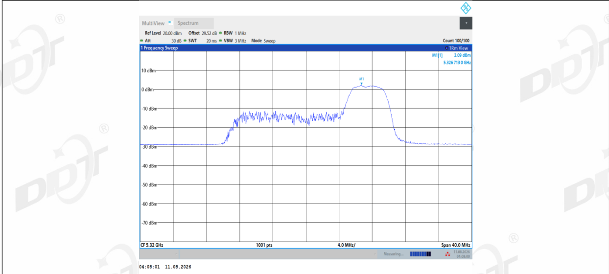
11AX20MIMO_Ant2_5320_106Tone_RU54
