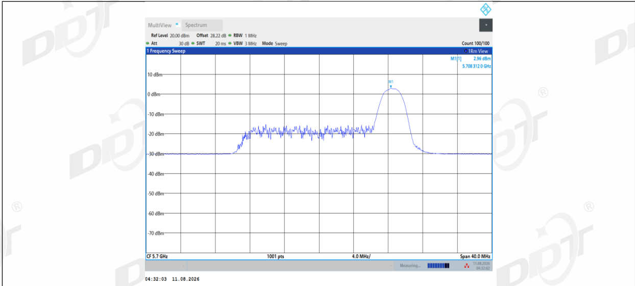
11AX20MIMO_Ant1_5700_52Tone_RU40
