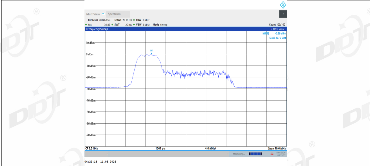
11AX20MIMO_Ant2_5500_106Tone_RU53
