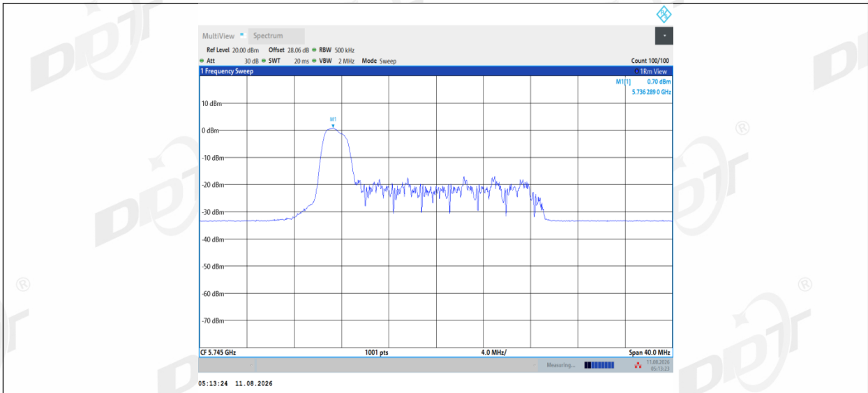
11AX20MIMO_Ant2_5745_52Tone_RU37
