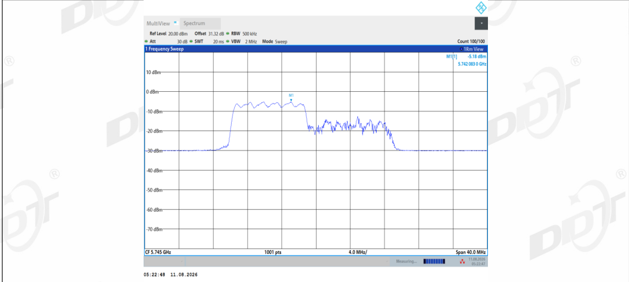
11AX20MIMO_Ant2_5745_26Tone_RU0
