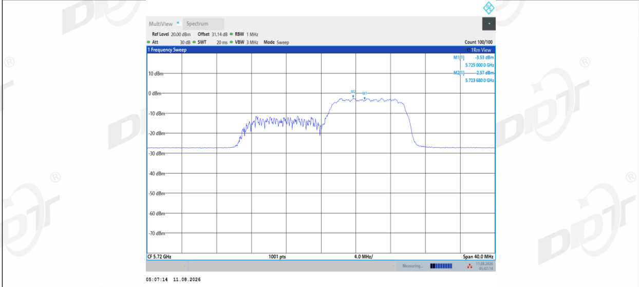
11AX20MIMO_Ant1_5720_UNII-3_26Tone_RU8
