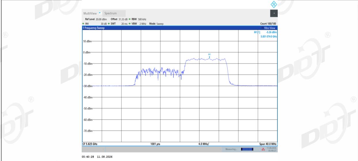
11AX20MIMO_Ant2_5825_26Tone_RU8
