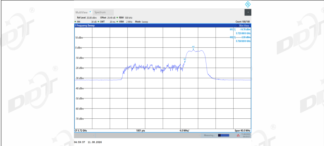
11AX20MIMO_Ant2_5720_UNII-3_106Tone_RU54
