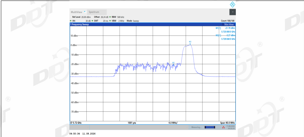
11AX20MIMO_Ant1_5720_UNII-3_52Tone_RU40
