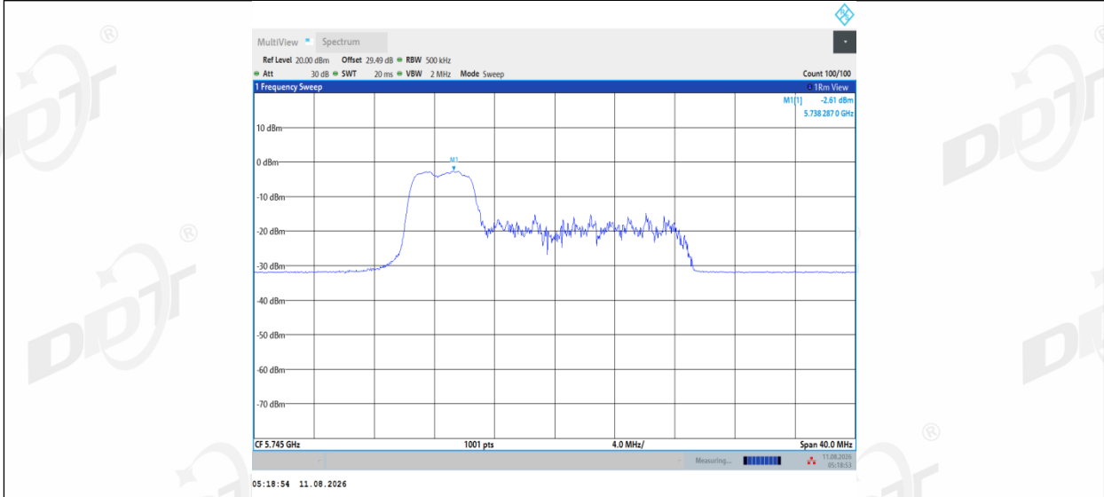
11AX20MIMO_Ant2_5745_106Tone_RU53
