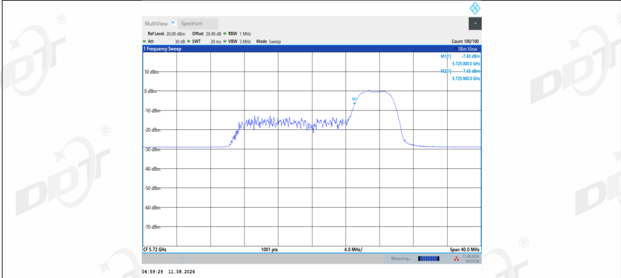
11AX20MIMO_Ant2_5720_UNII-2C_106Tone_RU54
