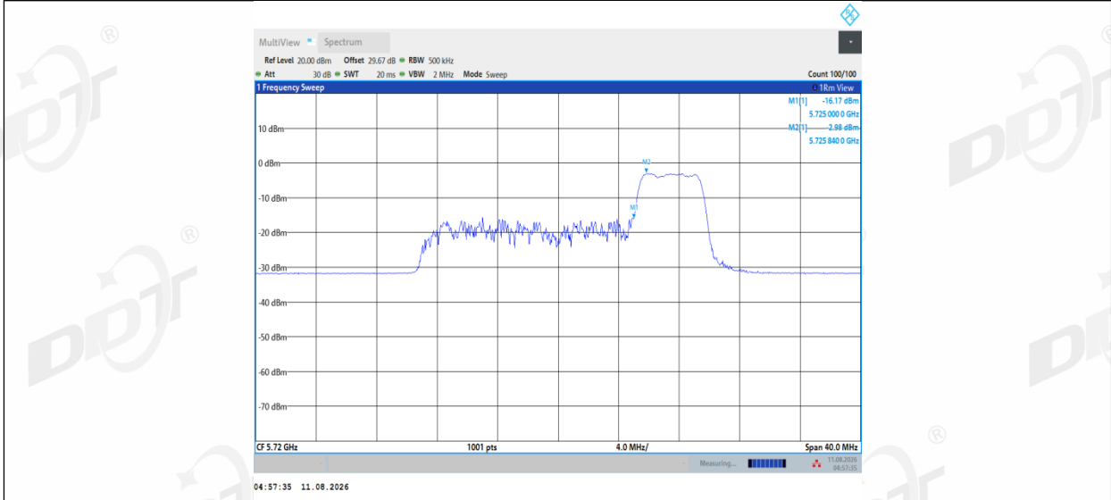
11AX20MIMO_Ant1_5720_UNII-3_106Tone_RU54
