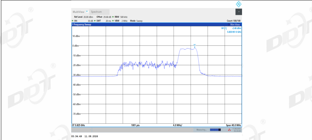
11AX20MIMO_Ant1_5825_106Tone_RU54
