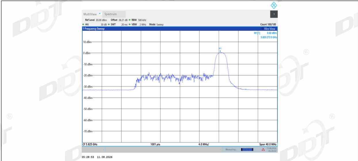
11AX20MIMO_Ant1_5825_52Tone_RU40
