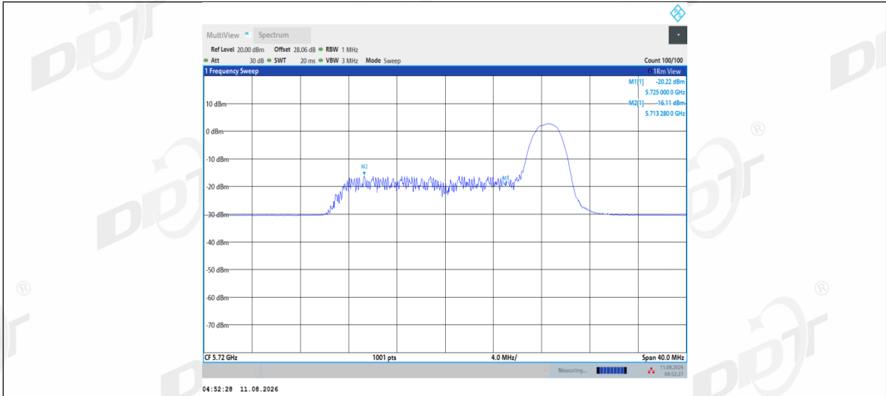
11AX20MIMO_Ant2_5720_UNII-2C_52Tone_RU40
