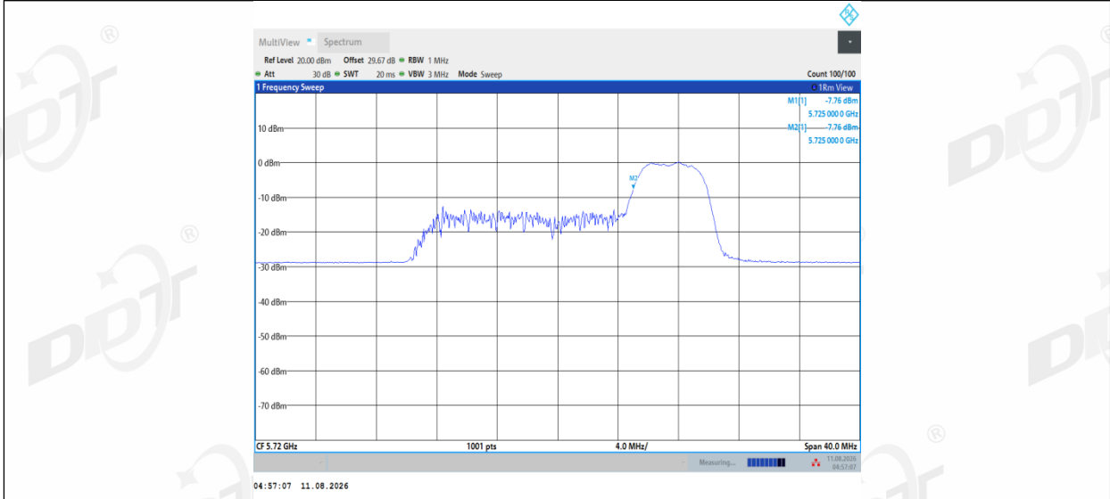
11AX20MIMO_Ant1_5720_UNII-2C_106Tone_RU54
