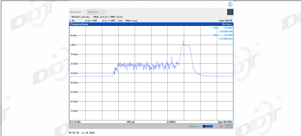
11AX20MIMO_Ant2_5720_UNII-3_52Tone_RU40
