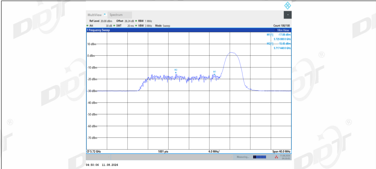
11AX20MIMO_Ant1_5720_UNII-2C_52Tone_RU40
