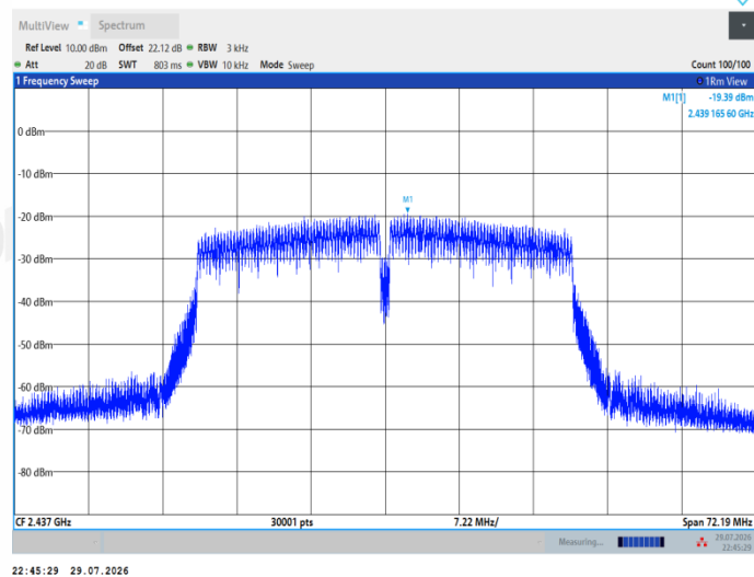
11N40MIMO_Ant2_2437
