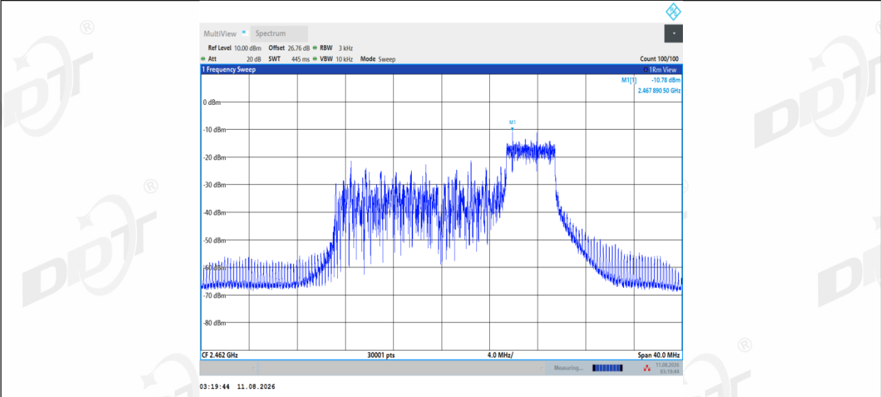
11AX20MIMO_Ant1_2462_106Tone_RU54
