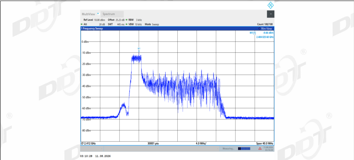
11AX20MIMO_Ant2_2412_52Tone_RU37
