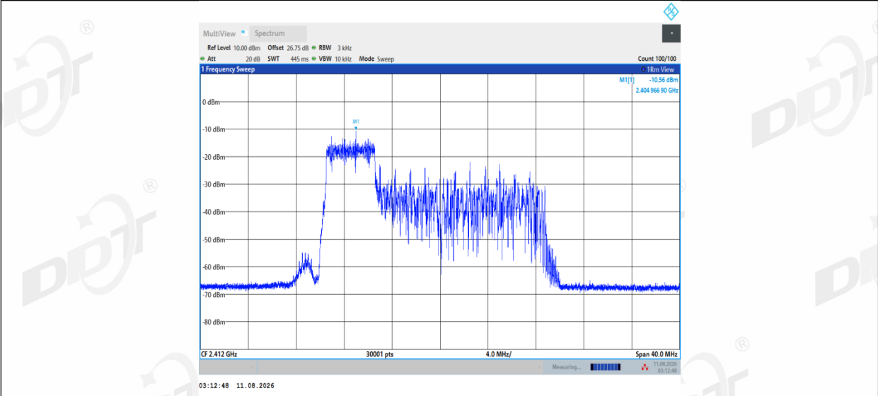
11AX20MIMO_Ant2_2412_106Tone_RU53
