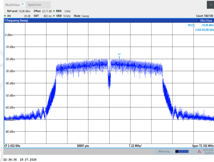
11N40MIMO_Ant2_2422
