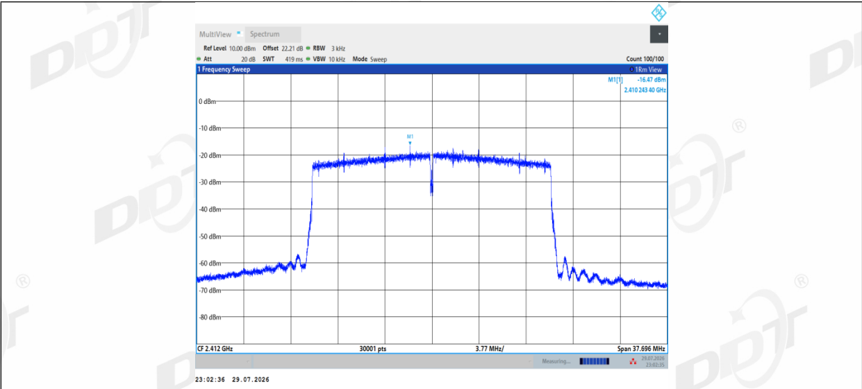
11AX20MIMO_Ant2_2412
