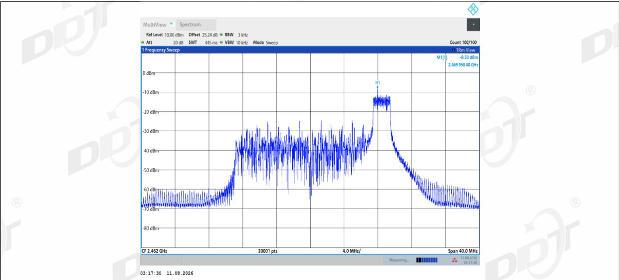
11AX20MIMO_Ant1_2462_52Tone_RU40
