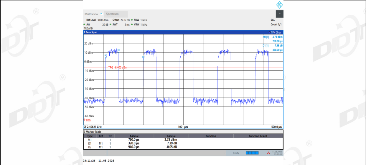
11AX20MIMO_Ant2_2412_106Tone_RU53
