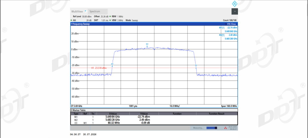
11AC80MIMO_Ant2_5690
