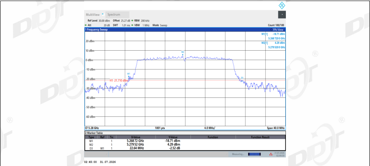
11AX20MIMO_Ant2_5280
