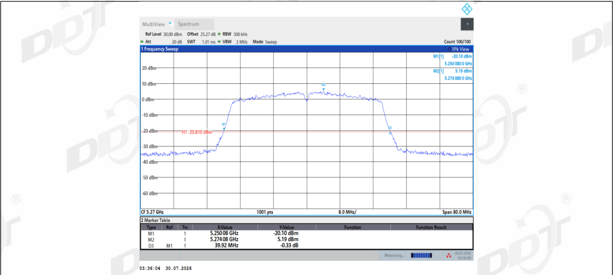
11AC40MIMO_Ant2_5270
