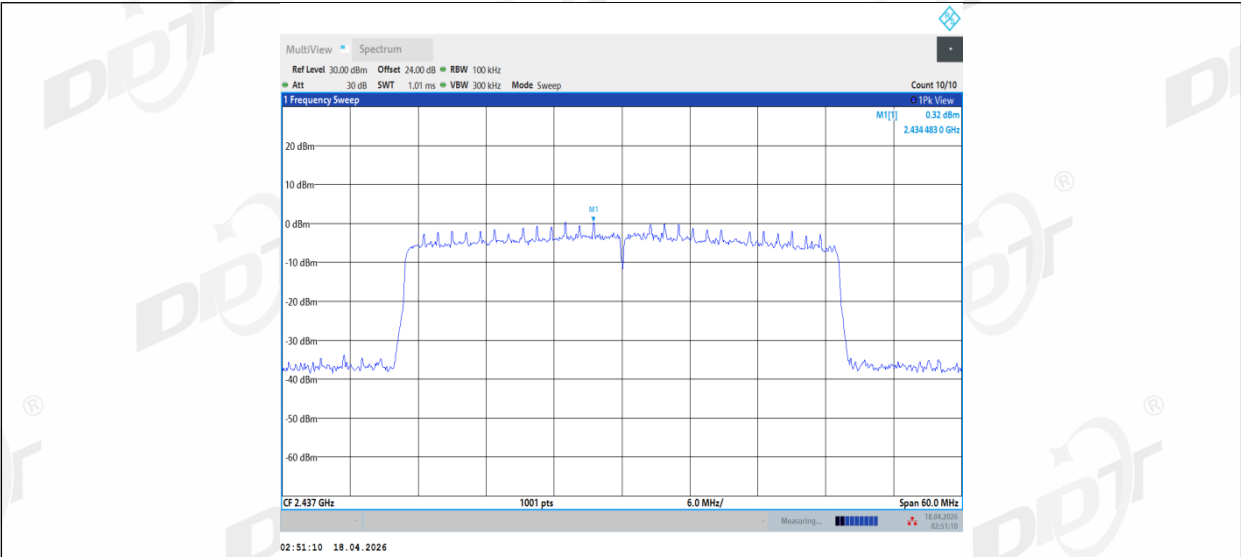
11AX40MIMO_Ant2_2437_30-1000
