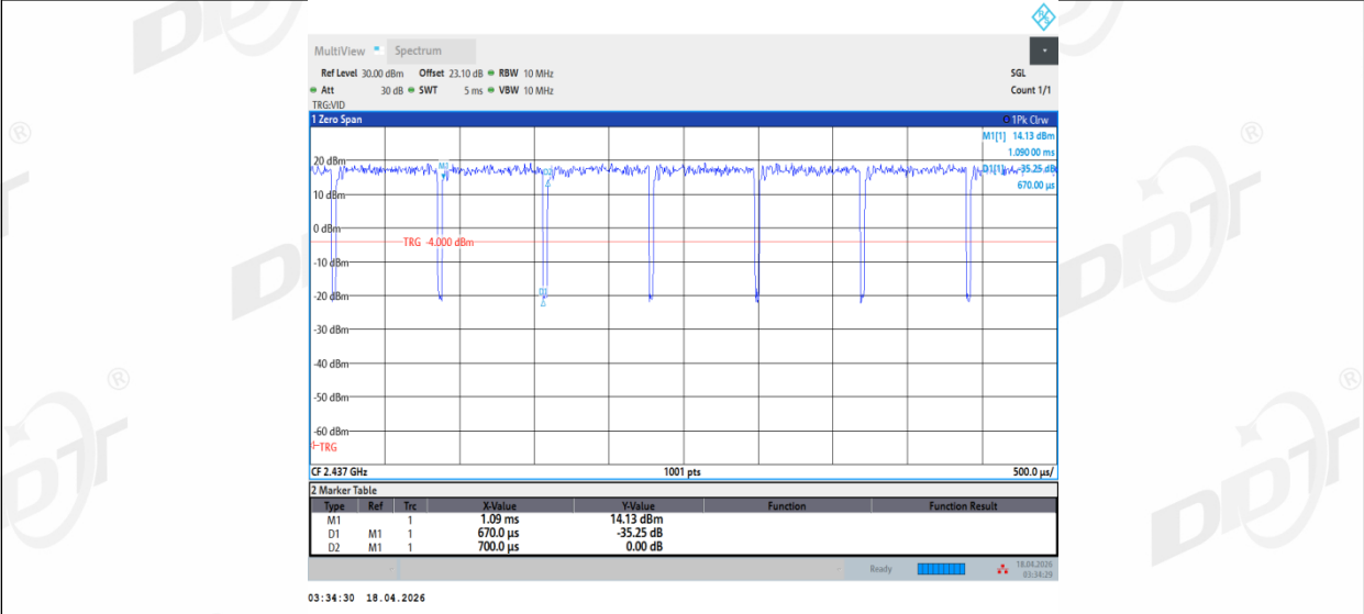
11N20MIMO_Ant2_2437
