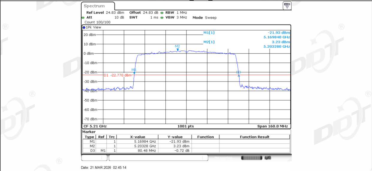
11AC80MIMO_Ant2_5210
