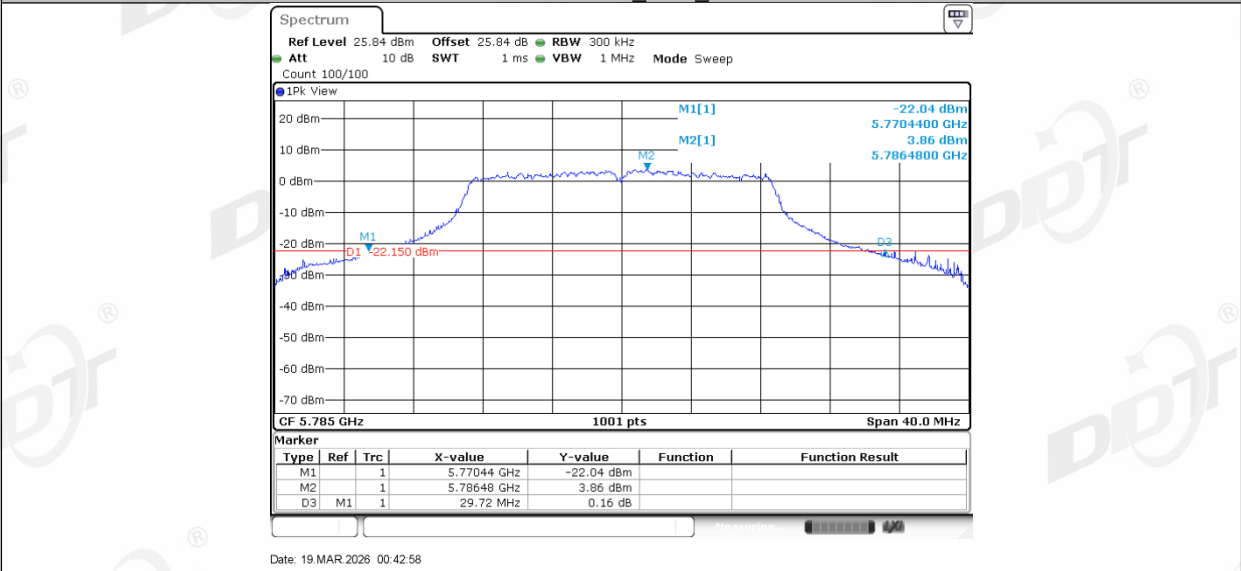
11AC20MIMO_Ant2_5785
