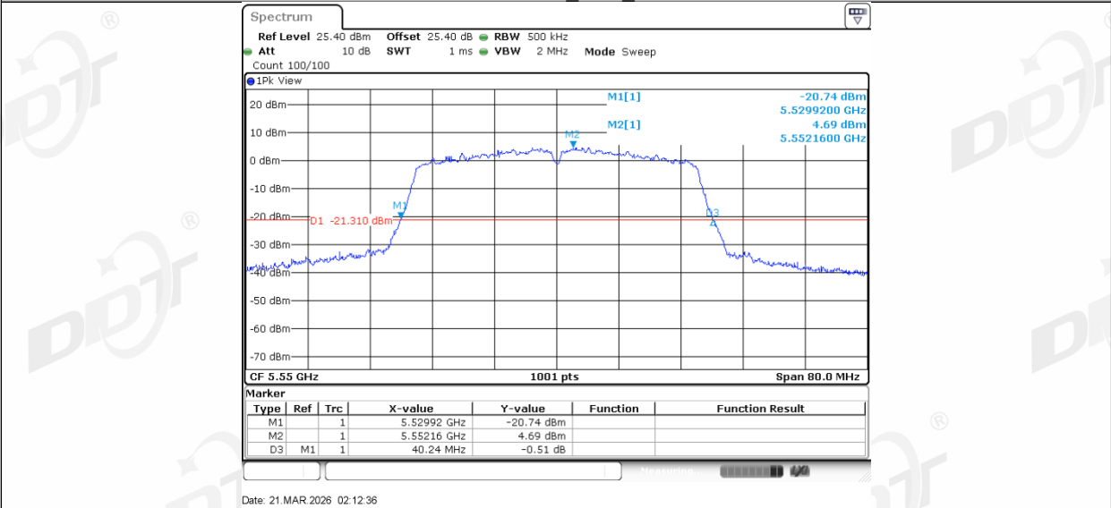
11AC40MIMO_Ant2_5550
