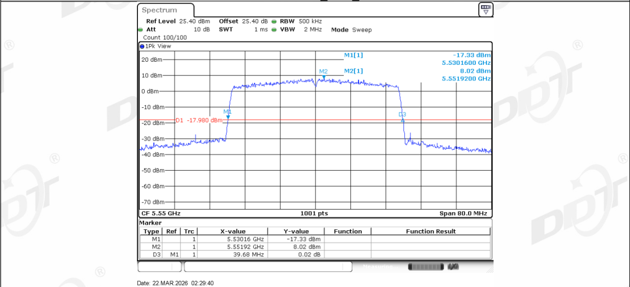
11AX40MIMO_Ant2_5550
