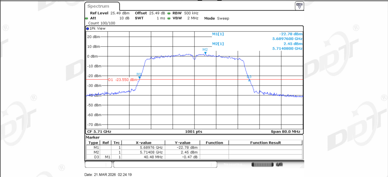
11AC40MIMO_Ant2_5710
