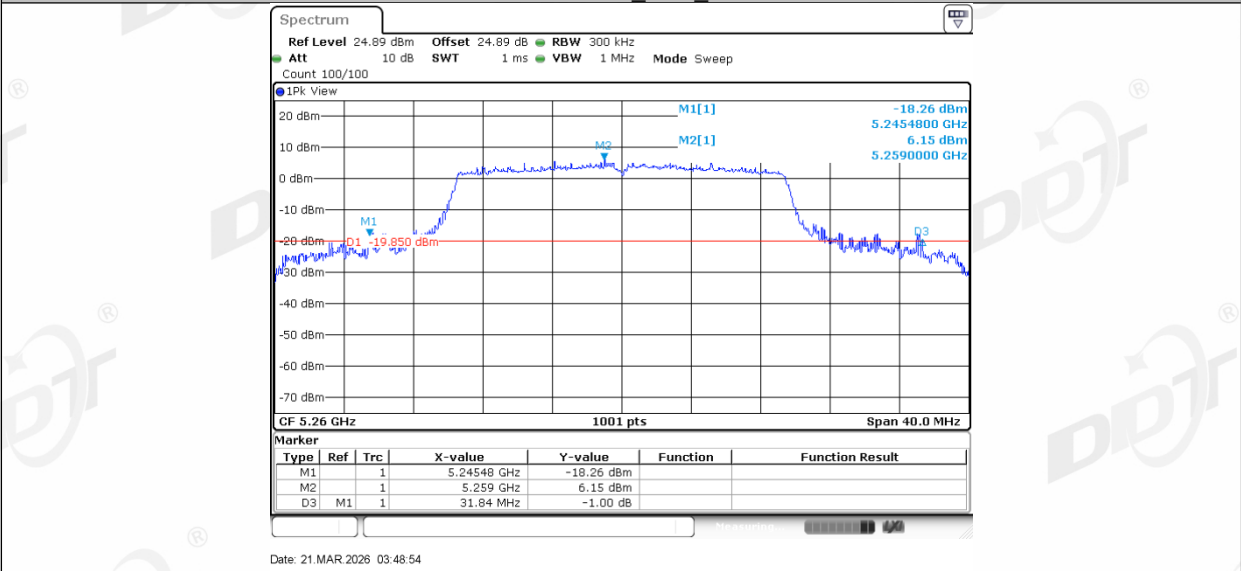
11AX20MIMO_Ant2_5260
