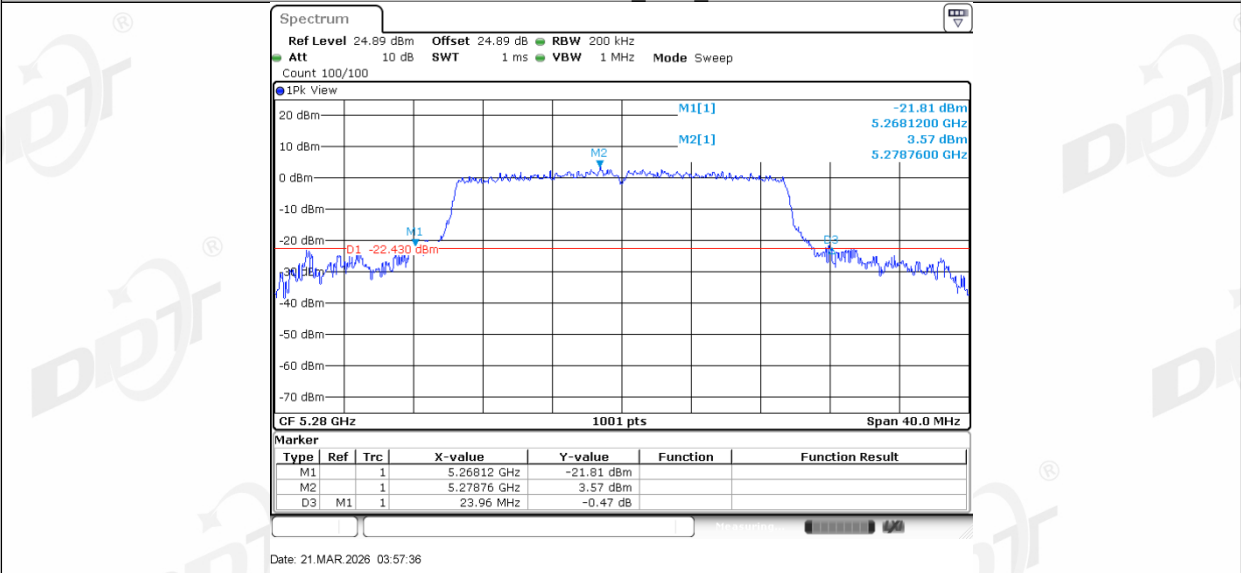
11AX20MIMO_Ant2_5280
