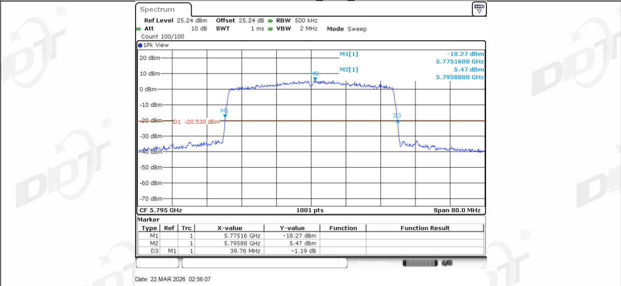
11AX40MIMO_Ant2_5795
