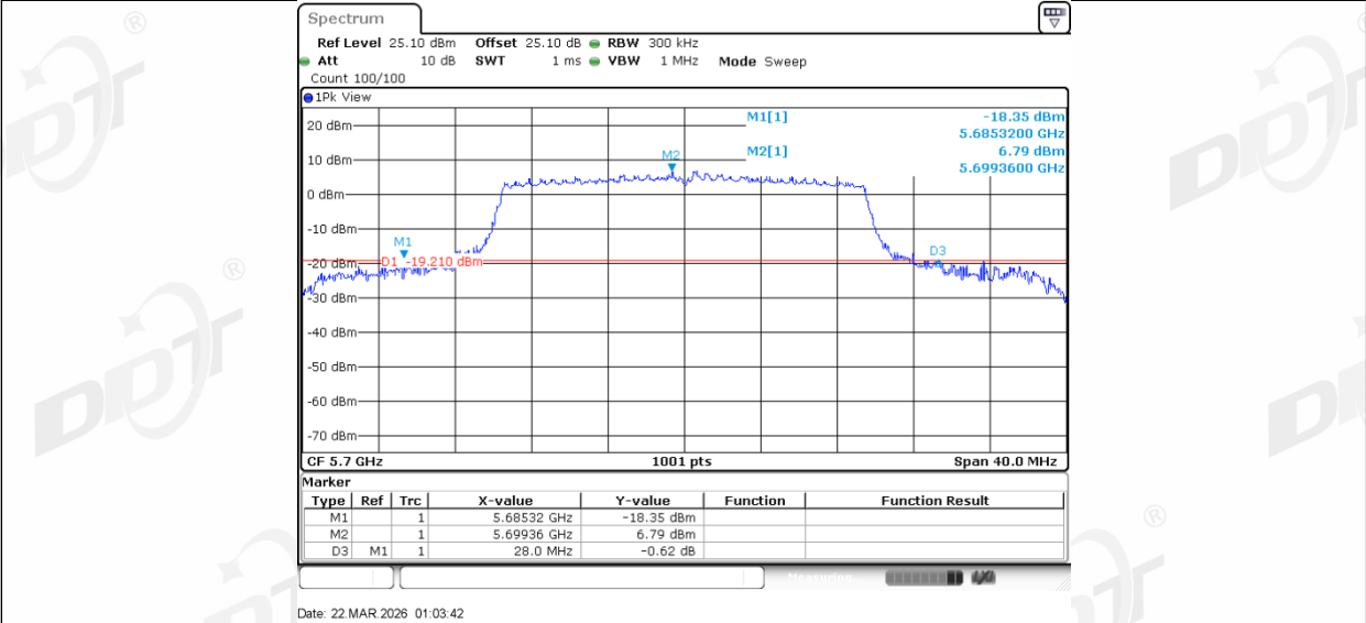
11AX20MIMO_Ant1_5720
