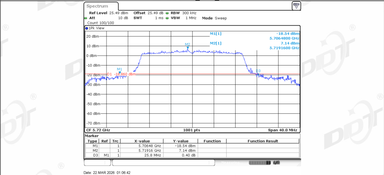
11AX20MIMO_Ant2_5720
