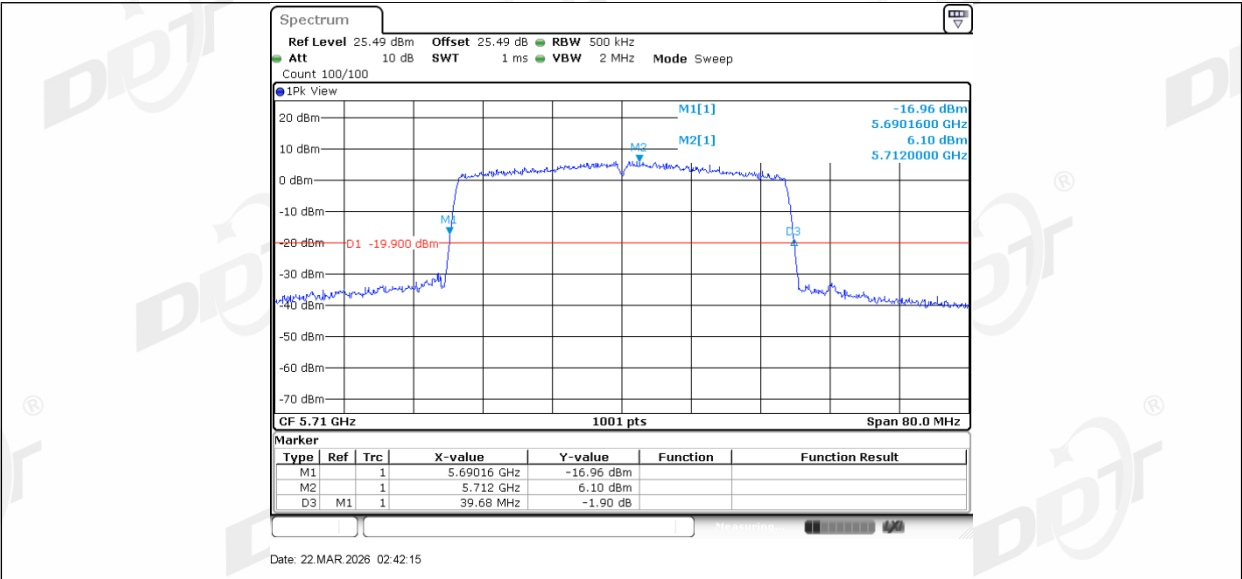
11AX40MIMO_Ant2_5710
