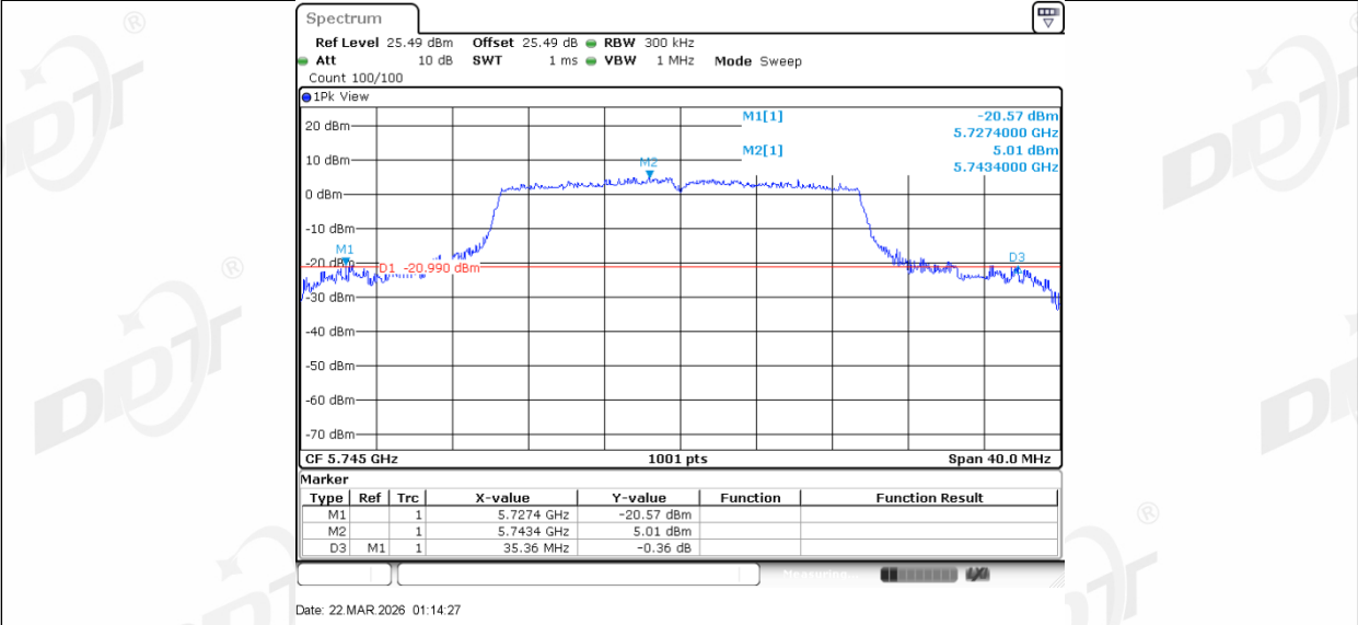
11AX20MIMO_Ant2_5745
