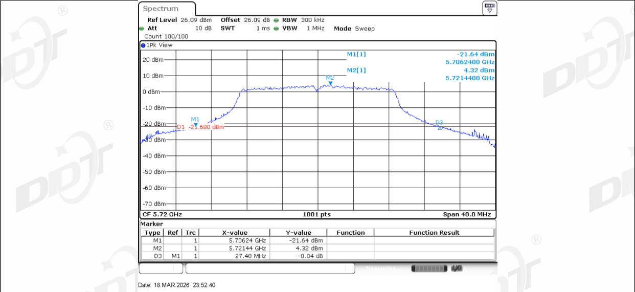
11AC20MIMO_Ant2_5720
