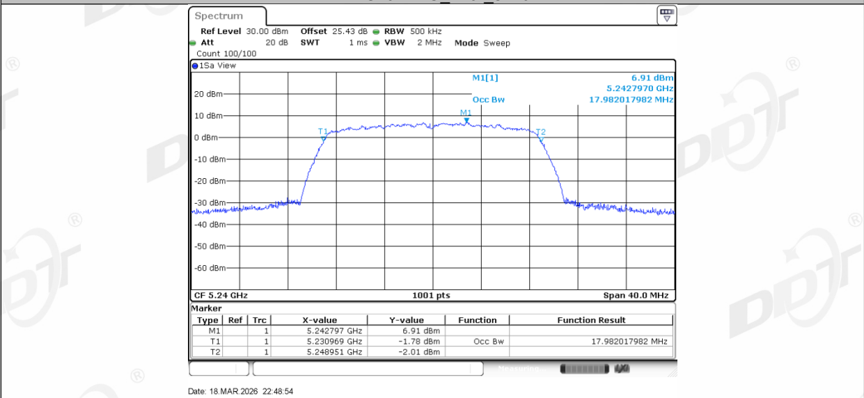
11AC20MIMO_Ant2_5240
