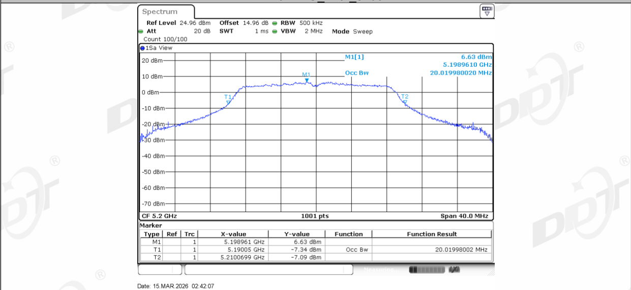
11N20MIMO_Ant2_5200
