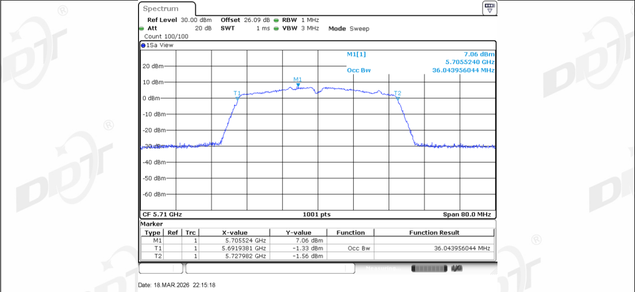
11N40MIMO_Ant2_5710
