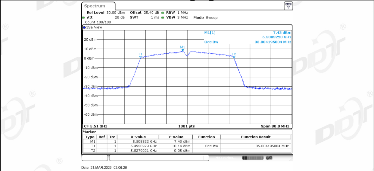
11AC40MIMO_Ant2_5510
