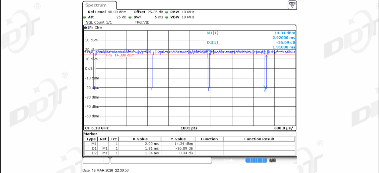
11AC20MIMO_Ant2_5180
