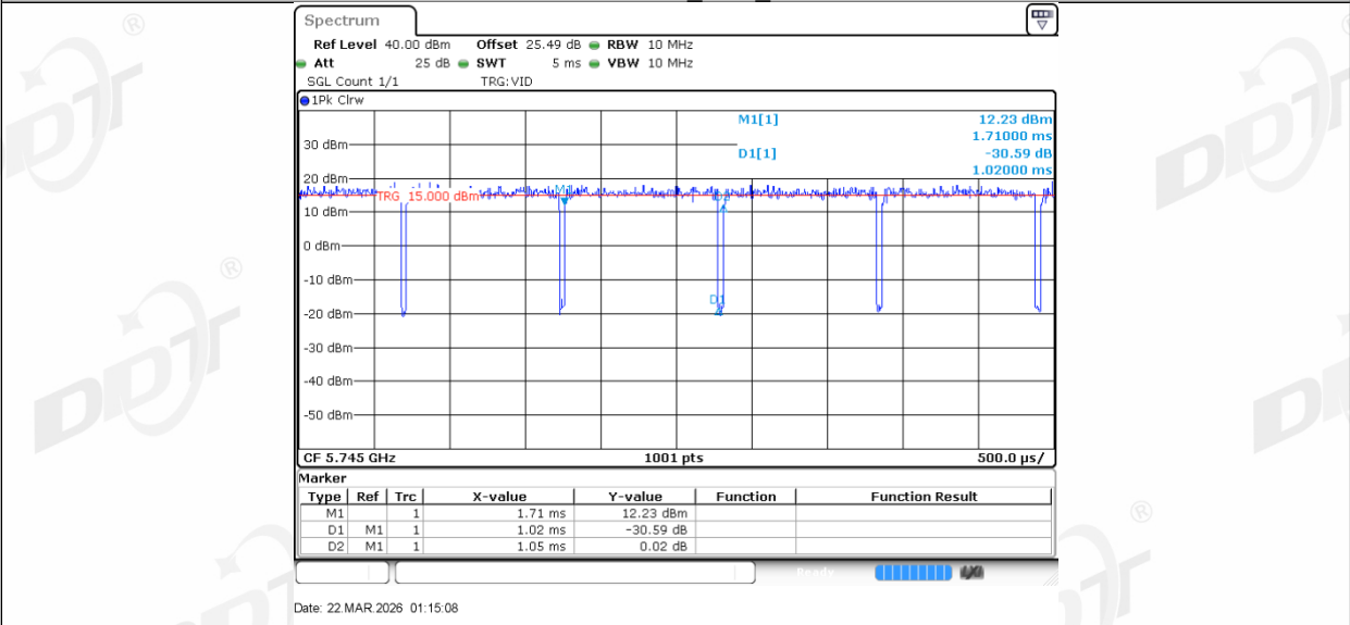
11AX20MIMO_Ant2_5745
