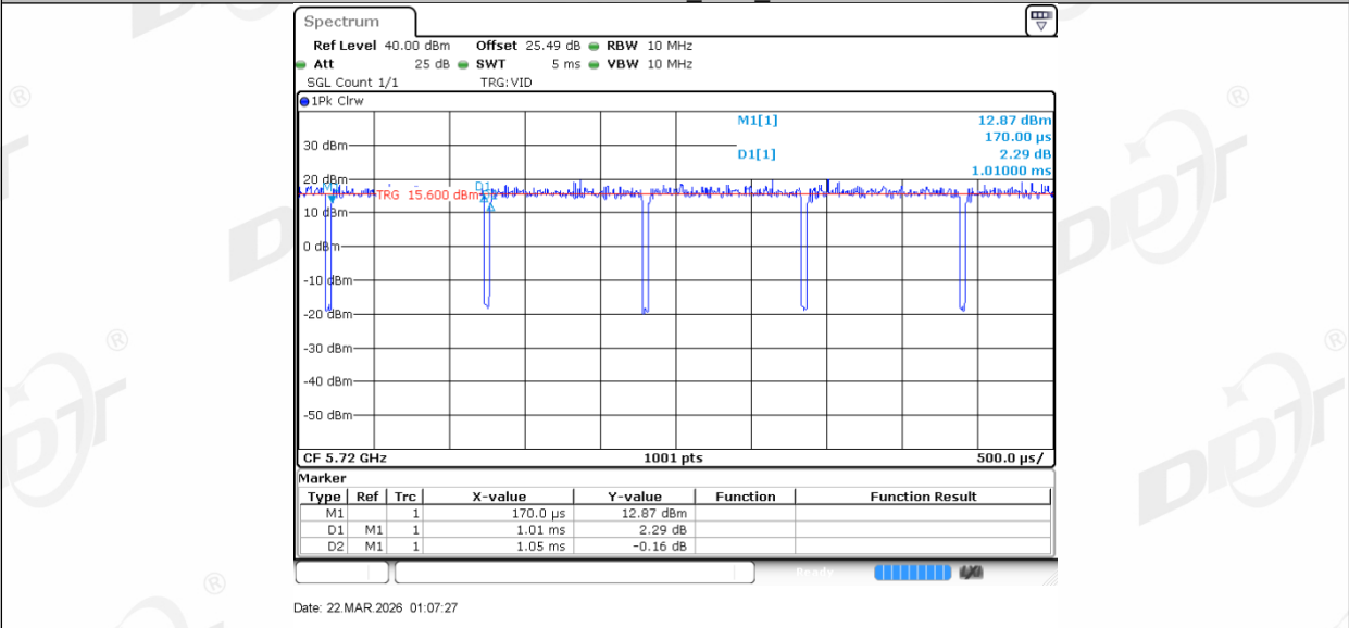
11AX20MIMO_Ant2_5720
