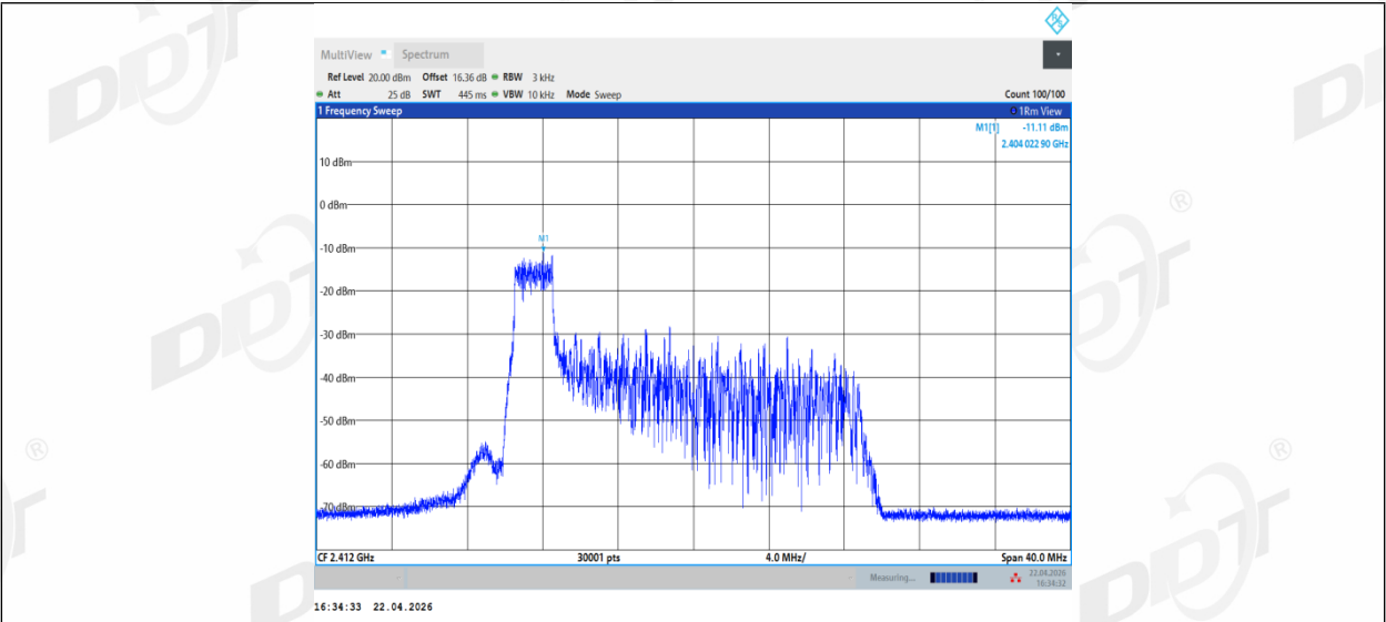
11AX20MIMO_Ant1_2412_52Tone_RU37
