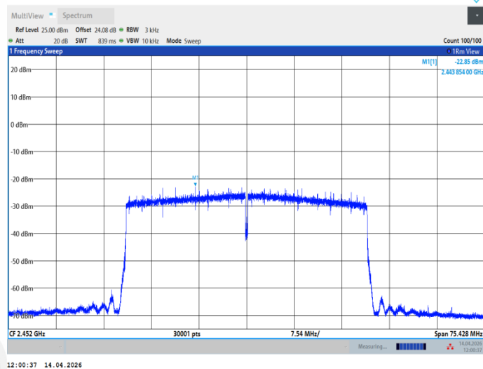
11AX40MIMO_Ant2_2452
