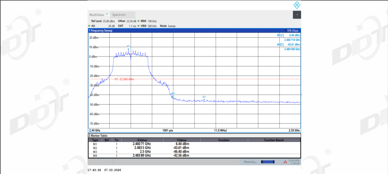
11N20MIMO_Ant2_High_2462
