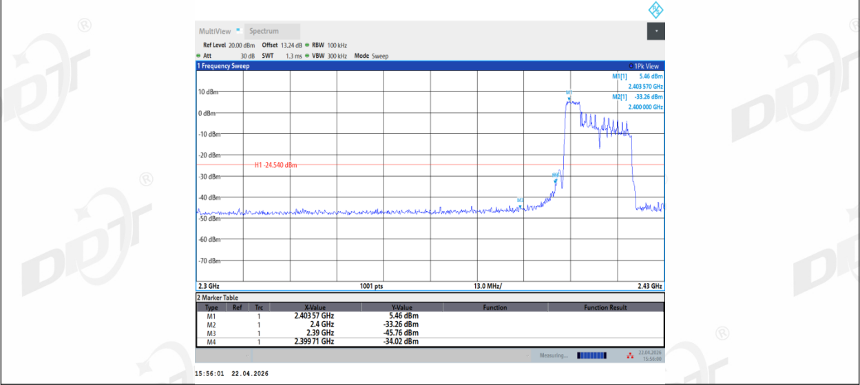
11AX20MIMO_Ant1_Low_2412_106Tone_RU53
