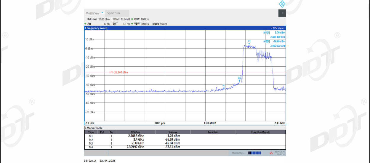
11AX20MIMO_Ant2_Low_2412_26Tone_RU0
