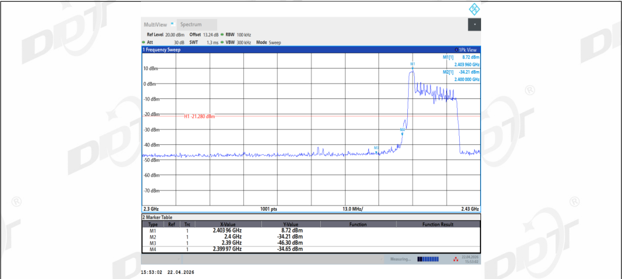
11AX20MIMO_Ant1_Low_2412_52Tone_RU37
