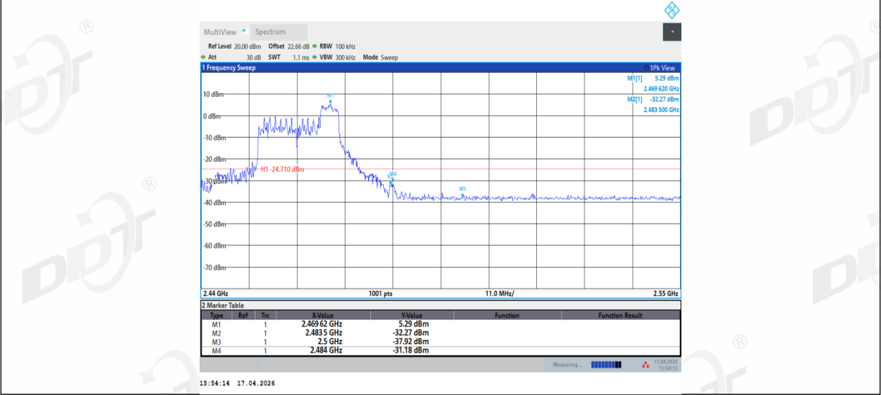
11AX20MIMO_Ant2_High_2462_106Tone_RU54
