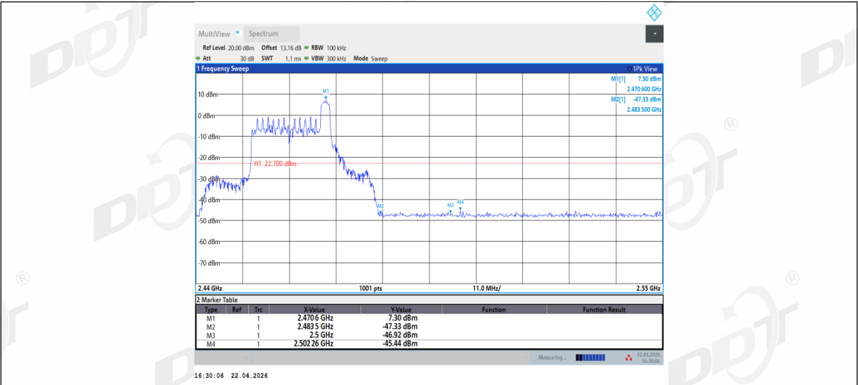
11AX20MIMO_Ant2_High_2462_52Tone_RU40
