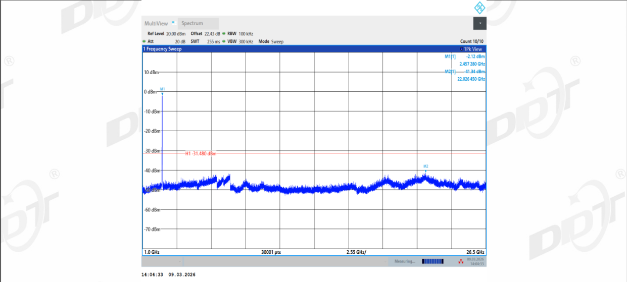
11N40MIMO_Ant2_2452_0~Reference
