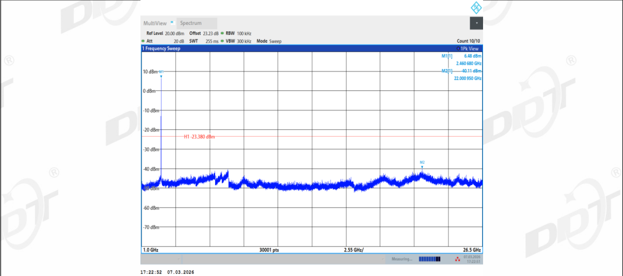
11N20MIMO_Ant1_2412_0~Reference
