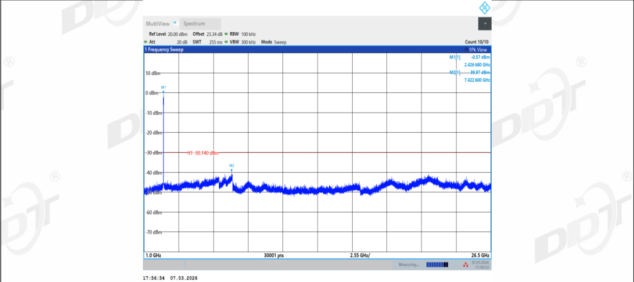
11N40MIMO_Ant1_2437_0~Reference
