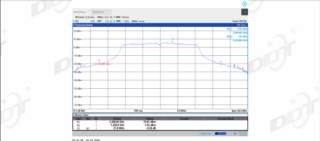
11AC20MIMO_Ant2_5280
