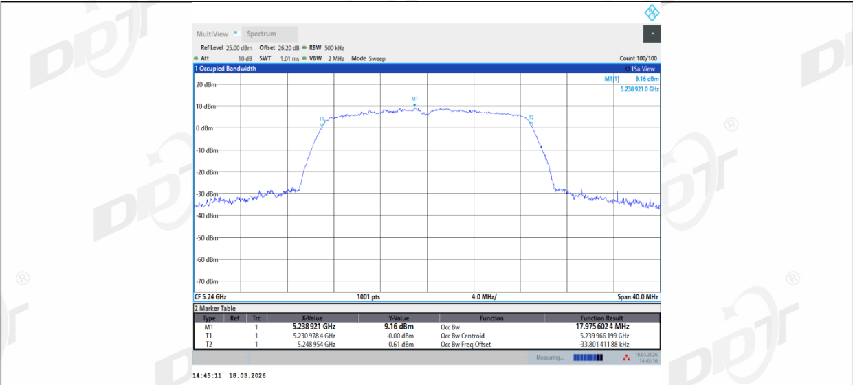
11N20MIMO_Ant2_5240
