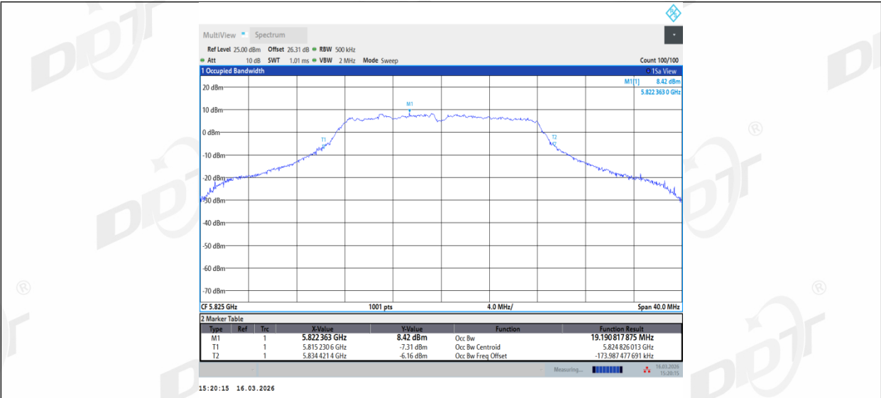
11A_Ant2_5825
