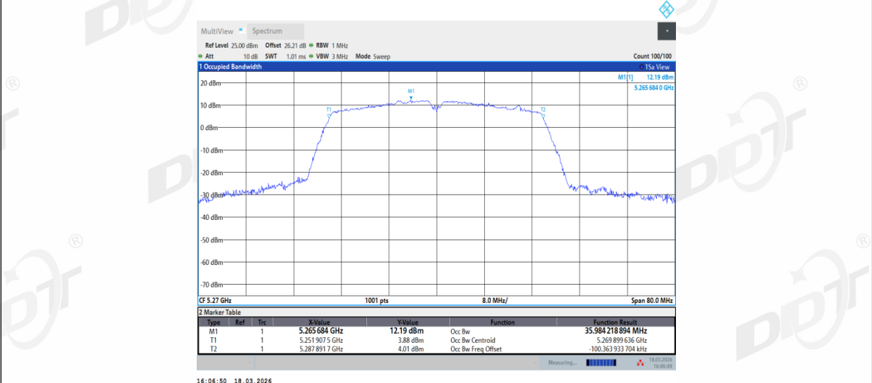
11N40MIMO_Ant2_5270
