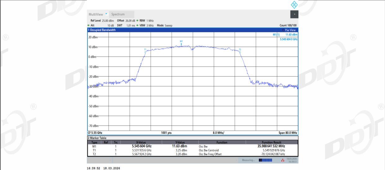
11N40MIMO_Ant2_5550
