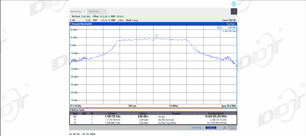
11N20MIMO_Ant2_5180
