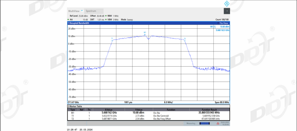
11AC40MIMO_Ant2_5670
