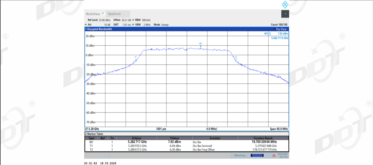
11AC20MIMO_Ant2_5280
