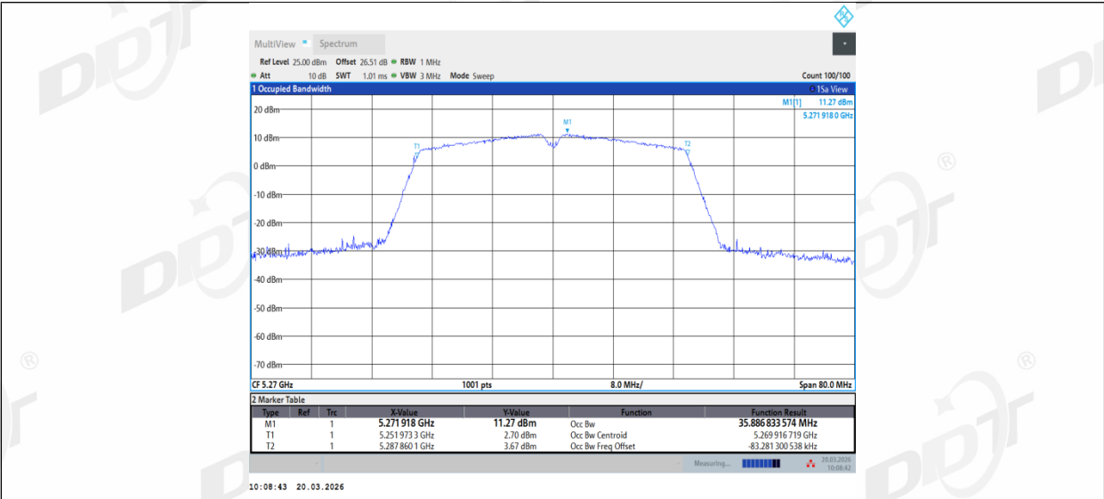
11AC40MIMO_Ant2_5270
