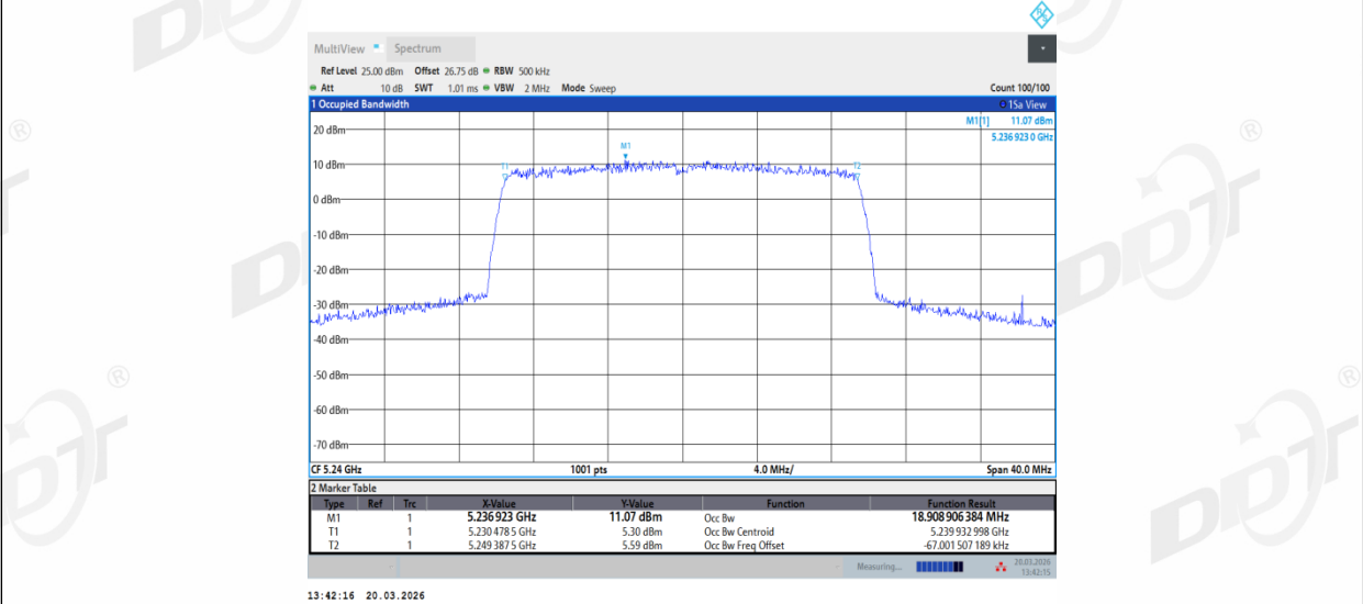
11AX20MIMO_Ant2_5240
