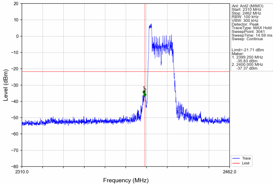
802.11ax(HEW40)_LCH_2422MHz_RU26_Left_Ant2 (MIMO)_NTNV
