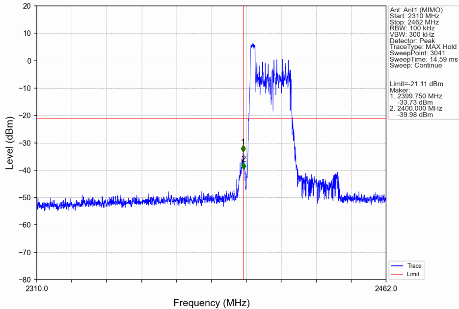
802.11ax(HEW40)_LCH_2422MHz_RU26_Left_Ant1 (MIMO)_NTNV
