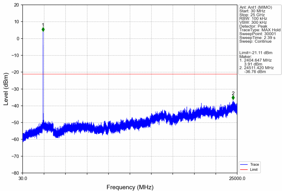
802.11ax(HEW40)_LCH_2422MHz_RU26_Left_Ant1 (MIMO)_NTNV
