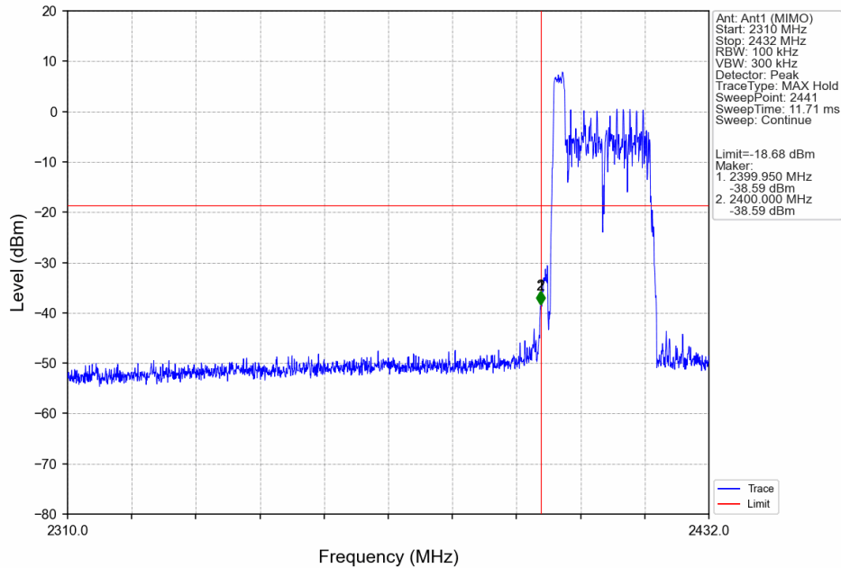
802.11ax(HEW20)_LCH_2412MHz_RU26_Left_Ant1 (MIMO)_NTNV
