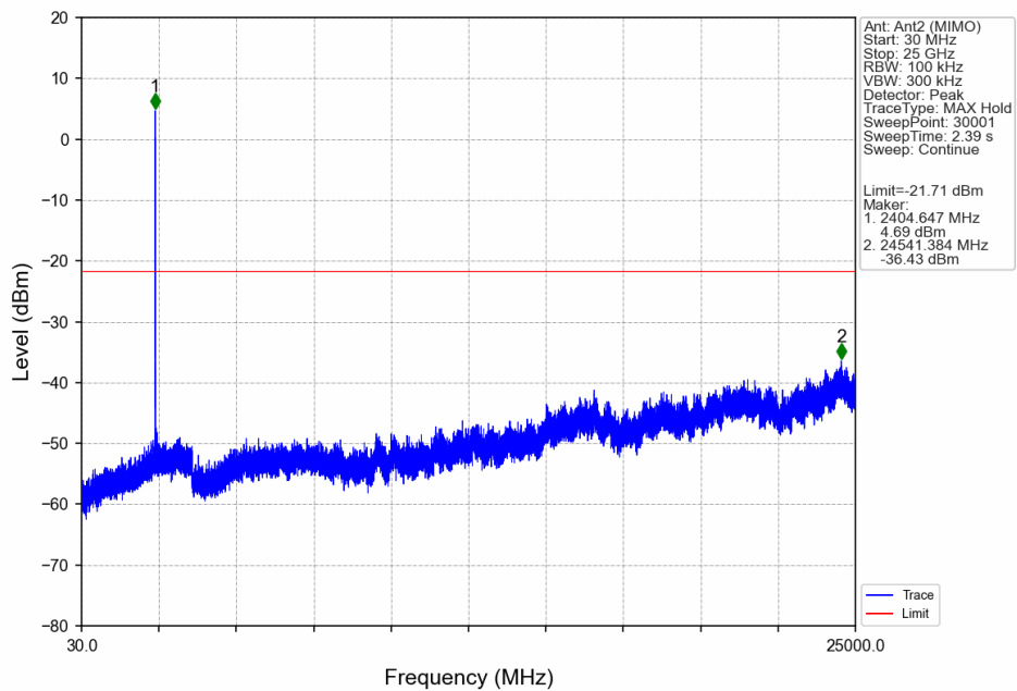
802.11ax(HEW40)_LCH_2422MHz_RU26_Left_Ant2 (MIMO)_NTNV
