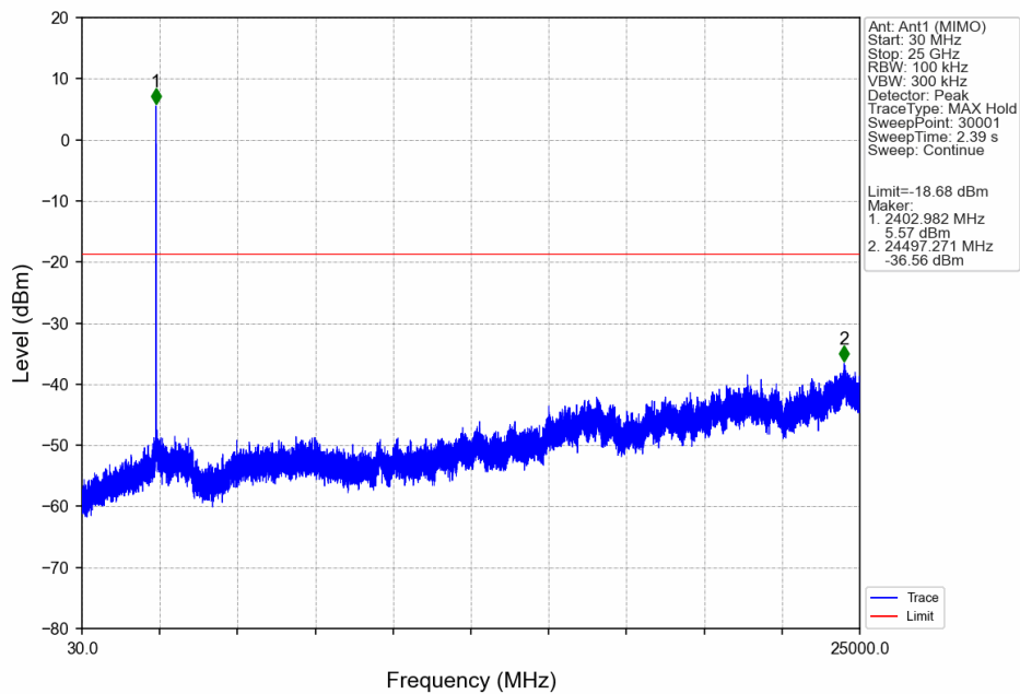
802.11ax(HEW20)_LCH_2412MHz_RU26_Left_Ant1 (MIMO)_NTNV
