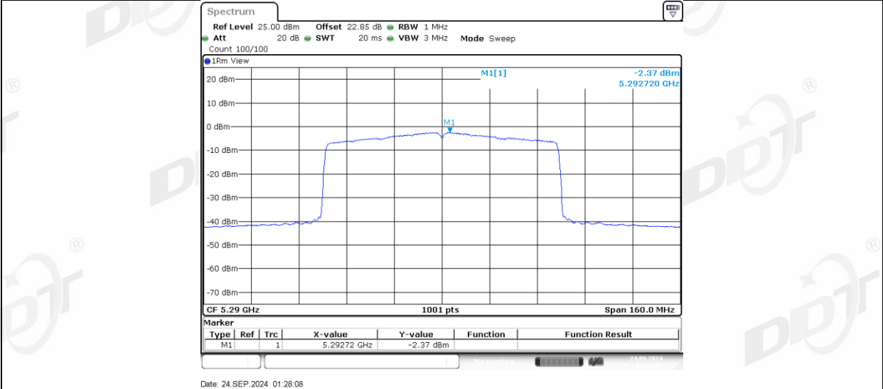
11AX80MIMO_Ant2_5290
