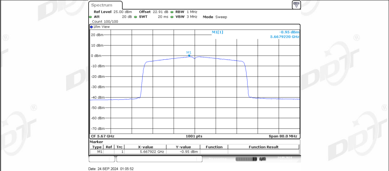
11AX40MIMO_Ant2_5670
