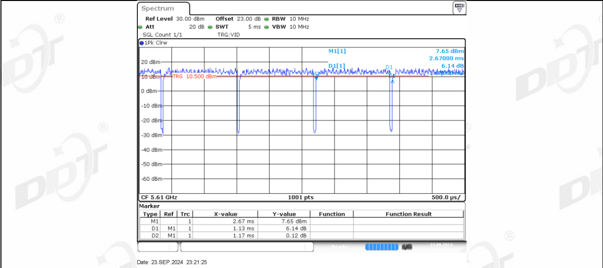
11AC80MIMO_Ant2_5610
