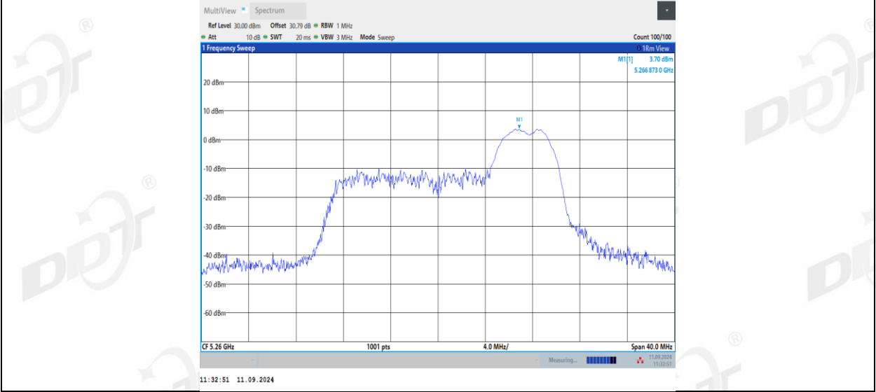
11AX20MIMO_Ant1_5260_106Tone_RU53
