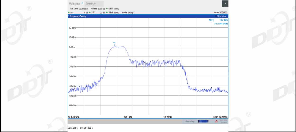
11AX20MIMO_Ant2_5180_52Tone_RU39
