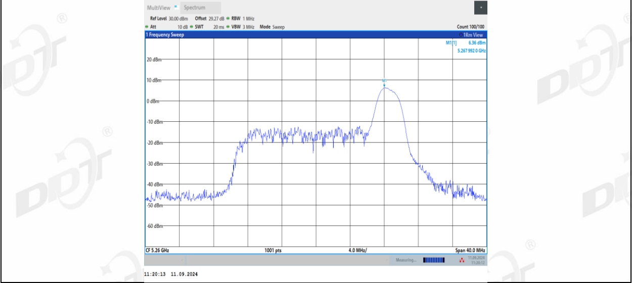
11AX20MIMO_Ant1_5260_52Tone_RU37
