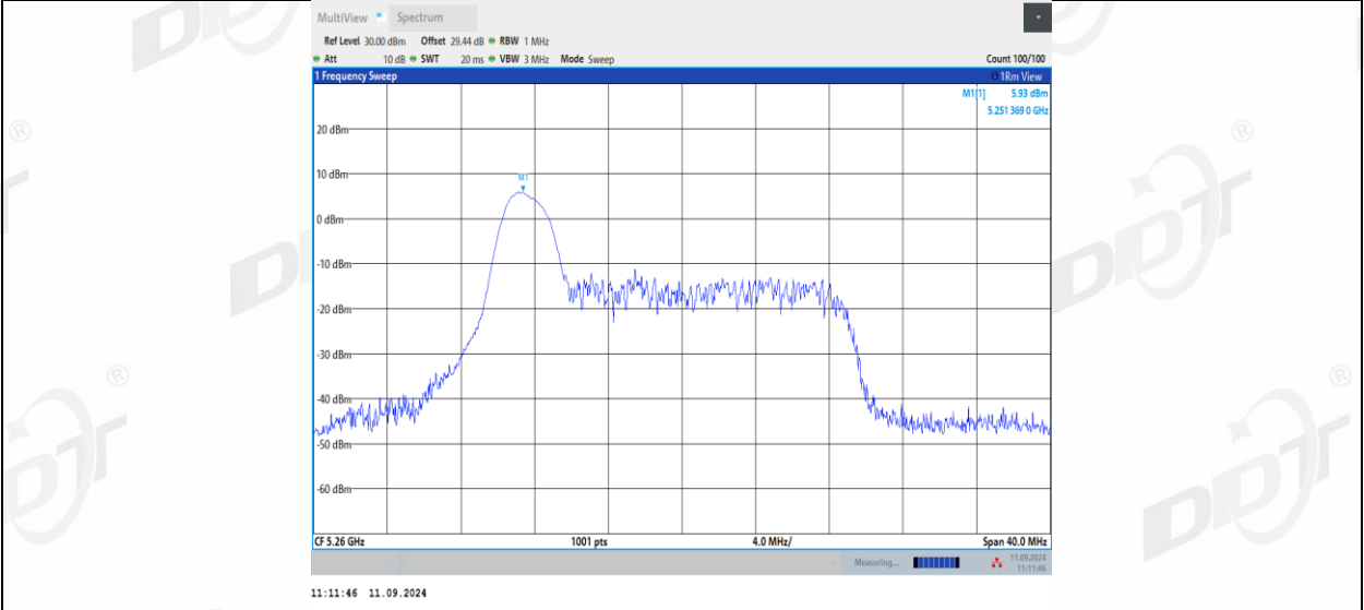
11AX20MIMO_Ant1_5260_26Tone_RU4
