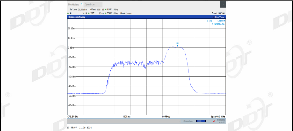
11AX20MIMO_Ant1_5240_106Tone_RU53
