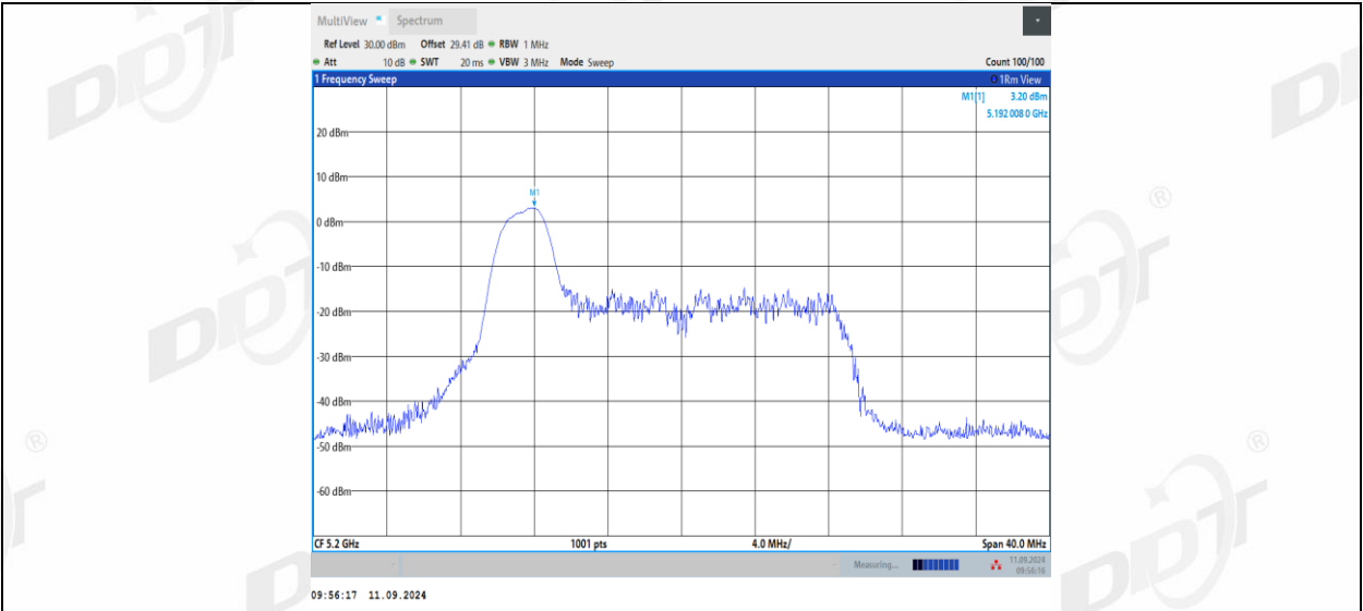
11AX20MIMO_Ant1_5200_26Tone_RU4
