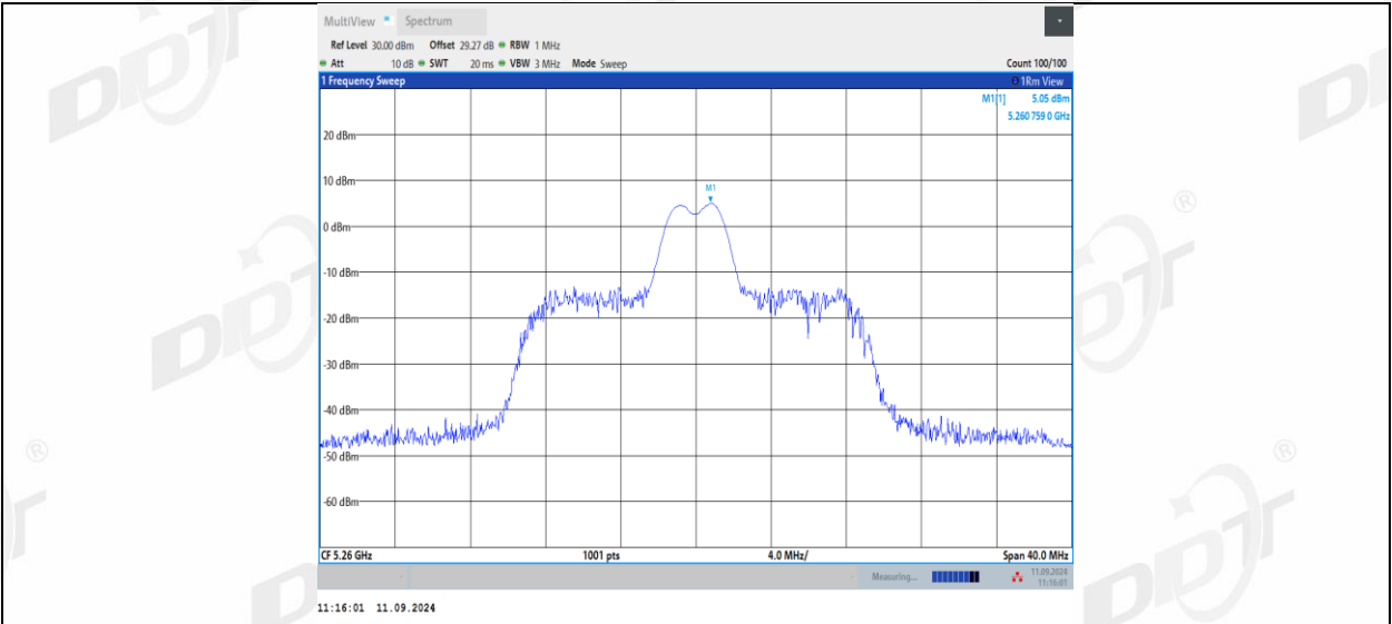
11AX20MIMO_Ant1_5260_26Tone_RU8
