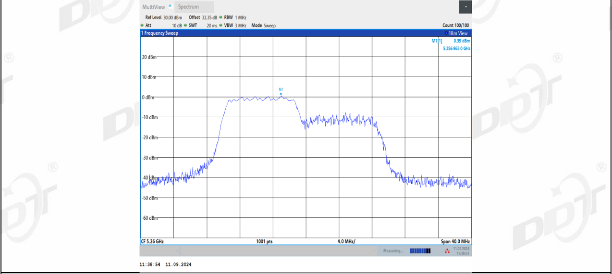
11AX20MIMO_Ant1_5260_106Tone_RU54
