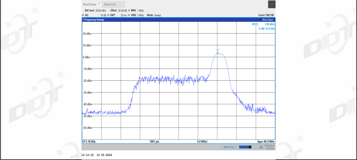
11AX20MIMO_Ant1_5180_52Tone_RU37
