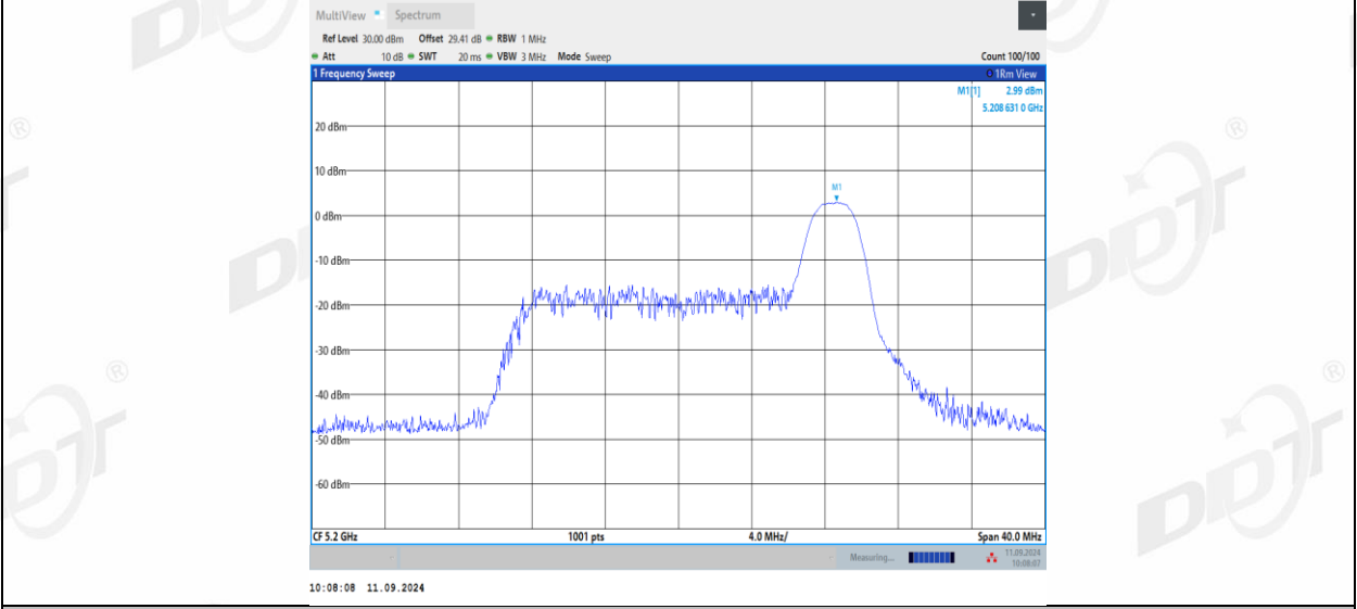
11AX20MIMO_Ant1_5200_52Tone_RU37
