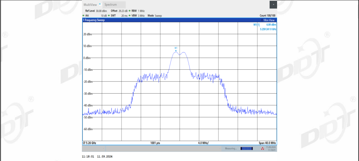
11AX20MIMO_Ant2_5260_26Tone_RU8
