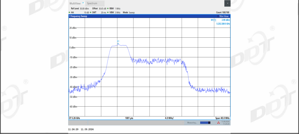
11AX20MIMO_Ant1_5260_52Tone_RU39
