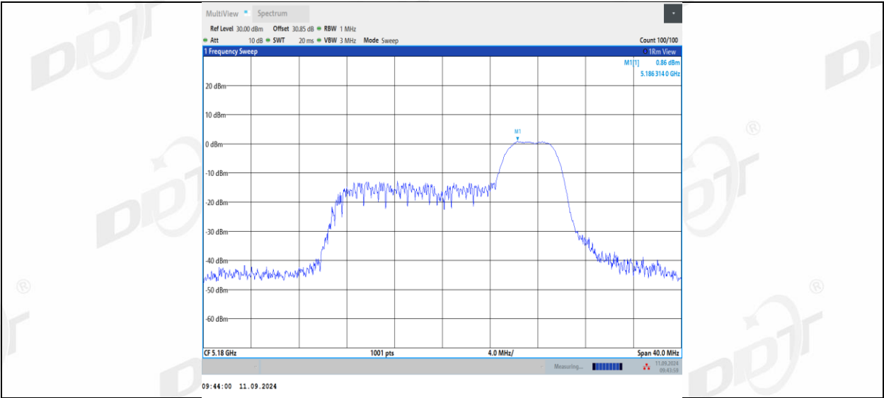
11AX20MIMO_Ant2_5180_106Tone_RU53
