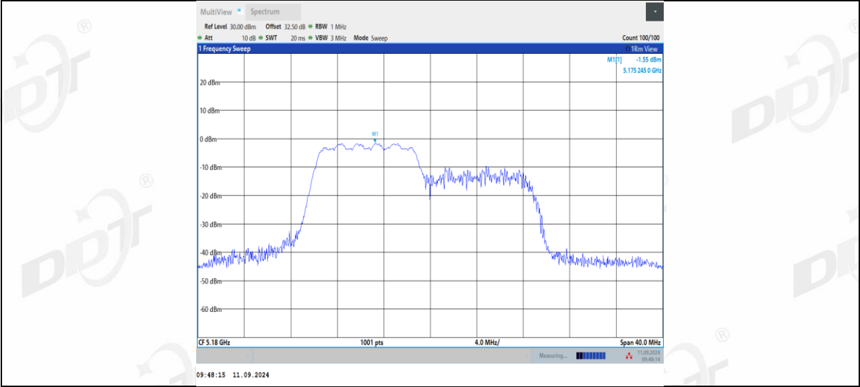
11AX20MIMO_Ant2_5180_106Tone_RU54
