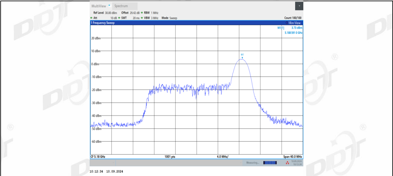
11AX20MIMO_Ant2_5180_52Tone_RU37
