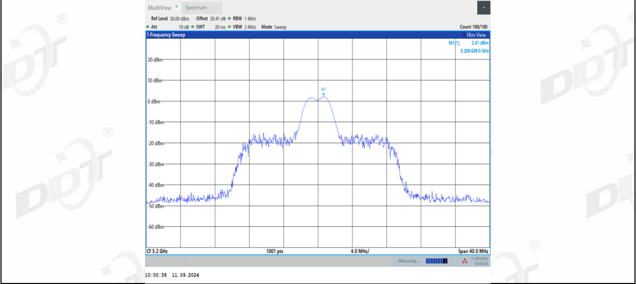
11AX20MIMO_Ant1_5200_26Tone_RU8
