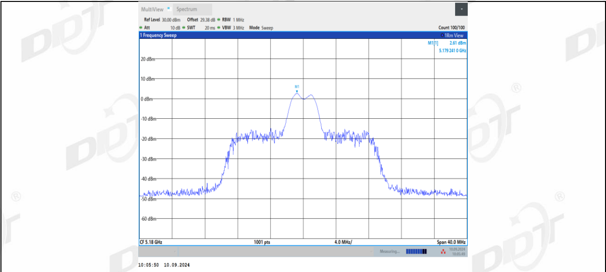
11AX20MIMO_Ant1_5180_26Tone_RU8
