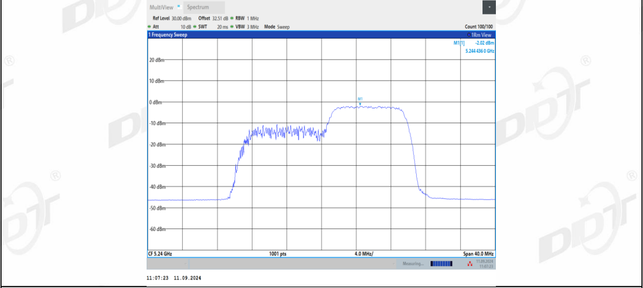
11AX20MIMO_Ant2_5240_26Tone_RU0
