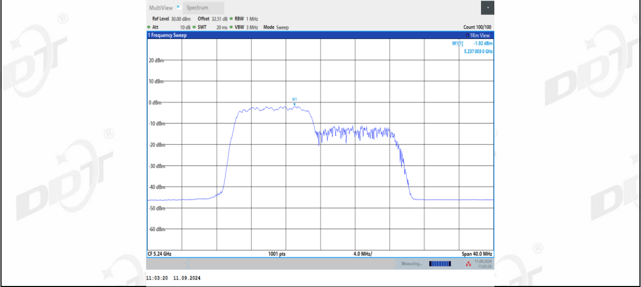
11AX20MIMO_Ant1_5240_106Tone_RU54
