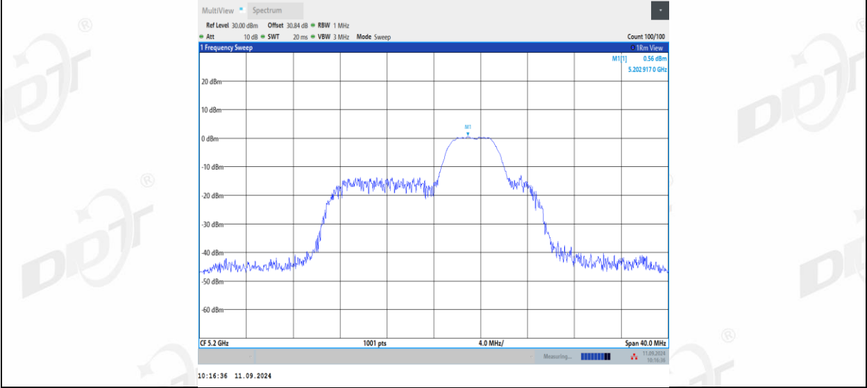
11AX20MIMO_Ant1_5200_52Tone_RU40
