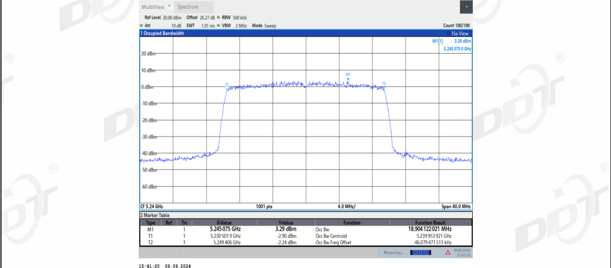
11AX20MIMO_Ant2_5240
