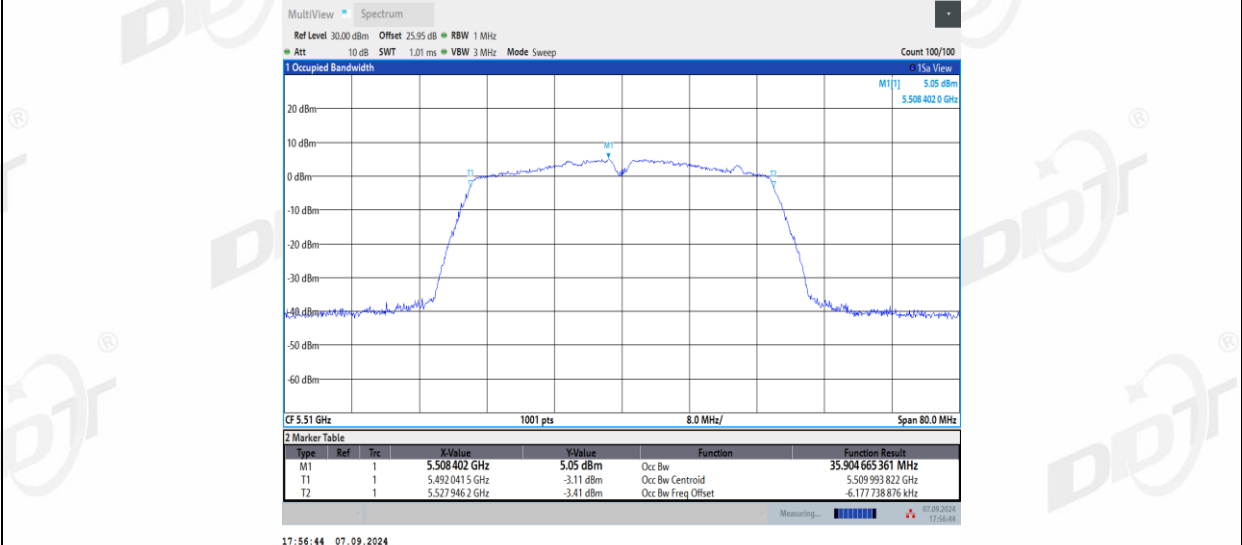
11N40MIMO_Ant2_5510
