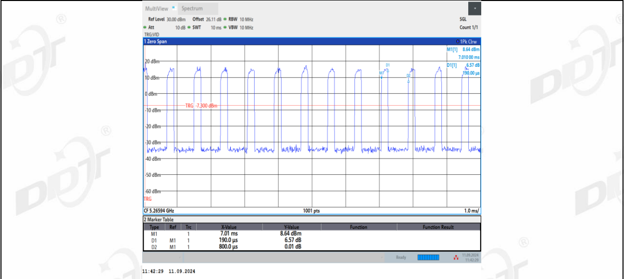
11AX20MIMO_Ant2_5260_26Tone_RU0
