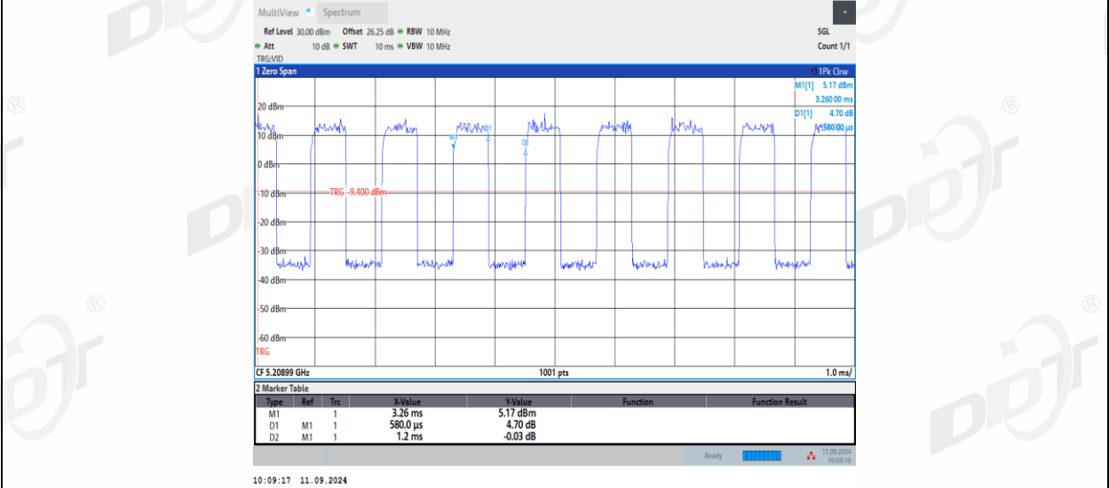
11AX20MIMO_Ant2_5200_52Tone_RU37
