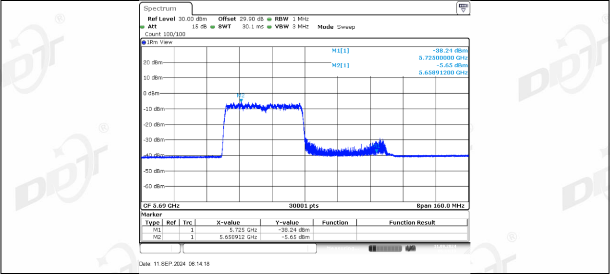
11AX80MIMO_Ant2_5690_UNII-2C_484Tone_RU66
