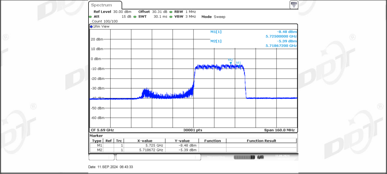
11AX80MIMO_Ant1_5690_UNII-3_242Tone_RU61
