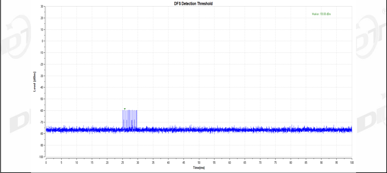
11AC80MIMO_5290_Type5
