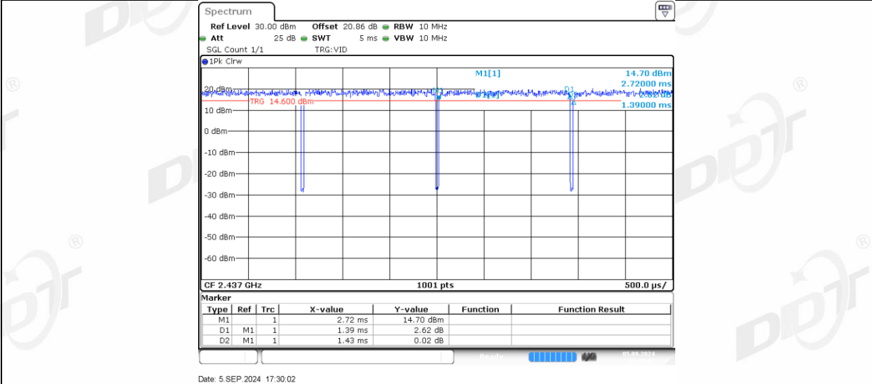
11G_Ant2_2437
