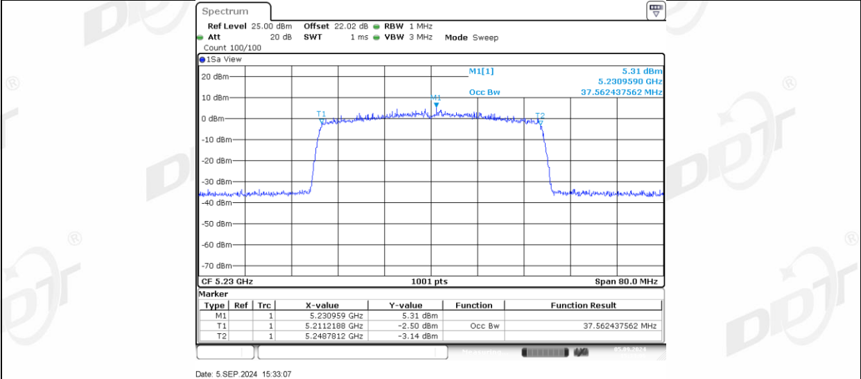
11AX40MIMO_Ant2_5230
