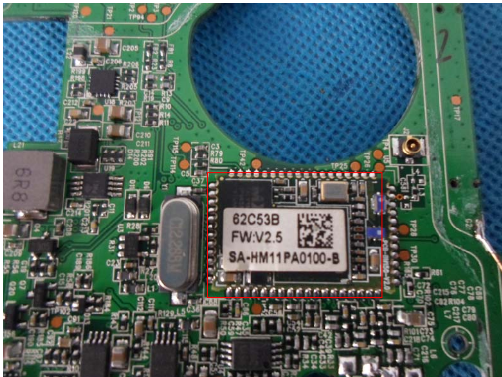
Photo 11 BT module
