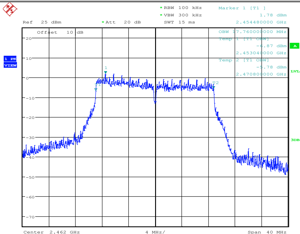
Occupied Bandwidth_11N20MIMO_2462_Ant1
