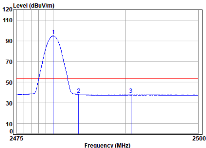
BLE_1M_TX_CH_39_Verical-AVG
