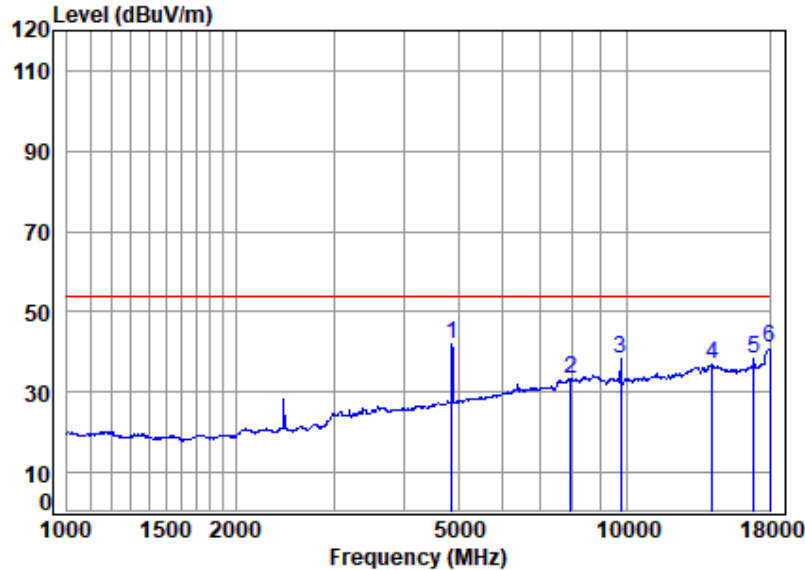
BLE_2M_TX_CH_19_Vertical-Avg
