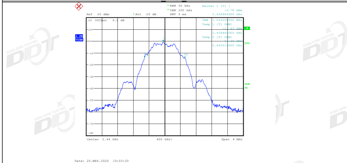
BLE_Ant2_2440
