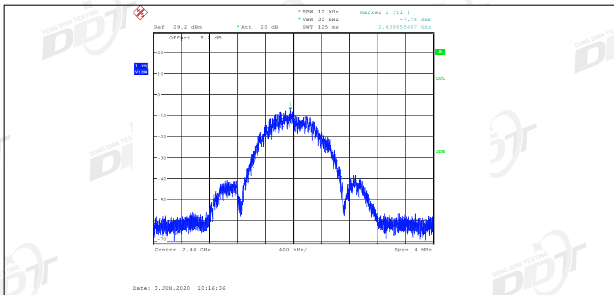
BLE_Ant2_2440
