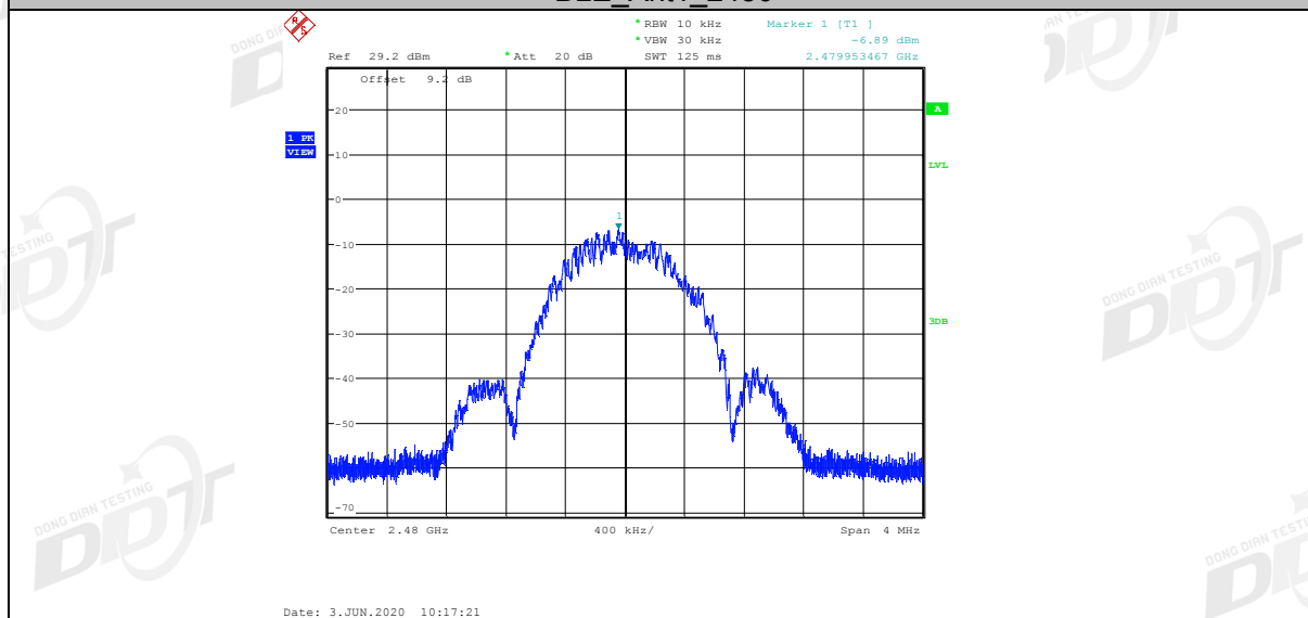
BLE_Ant2_2480
