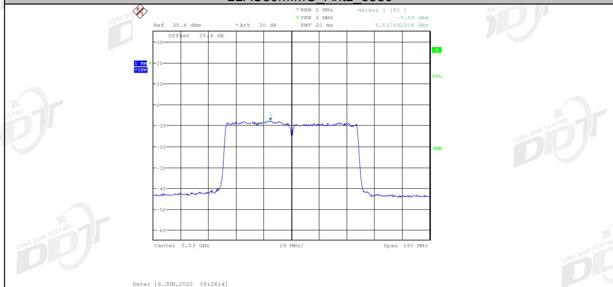
11AC80MIMO_Ant2_5530
