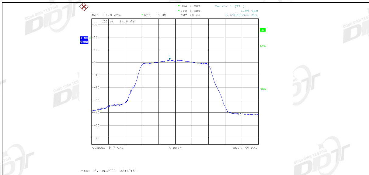
11A_Ant1_5745
