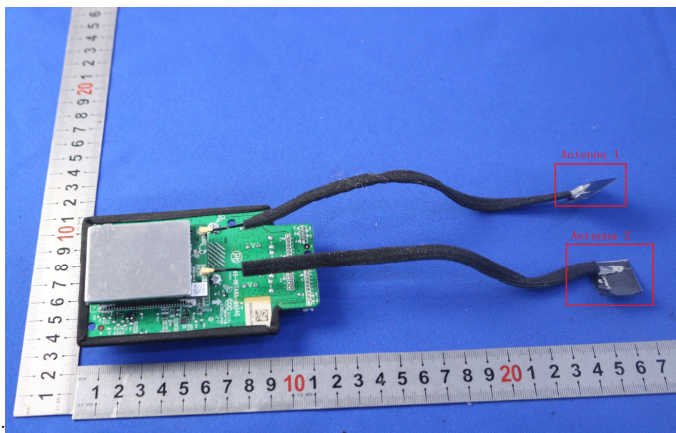
EUT Antenna:
