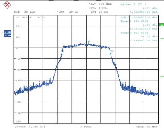
11A_ANT1_5825_99% Bandwidth
