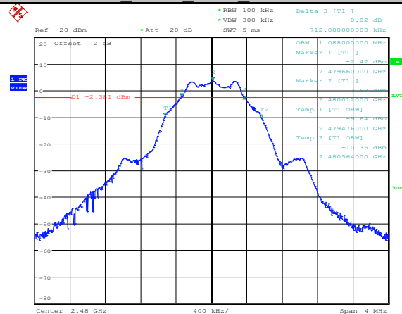
BLE ANT1 2480 6 dB bandwidth
