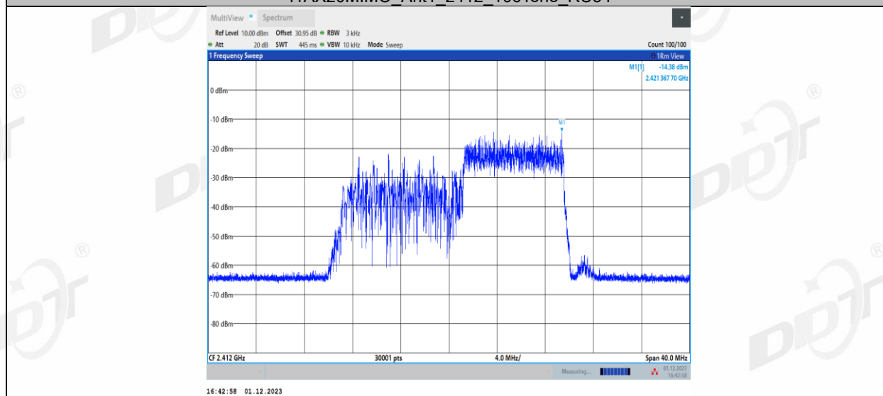
11AX20MIMO_Ant2_2412_26Tone_RU0
