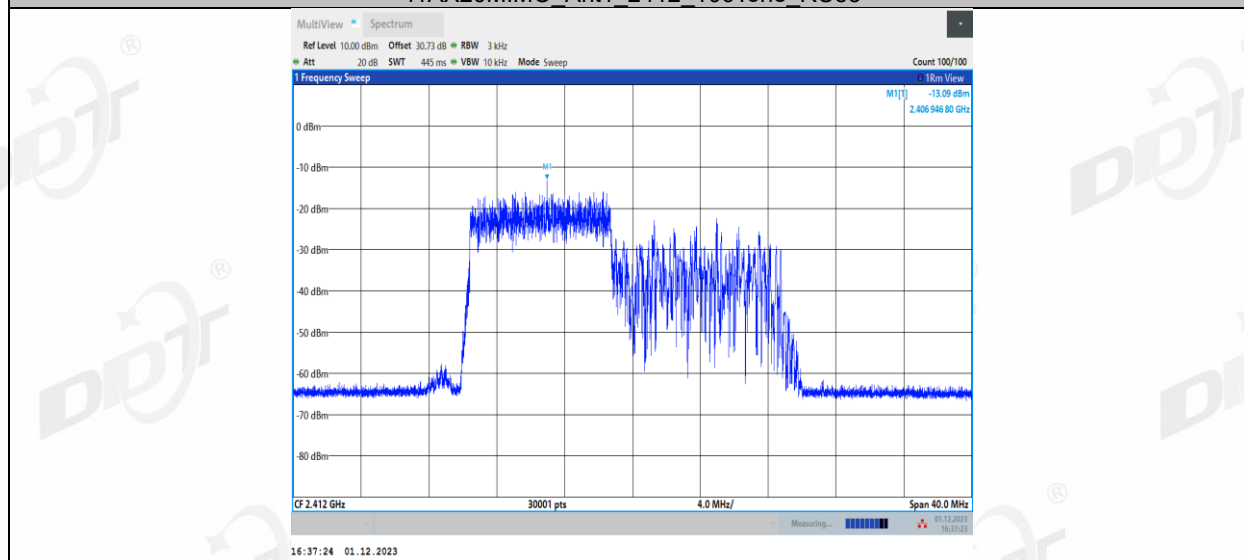
11AX20MIMO_Ant1_2412_106Tone_RU54
