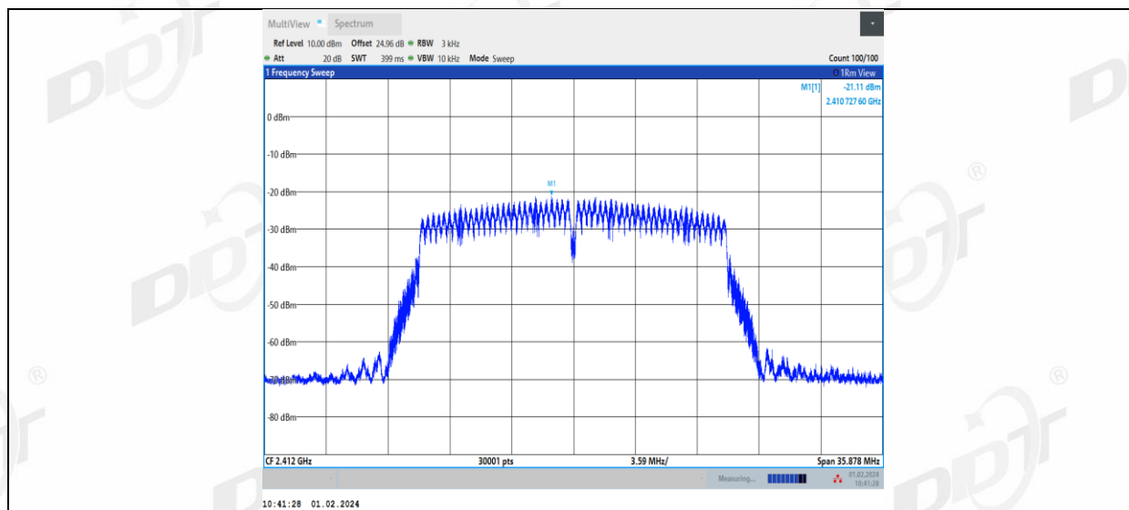
11N20MIMO_Ant2_2412
