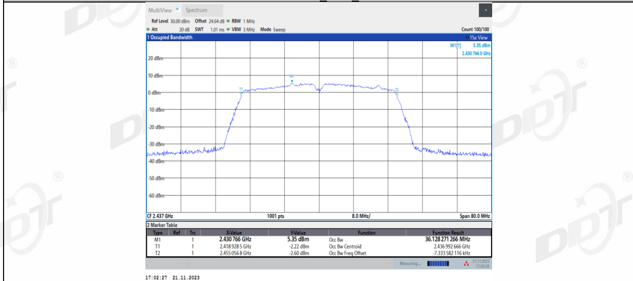
11N40MIMO_Ant2_2437
