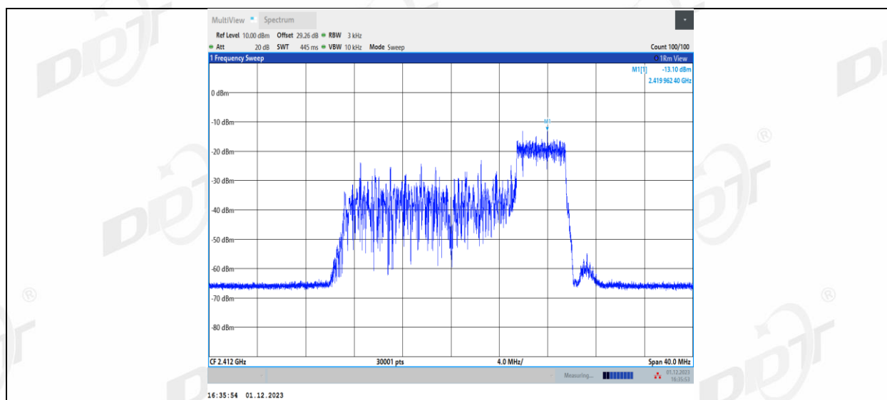
11AX20MIMO_Ant1_2412_106Tone_RU53
