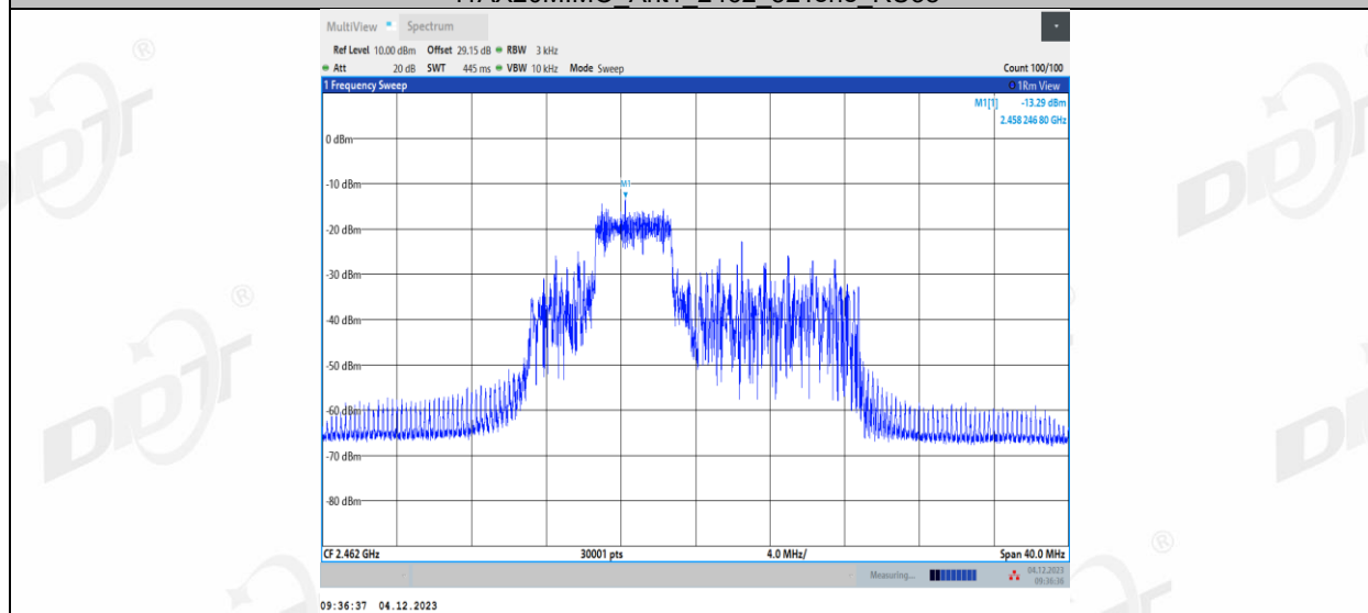
11AX20MIMO_Ant1_2462_52Tone_RU39
