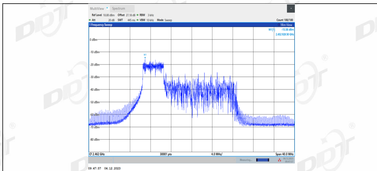
11AX20MIMO_Ant2_2462_52Tone_RU38
