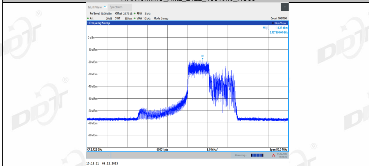
11AX40MIMO_Ant2_2422_106Tone_RU56
