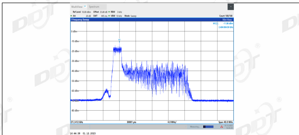
11AX20MIMO_Ant2_2412_26Tone_RU4
