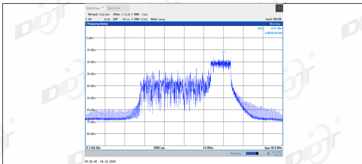
11AX20MIMO_Ant2_2462_106Tone_RU53
