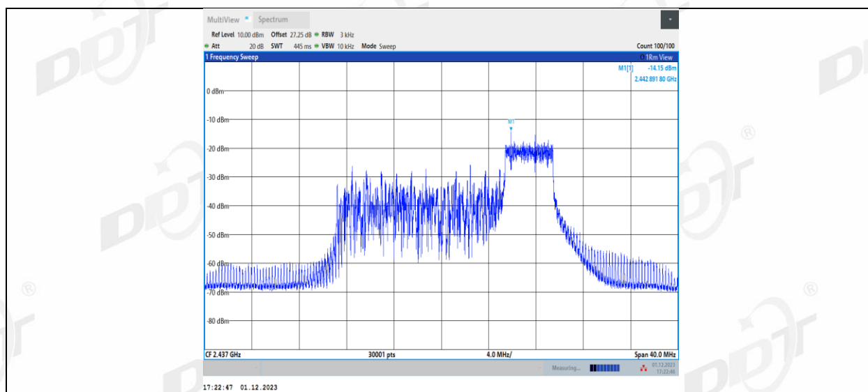
11AX20MIMO_Ant2_2437_106Tone_RU53
