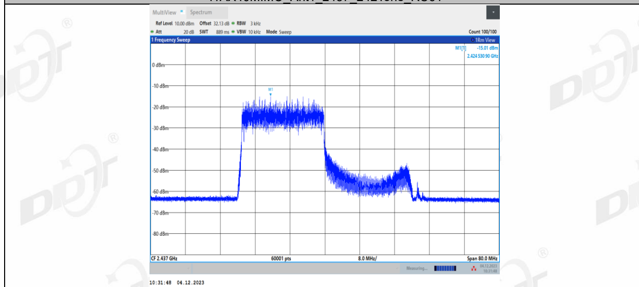
11AX40MIMO_Ant1_2437_242Tone_RU62
