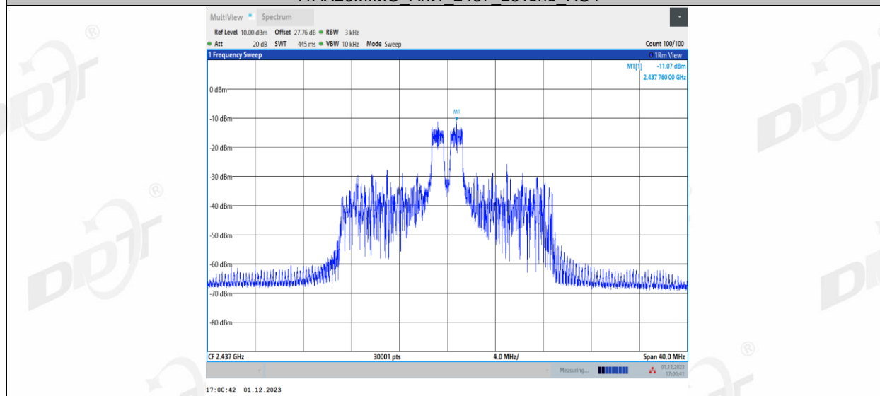
11AX20MIMO_Ant1_2437_26Tone_RU8
