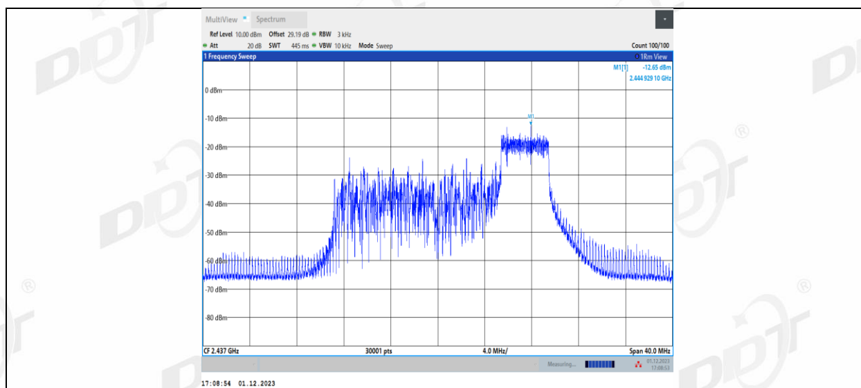
11AX20MIMO_Ant1_2437_106Tone_RU53
