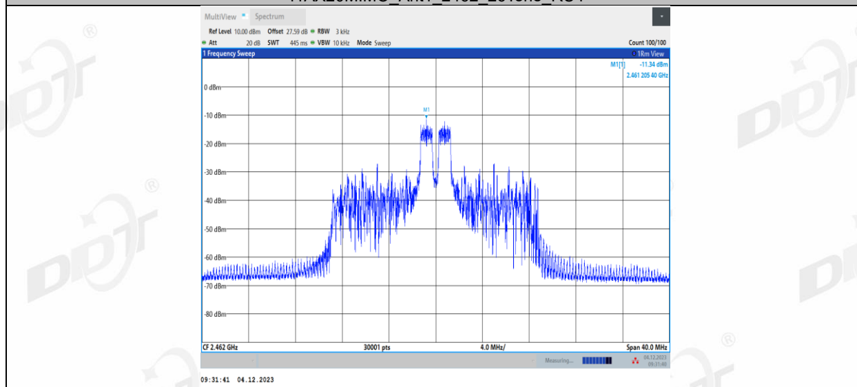
11AX20MIMO_Ant1_2462_26Tone_RU8
