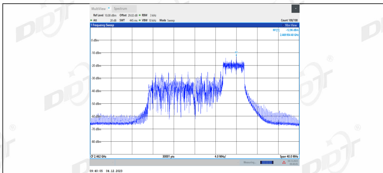
11AX20MIMO_Ant1_2462_106Tone_RU53
