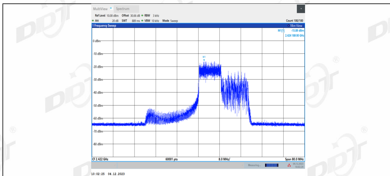
11AX40MIMO_Ant1_2422_106Tone_RU56
