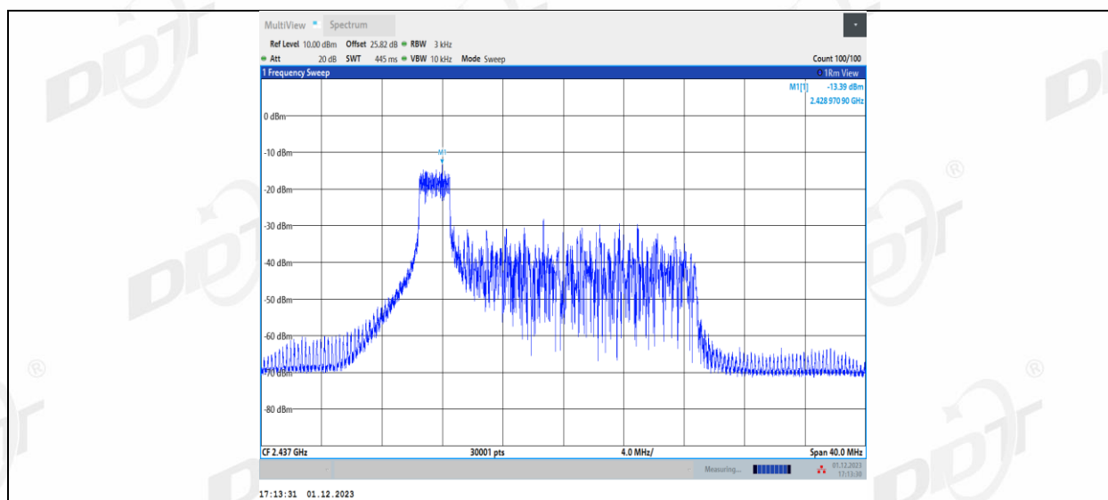
11AX20MIMO_Ant2_2437_26Tone_RU4
