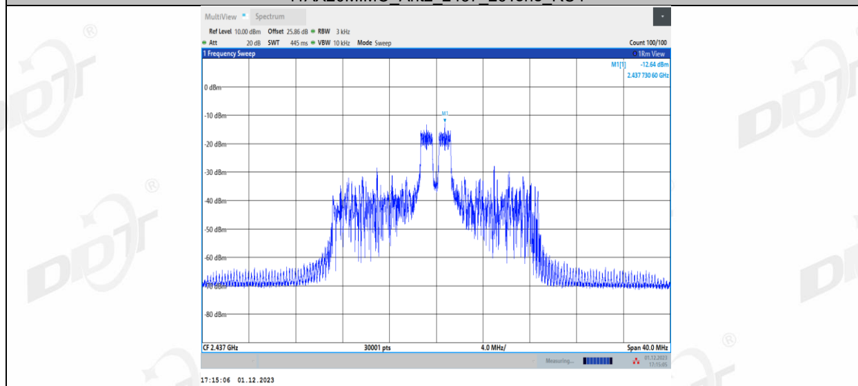
11AX20MIMO_Ant2_2437_26Tone_RU8
