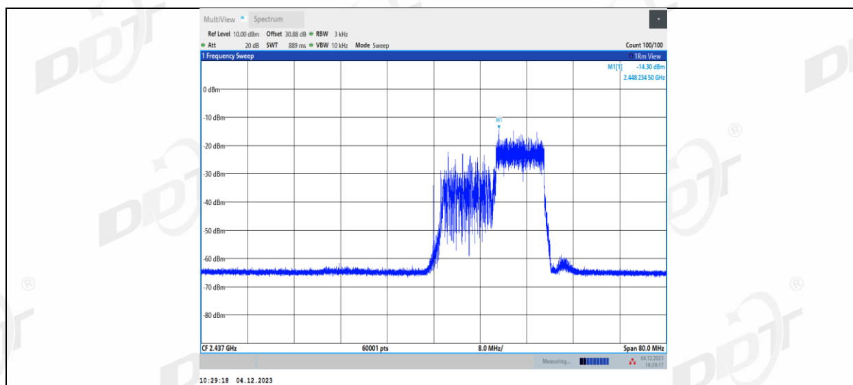
11AX40MIMO_Ant1_2437_242Tone_RU61
