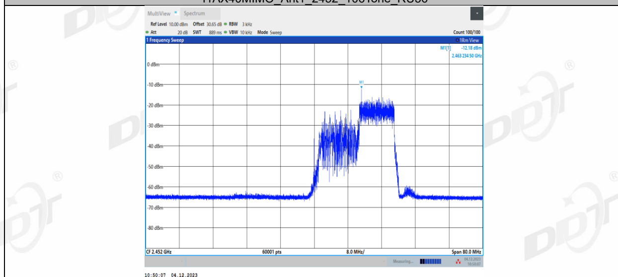
11AX40MIMO_Ant1_2452_242Tone_RU61
