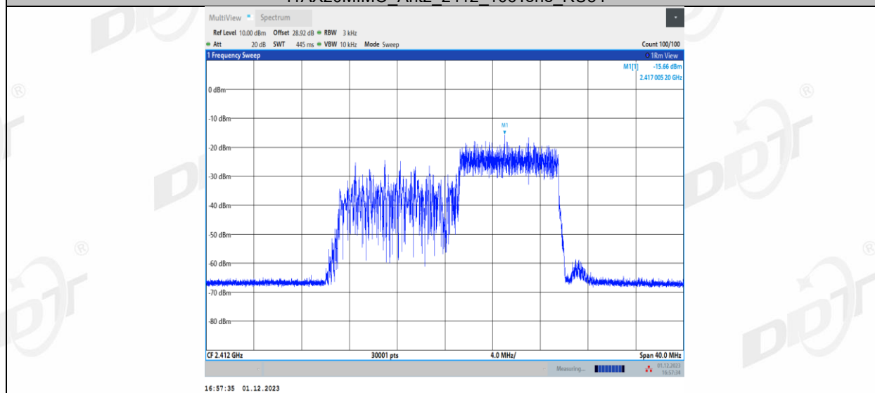
11AX20MIMO_Ant1_2437_26Tone_RU0
