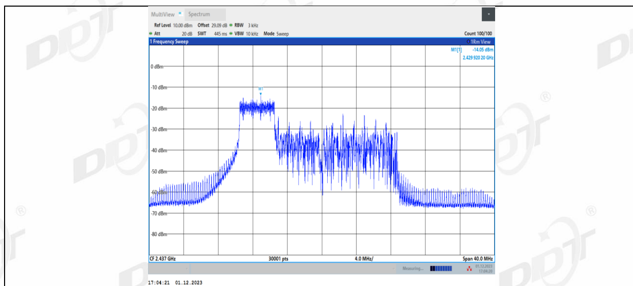
11AX20MIMO_Ant1_2437_52Tone_RU38
