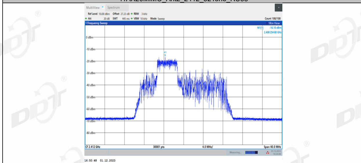
11AX20MIMO_Ant2_2412_52Tone_RU39
