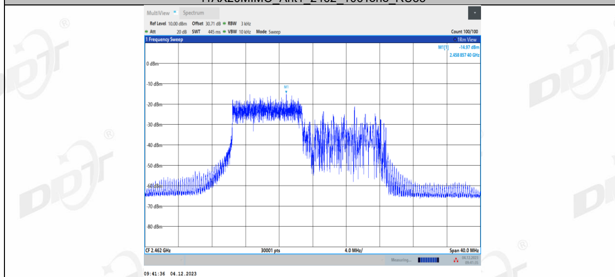
11AX20MIMO_Ant1_2462_106Tone_RU54
