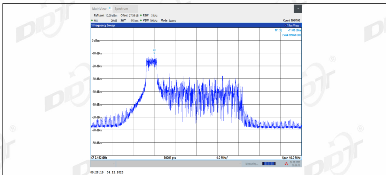
11AX20MIMO_Ant1_2462_26Tone_RU4
