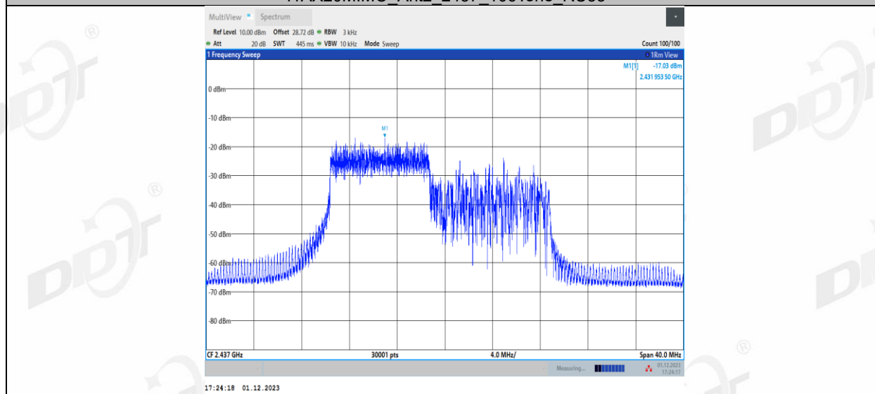
11AX20MIMO_Ant2_2437_106Tone_RU54
