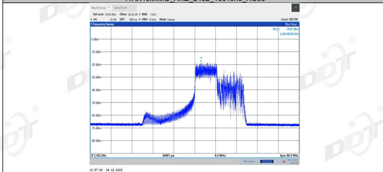
11AX40MIMO_Ant2_2452_106Tone_RU56
