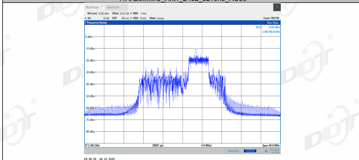
11AX20MIMO_Ant1_2462_52Tone_RU40
