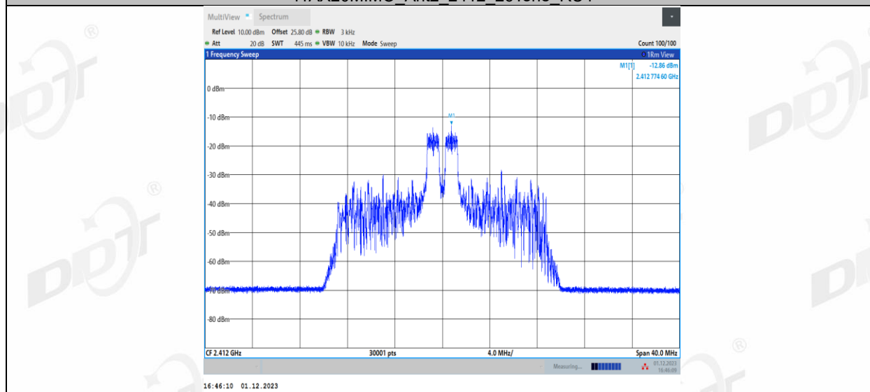
11AX20MIMO_Ant2_2412_26Tone_RU8
