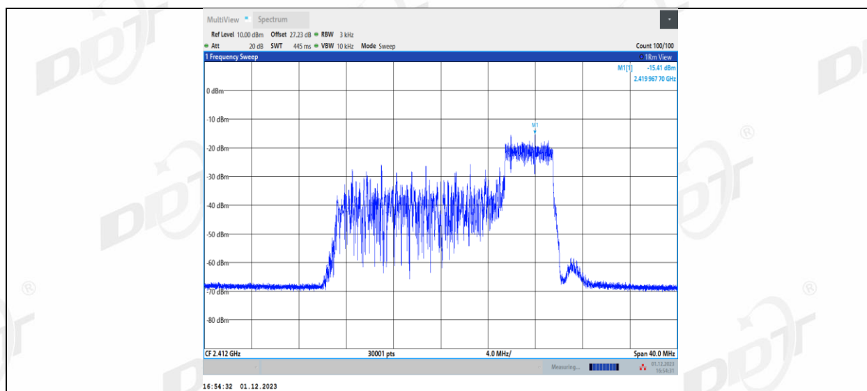
11AX20MIMO_Ant2_2412_106Tone_RU53
