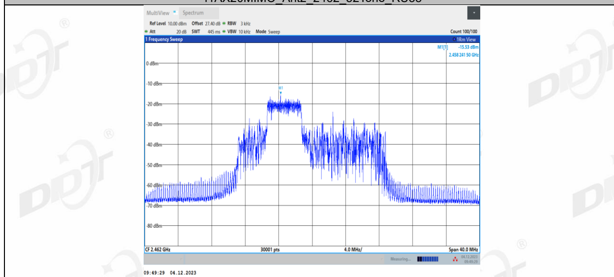
11AX20MIMO_Ant2_2462_52Tone_RU39
