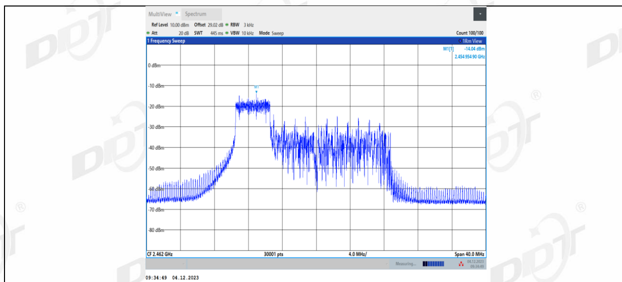
11AX20MIMO_Ant1_2462_52Tone_RU38
