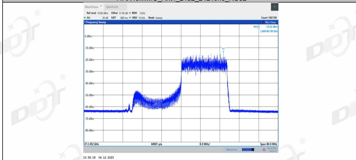
11AX40MIMO_Ant2_2452_106Tone_RU55
