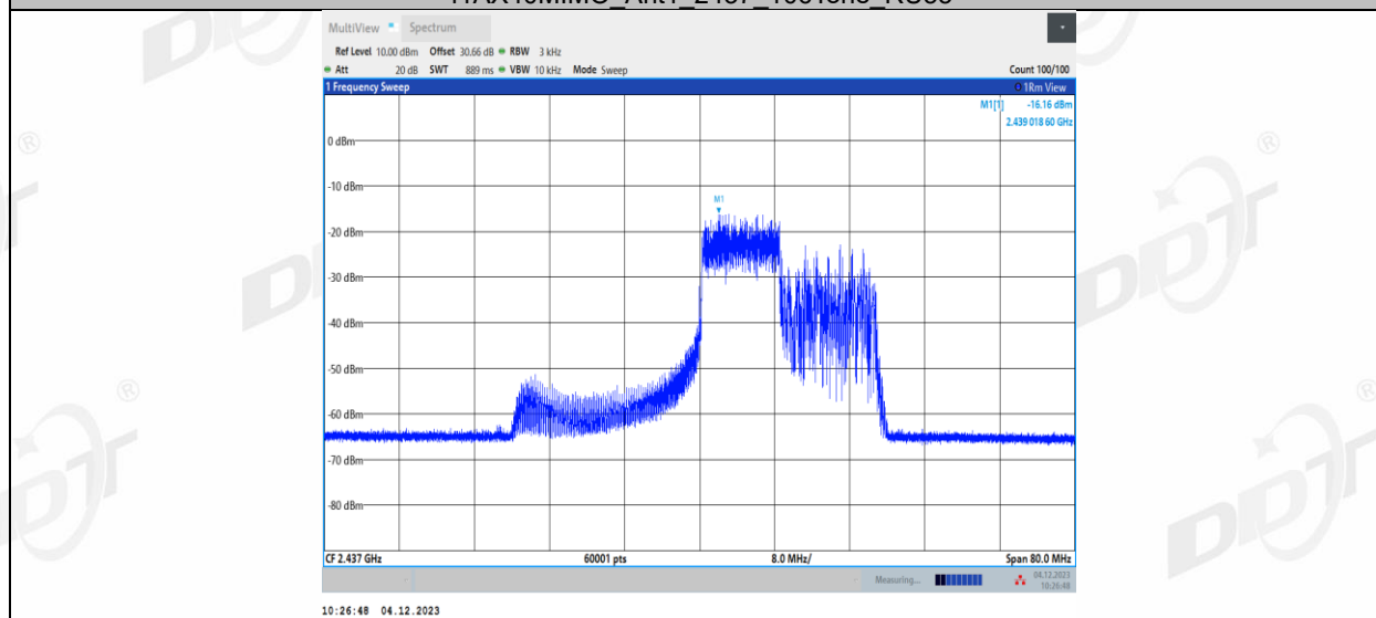
11AX40MIMO_Ant1_2437_106Tone_RU56
