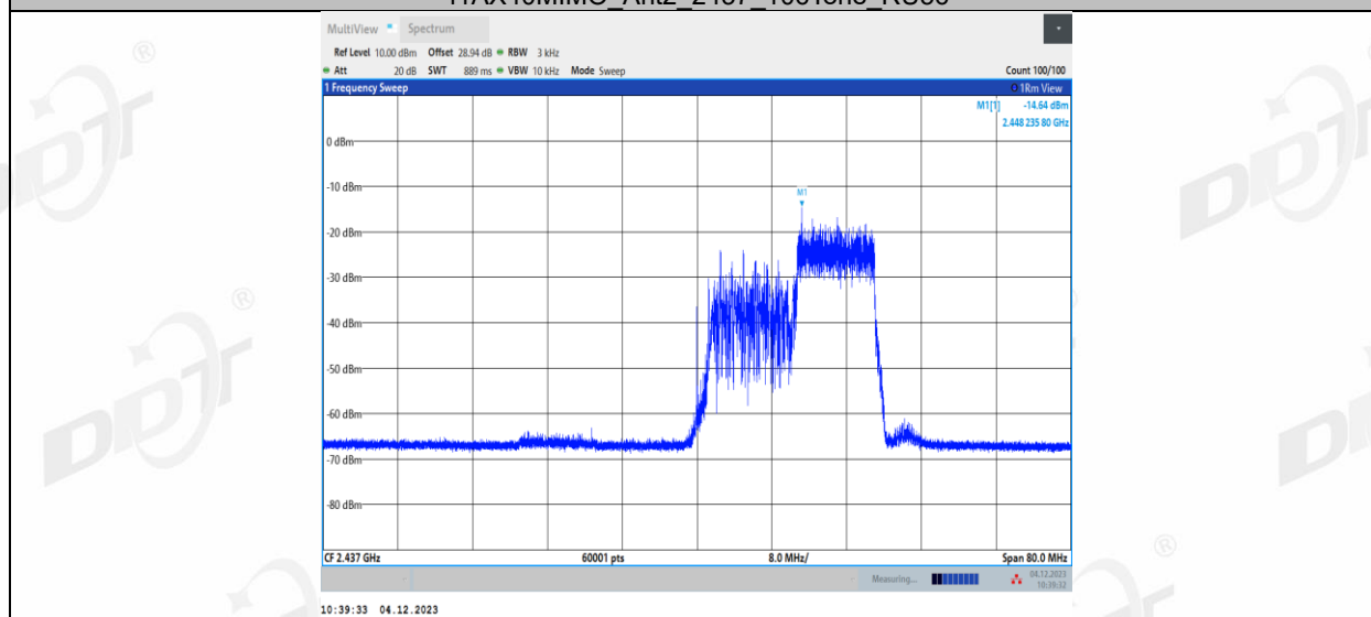
11AX40MIMO_Ant2_2437_242Tone_RU61
