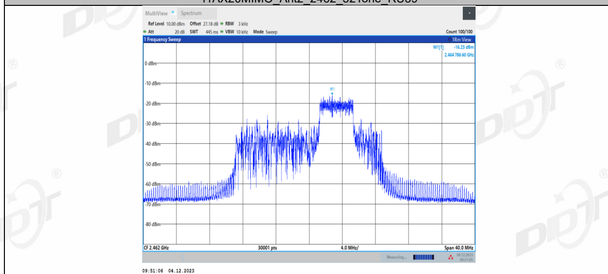
11AX20MIMO_Ant2_2462_52Tone_RU40
