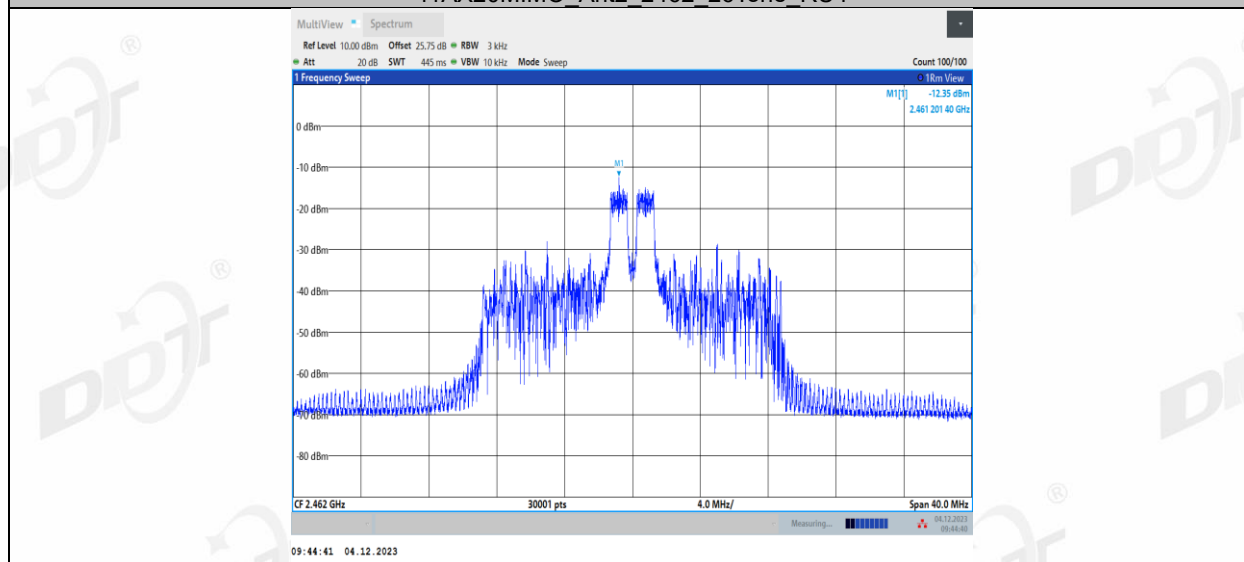
11AX20MIMO_Ant2_2462_26Tone_RU8
