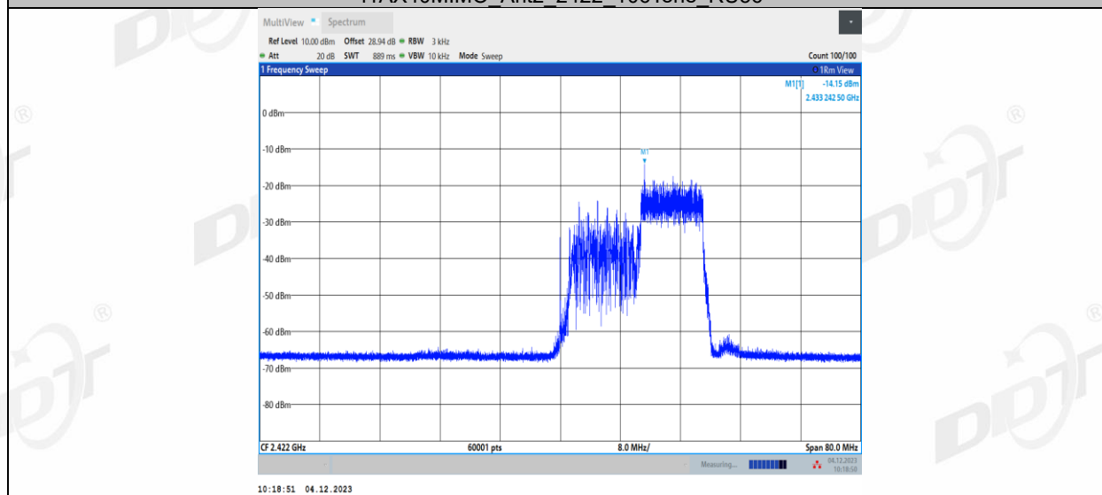
11AX40MIMO_Ant2_2422_242Tone_RU61
