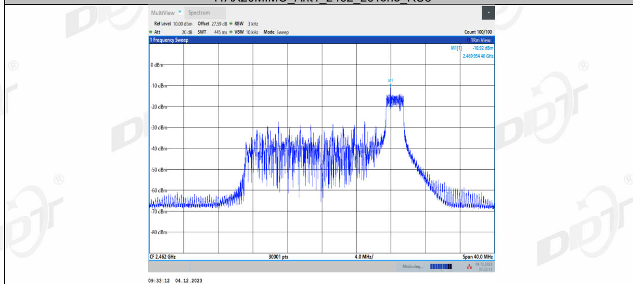
11AX20MIMO_Ant1_2462_52Tone_RU37
