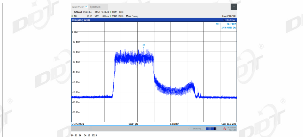
11AX40MIMO_Ant2_2422_242Tone_RU62
