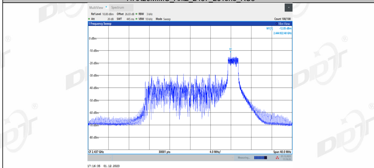
11AX20MIMO_Ant2_2437_52Tone_RU37
