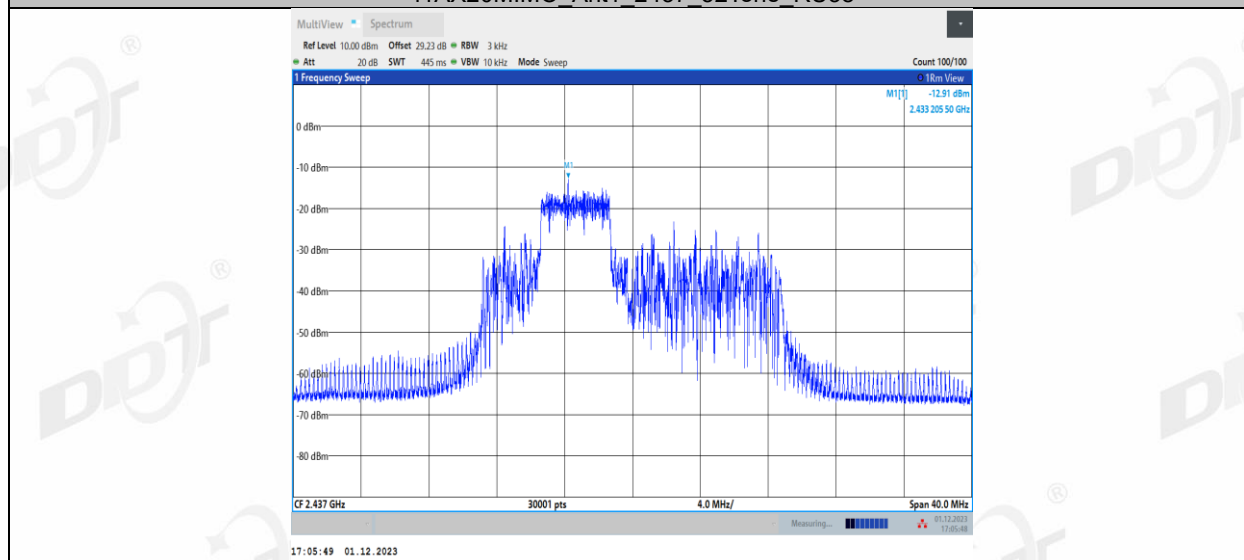
11AX20MIMO_Ant1_2437_52Tone_RU39
