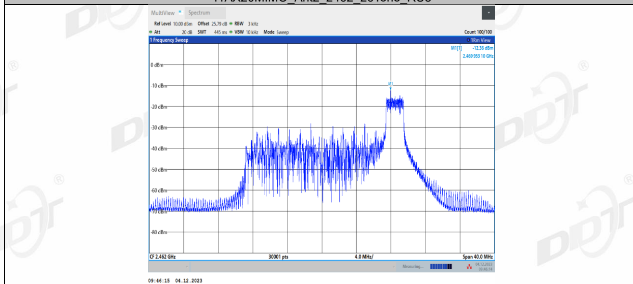
11AX20MIMO_Ant2_2462_52Tone_RU37
