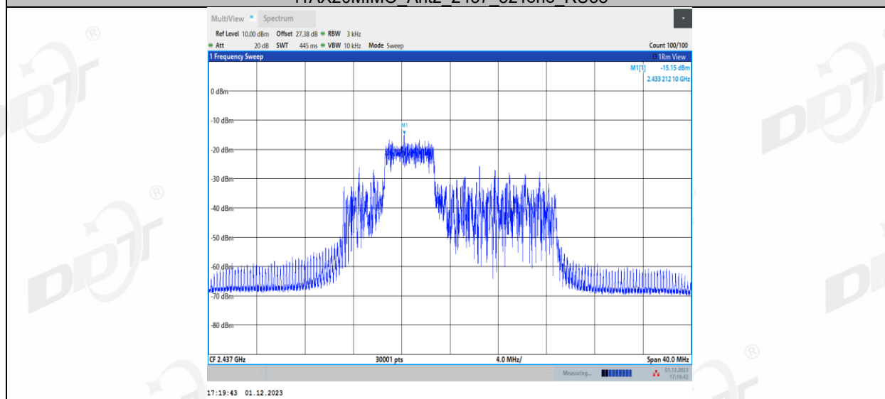
11AX20MIMO_Ant2_2437_52Tone_RU39
