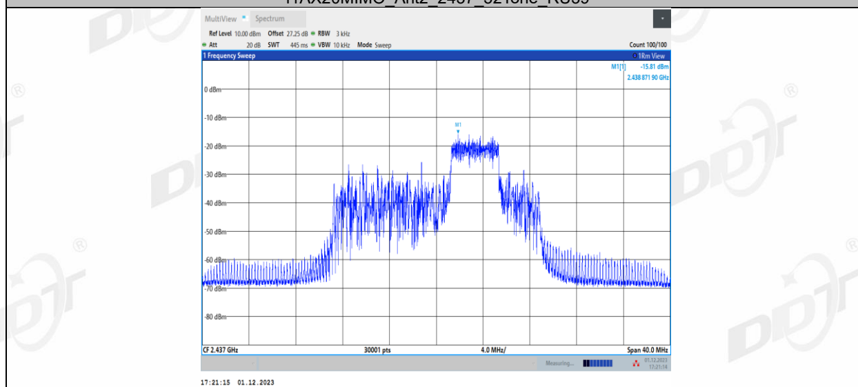
11AX20MIMO_Ant2_2437_52Tone_RU40
