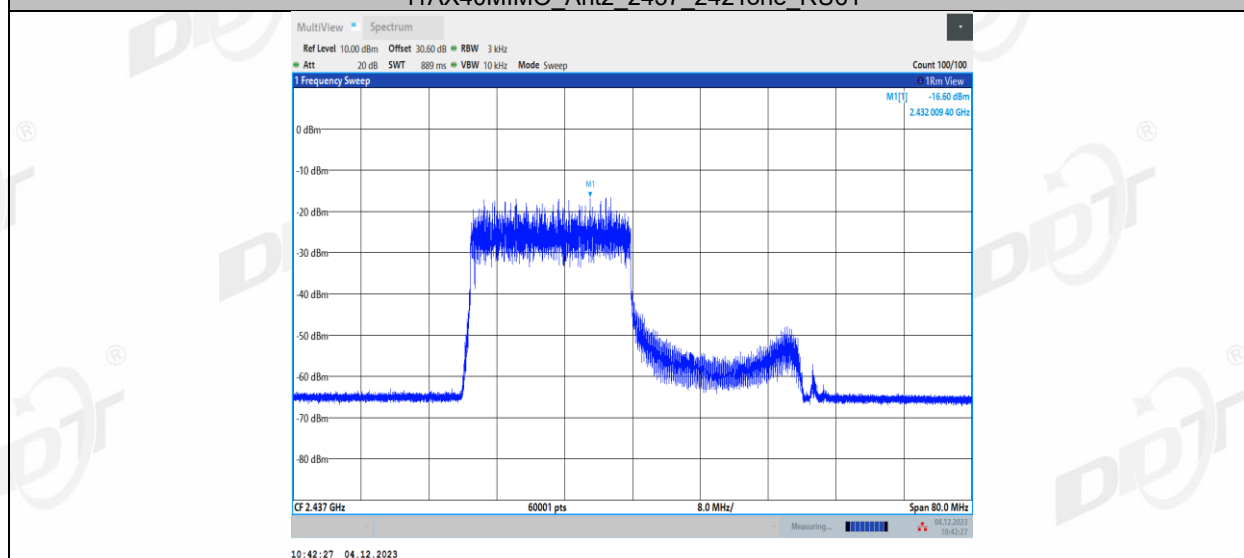
11AX40MIMO_Ant2_2437_242Tone_RU62
