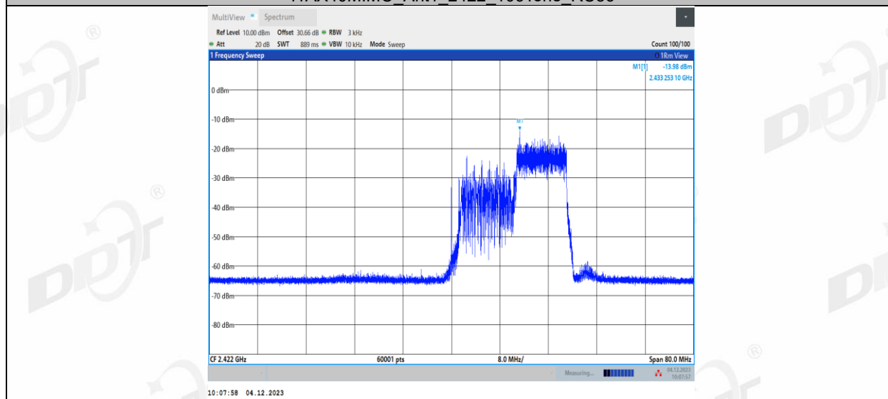
11AX40MIMO_Ant1_2422_242Tone_RU61
