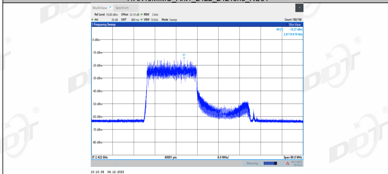
11AX40MIMO_Ant1_2422_242Tone_RU62
