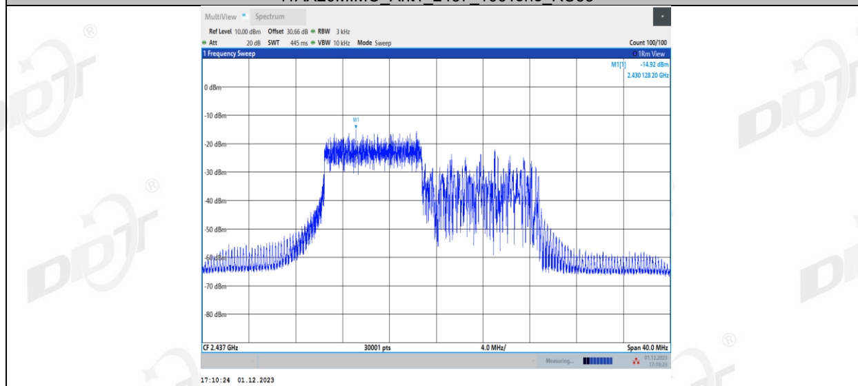
11AX20MIMO_Ant1_2437_106Tone_RU54
