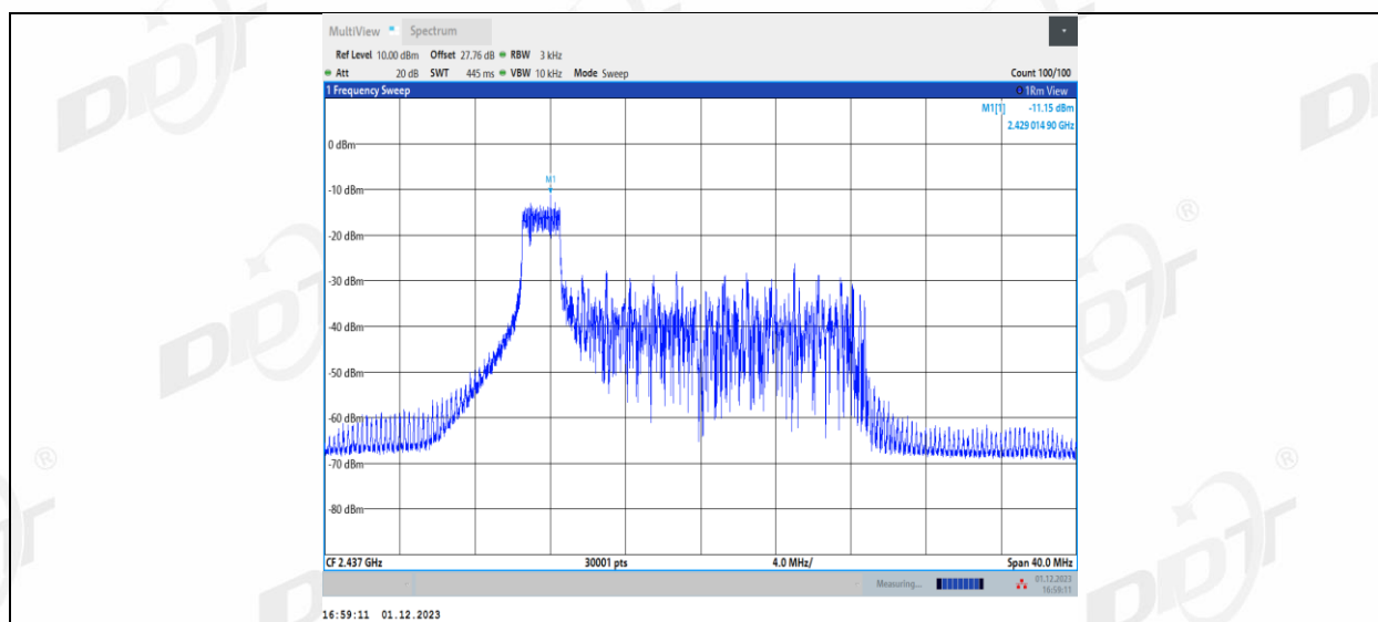
11AX20MIMO_Ant1_2437_26Tone_RU4
