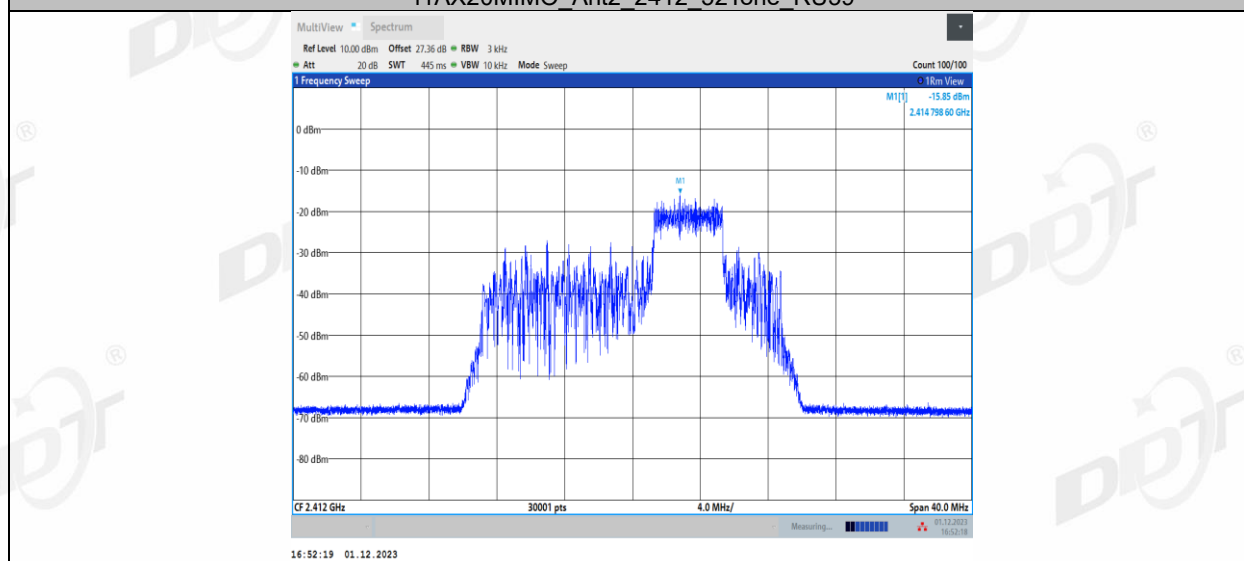
11AX20MIMO_Ant2_2412_52Tone_RU40
