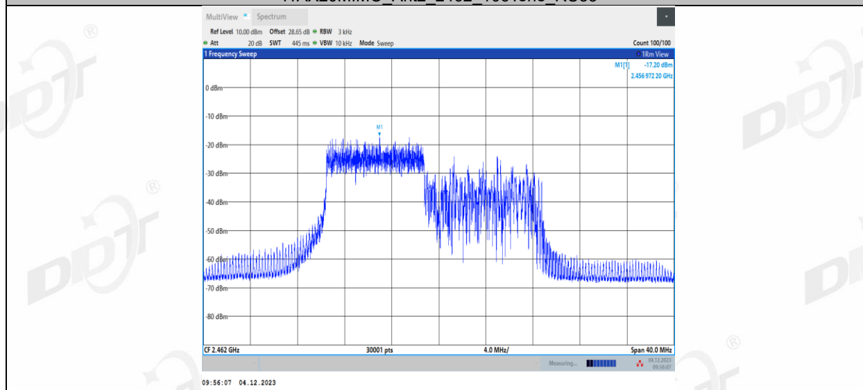
11AX20MIMO_Ant2_2462_106Tone_RU54
