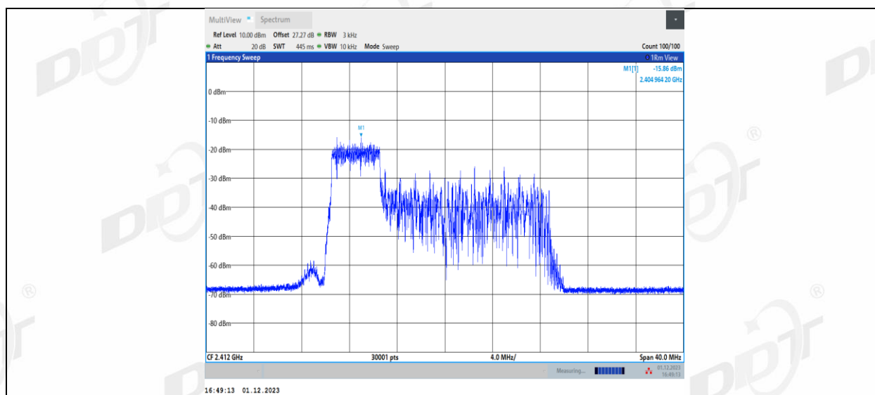
11AX20MIMO_Ant2_2412_52Tone_RU38
