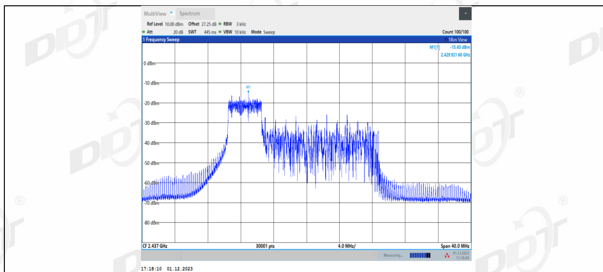
11AX20MIMO_Ant2_2437_52Tone_RU38
