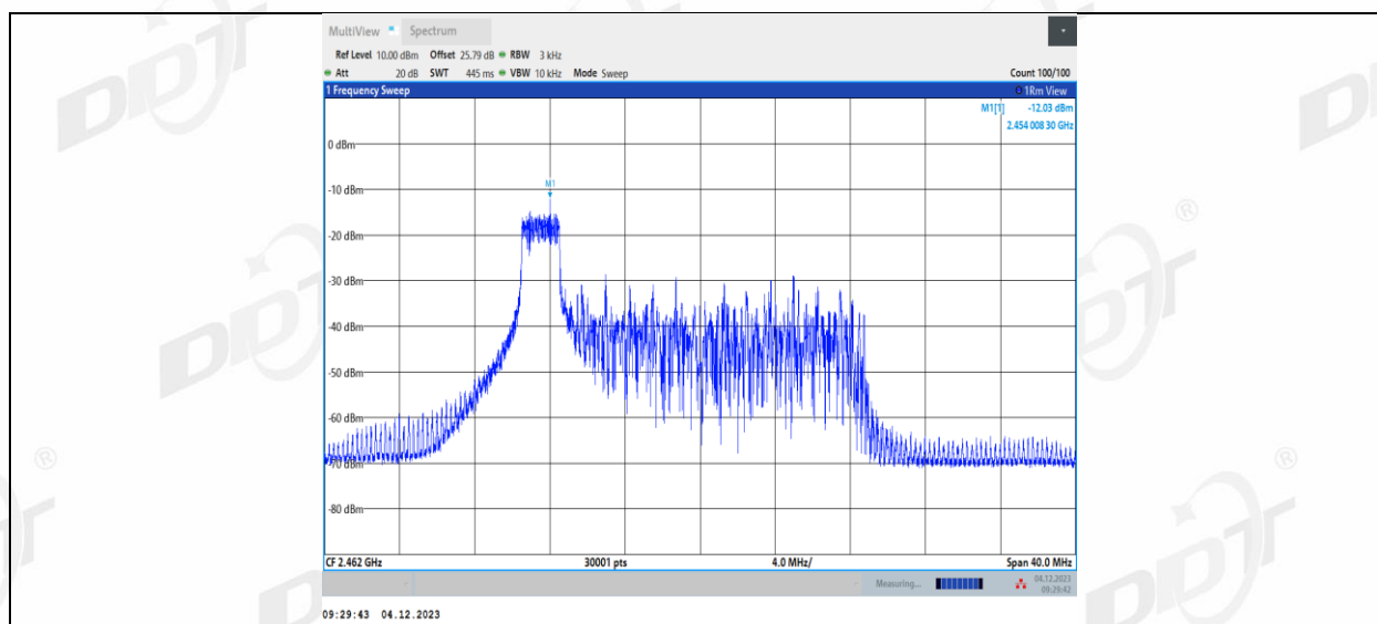
11AX20MIMO_Ant2_2462_26Tone_RU4
